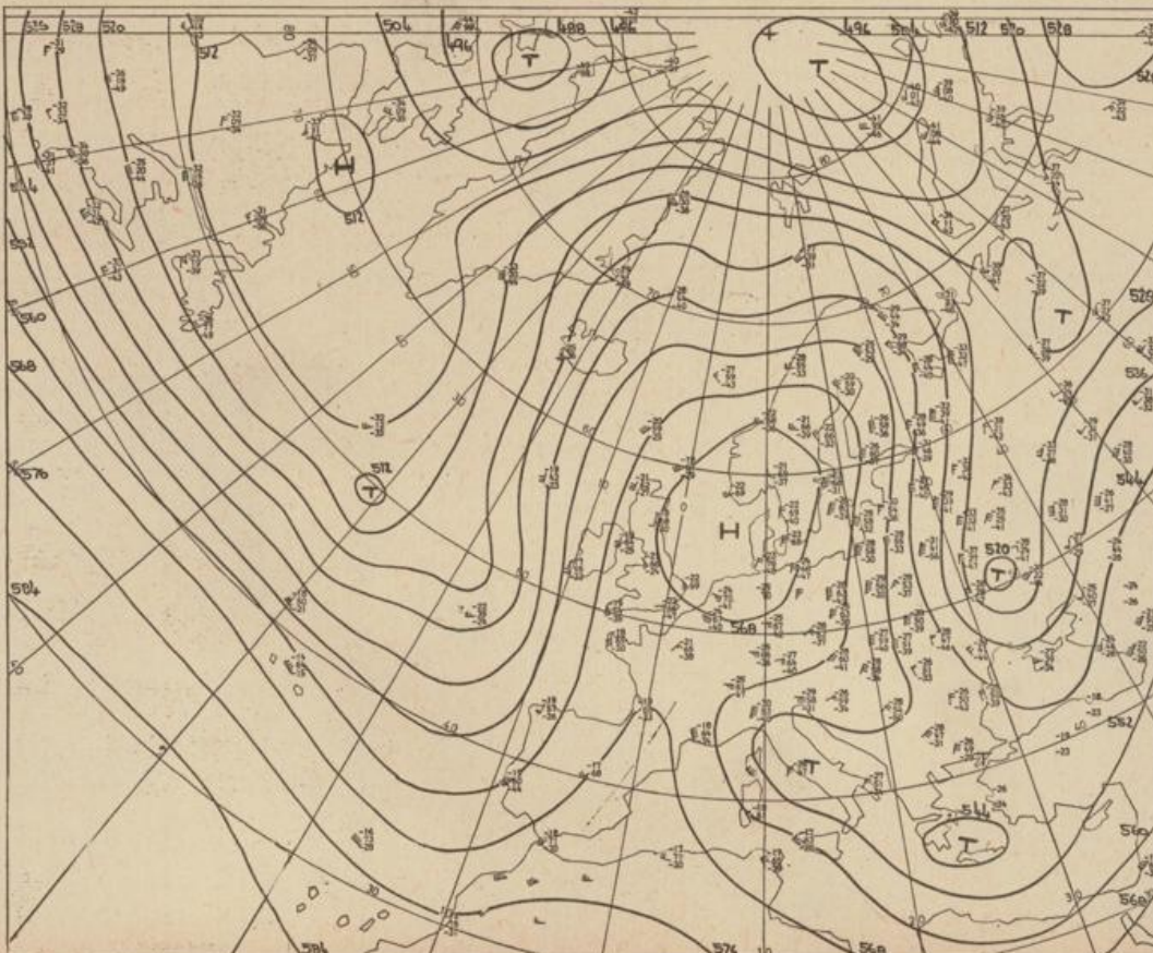
Höhenwetterkarte (Absolute Topographie 500 mb entsprechend ca. 5500 m Höhe) vom 04.12. 01 Uhr
