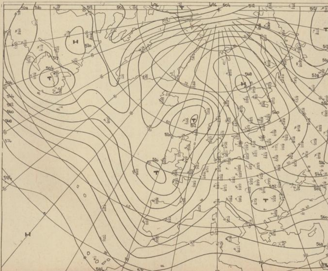
Höhenwetterkarte (Absolute Topographie 500 mb entsprechend ca. 5500 m Höhe) vom 08.12. 01 Uhr
