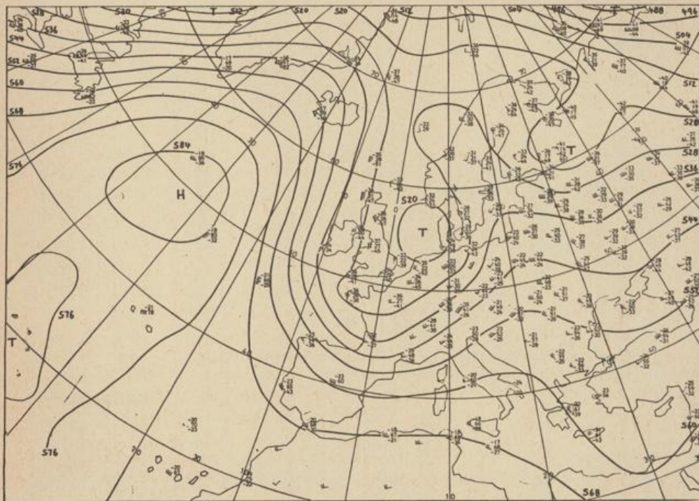
Höhenwetterkarte (Absolute Topographie 500 mb entsprechend ca. 5500 m Höhe) vom 28.12. 01 Uhr
