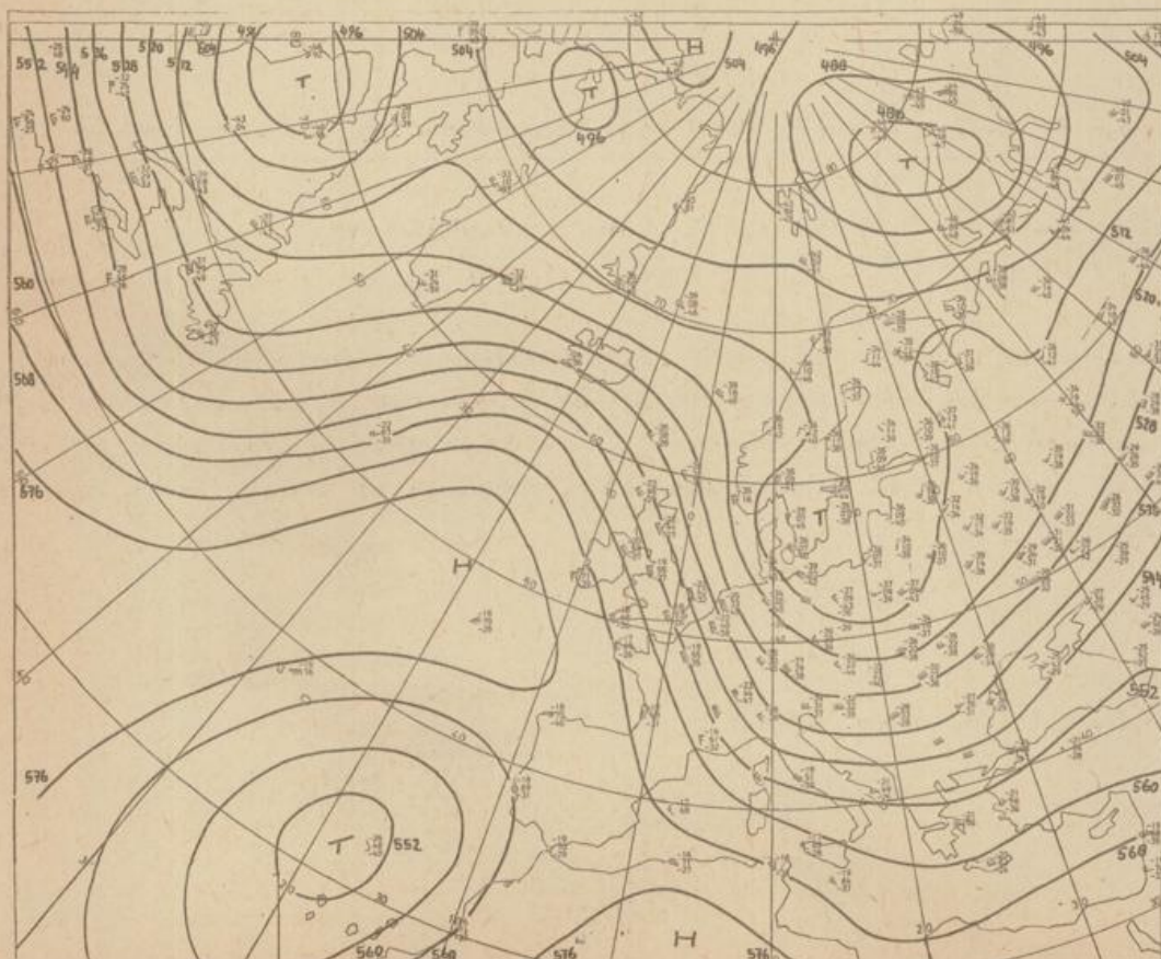
Höhenwetterkarte (Absolute Topographie 500 mb entsprechend ca. 5500 m Höhe) vom 01.01. 01 Uhr
