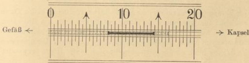
Abb. 10. Mittelstück des Minimumthermometers.
