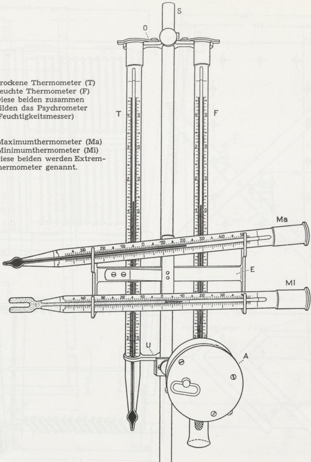
Abb. 3: Anordnung der Thermometer
