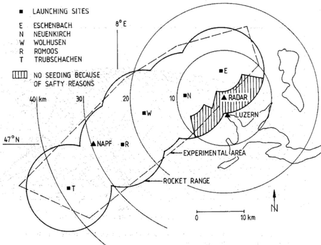
Bild 3: Das Testgebiet vom Großversuch IV mit den 5 Standorten der Raketenwerfer. Ebenfalls eingezeichnet sind die Wirkungskreise der Raketen.
