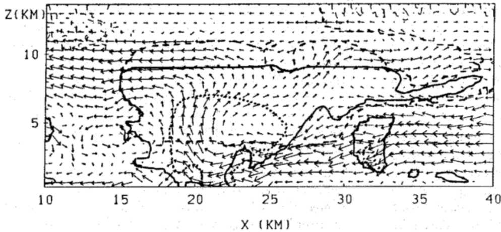
Bild 1: Windvektoren und Isolinien des Mischungsverhältnisses von Wolkenwasser (ausgezogen), Regenwasser (punktiert) und Eis (gestrichelt) kurz nach dem Zeitpunkt, an dem der Niederschlag den Erdboden erreicht hat (52 Min. Simulationszeit). Die Isolinien sind so gewählt, daß sie den Umriß der Wolke wiedergeben. Die Wolke bewegt sich mit der mittleren Strömung von rechts nach links.
