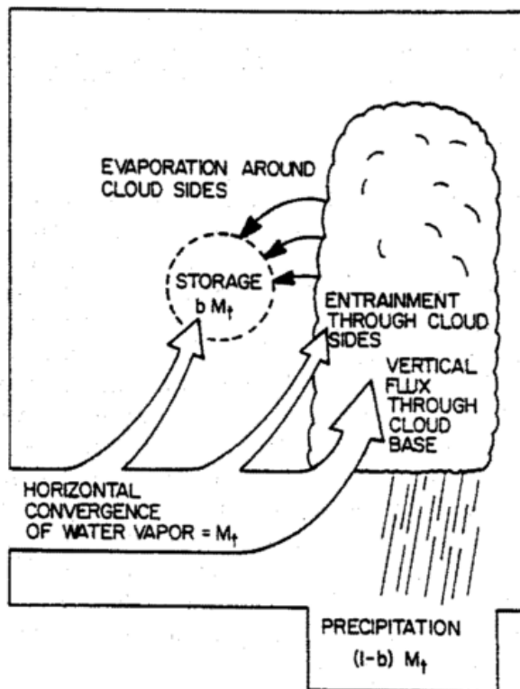
Bild 4: Schematische Darstellung zum Feuchtezyklus in einer Gittersäule mit Konvektion (nach ANTHES 1977).
