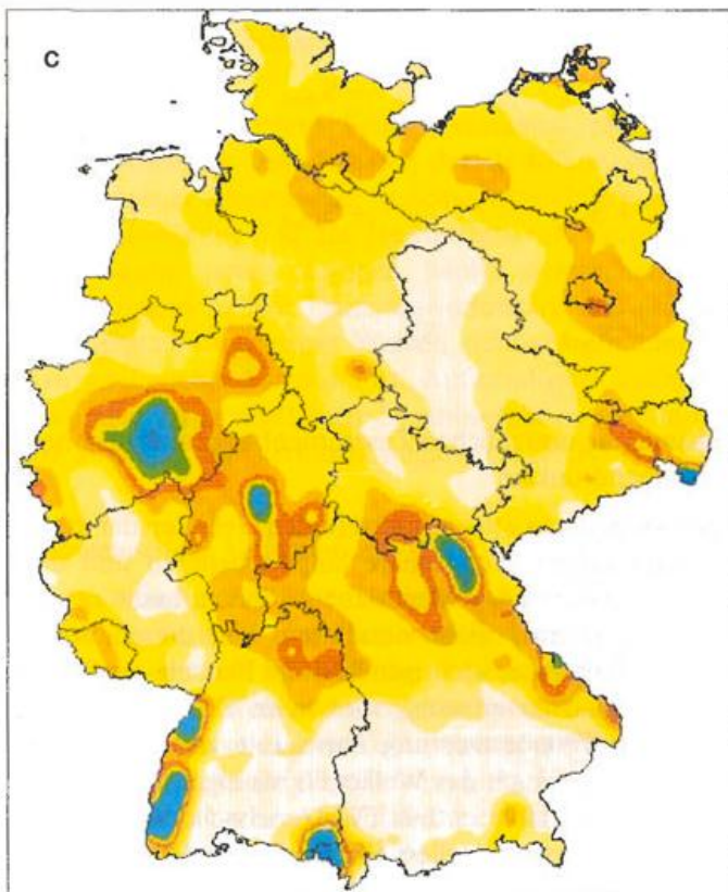
Bild 2: Räumliche Verteilung der 24-stündigen Niederschlags-summe vom 15.2.92 6 UTC bis 16.2.92 6 UTC für das Gebiet der Bundesrepublik Deutschland (Einheit 0.1 mm). a) Beobachtungen (Klimameßnetz, ca. 4500 Stationen) b) Vorhersage mit dem Europa-Modell c) Vorhersage mit dem Deutschland-Modell
