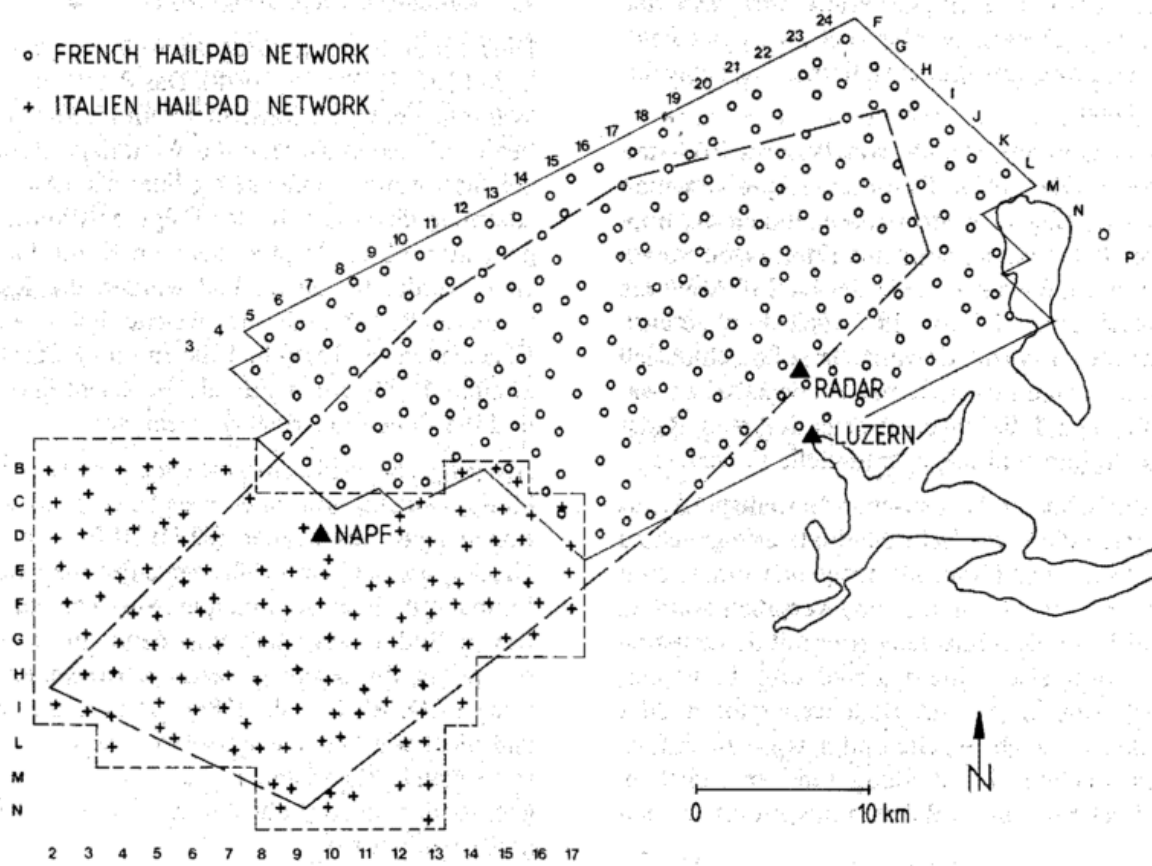
Bild 1: Das Testgebiet vom Großversuch IV in der Zentralschweiz. Die Kreuze, bzw. die Kreise bezeichnen Standorte, wo ein Hageldetektor mit einer Auffangfläche von 0,1 m 2 aufgestellt war. „Napf“ bezeichnet den im Testgebiet liegenden dominierenden Berg (1408 m ü. M.), an dem sich sehr viele Cumulonimben bilden.
