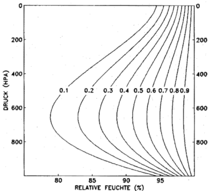
Bild 1: Parametrisierung des Bedeckungsgrades als Funktion von Druck und relativer Feuchte im Europa-Modell des DWD.
