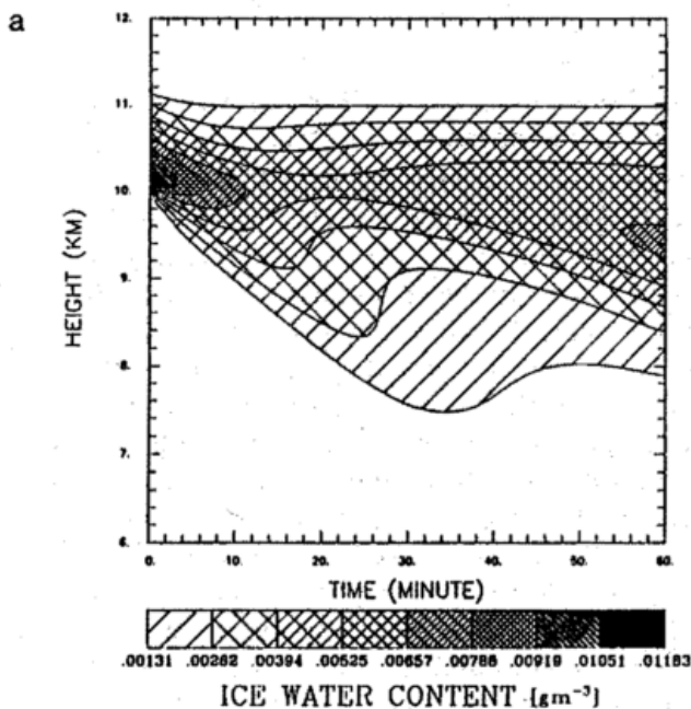
Bild 3: Entwicklung der Vertikalverteilung des Eiswassergehaltes für vorgegebene Vertikalgeschwindigkeiten a) w = 5 cm/s und b) w = 0 .
