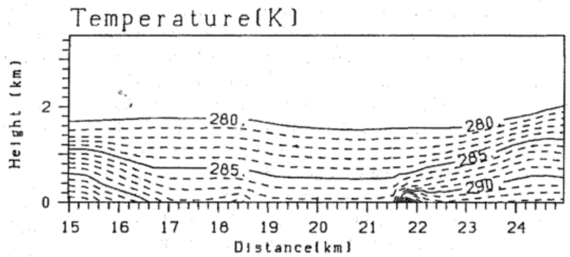
Bild 2: Isothermen im Abstand 1 K zum gleichen Zeitpunkt wie in Bild 1. Der Ausschnitt unterhalb der Wolke ist hier vergrößert dargestellt.
