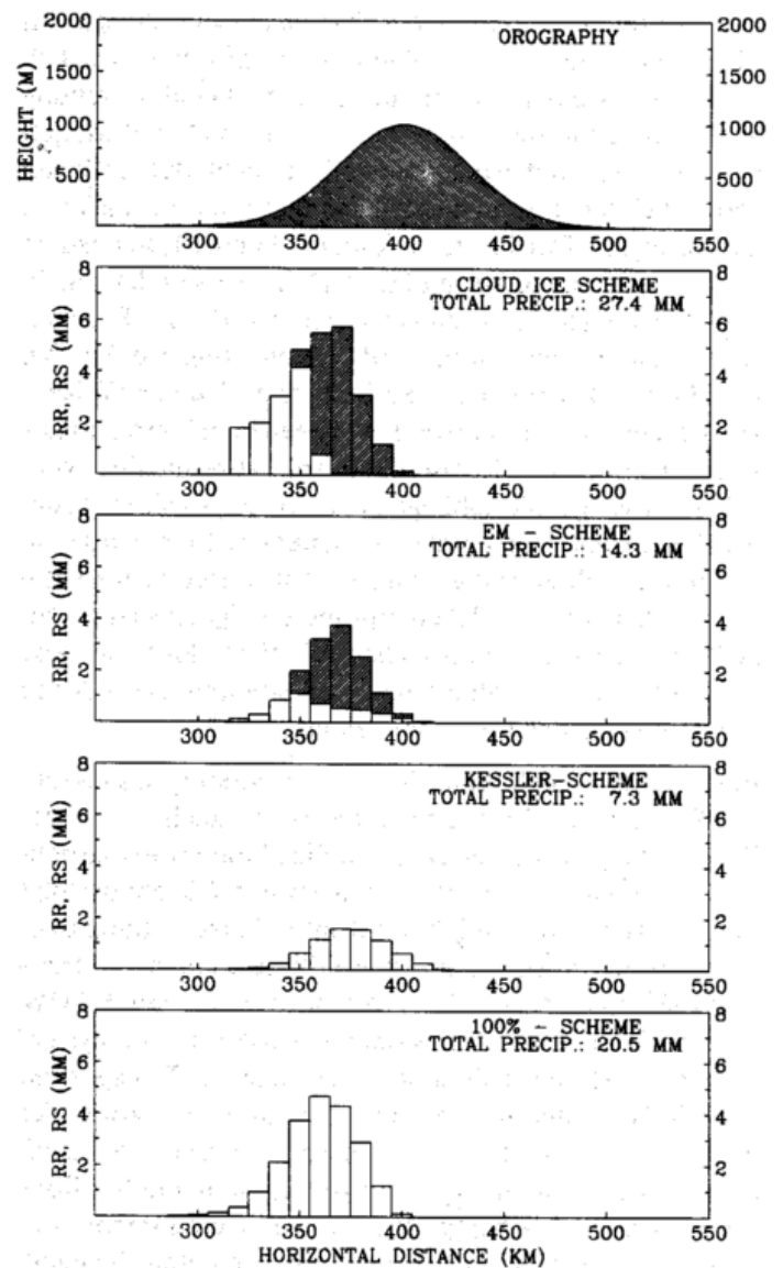
Bild 3: Verteilung der 6-stündigen Niederschlagsmenge von Regen (RR) und Schnee (RS, schraffiert) für die Simulation einer zweidimensionalen Gebirgsüberströmung mit dem Wolkeneisschema, der EM-Parametrisierung, dem Kessler-Verfahren und dem 100%-Schema (Maschenweite 10 km; Anfangsbedingungen: 10 m/s Anströmgeschwindigkeit, 5°C in 1000 hPa bei 6.5 K/km Temperaturgradient, 90% relative Feuchte in der mittleren Troposphäre).
