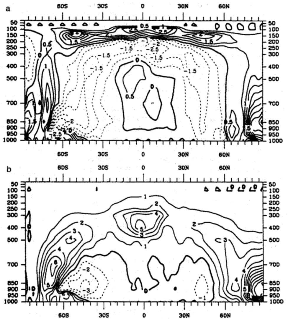
Bild 3: Änderung der zonal gemittelten Wolkenbedeckung (a) und des Wolkenwassergehalts (b) als Funktion der Höhe (Druck in hPa) und der geographischen Breite, simuliert mit dem ECHAM-Modell. Die Differenzen beziehen sich auf 10-jährige Mittel zwischen den Werten für eine um 2,5 K erhöhte Meeresoberflächentemperatur und heutigen Werten (J. PERLWITZ, persönliche Mitteilung). Einheiten: (a) Prozent für Bedeckungsgrad und (b) 10^{-3} g/kg für das Wolkenwassermischungsverhältnis.
