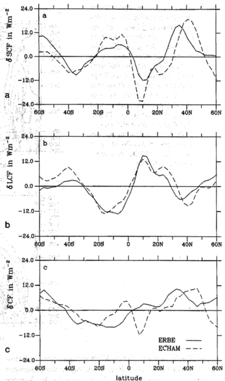
Bild 4: Abweichung des zonal gemittelten "Cloud Forcing" gegenüber dem Jahresmittel 1985 als Funktion der geographischen Breite, simuliert mit dem ECHAM-Modell (gestrichelt) und analysiert aufgrund von ERBE-Messungen (ausgezogen), jeweils für den Monat Juli 1985. Positive Werte bedeuten eine Erwärmung durch Wolkenveränderungen relativ zum Jahresmittel, negative eine Abkühlung. a) Solarer Spektralbereich b) Terrestrischer Spektralbereich c) Nettoeffekt
