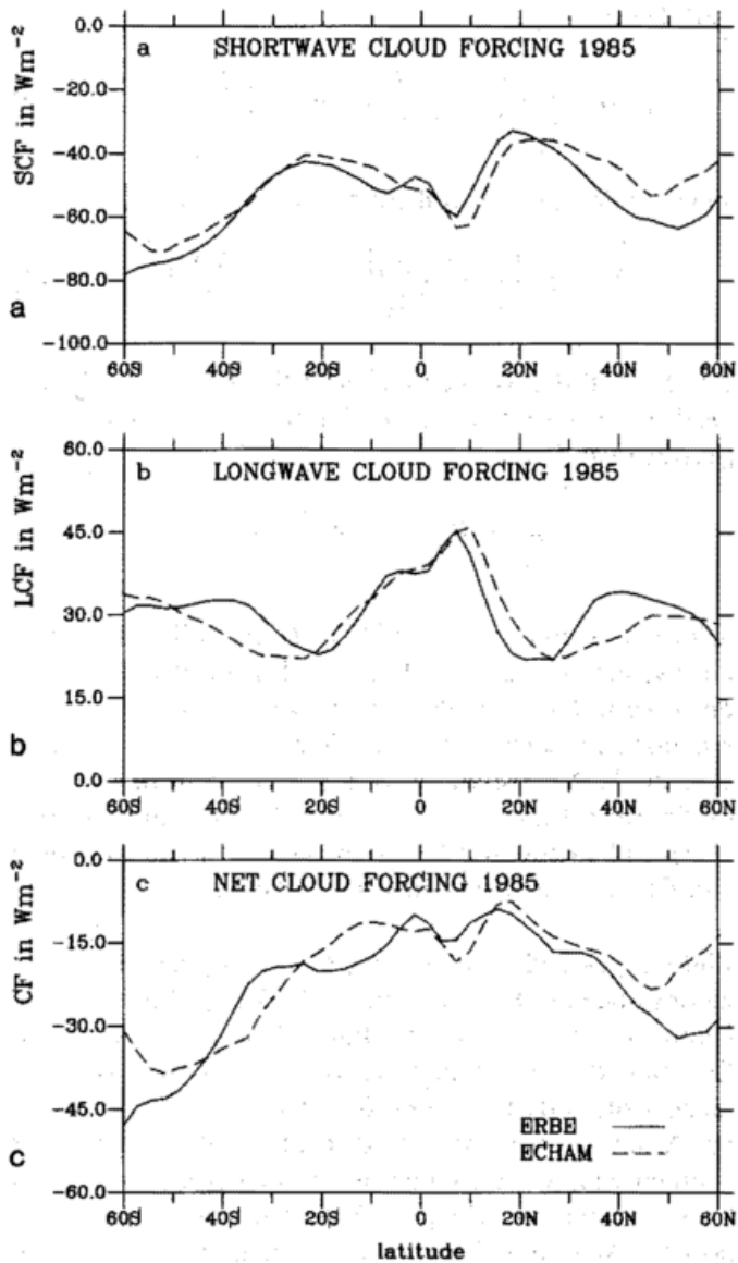
Bild 1: Vergleich von simuliertem und beobachtetem zonal gemitteltem „Cloud Forcing“ als Funktion der geographischen Breite für das Jahr 1985. Positive Werte bedeuten eine Erwärmung des Klimasystems durch Wolken, negative eine Abkühlung. a) Solarer Spektralbereich b) Terrestrischer Spektralbereich c) Nettoeffekt
