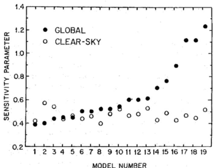
Bild 2: Klimasensitivitätsparameter \lambda bzw. \lambda_0 (K pro \text{W/m}^2 Strahlungsbilanzänderung) jeweils für die wolkenfreie Atmosphäre (offene Kreise) und für die bewölkte Atmosphäre (ausgefüllte Kreise), simuliert von 19 atmosphärischen Zirkulationsmodellen (CESS et al. 1990).
