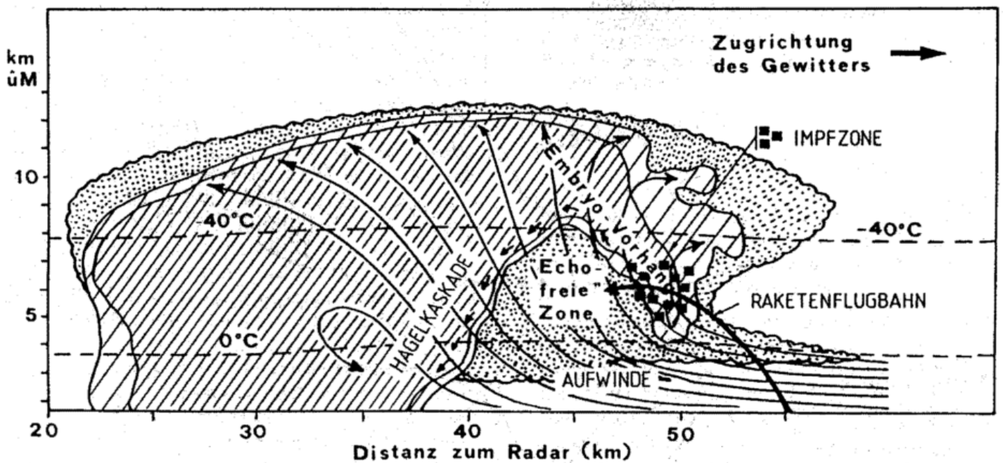
Bild 2: Das konzeptionelle Hagelzellenmodell, wie es im Großversuch IV benützt wurde. In der Impfzone befinden sich die zu vereisenden unterkühlten großen Regentropfen.
