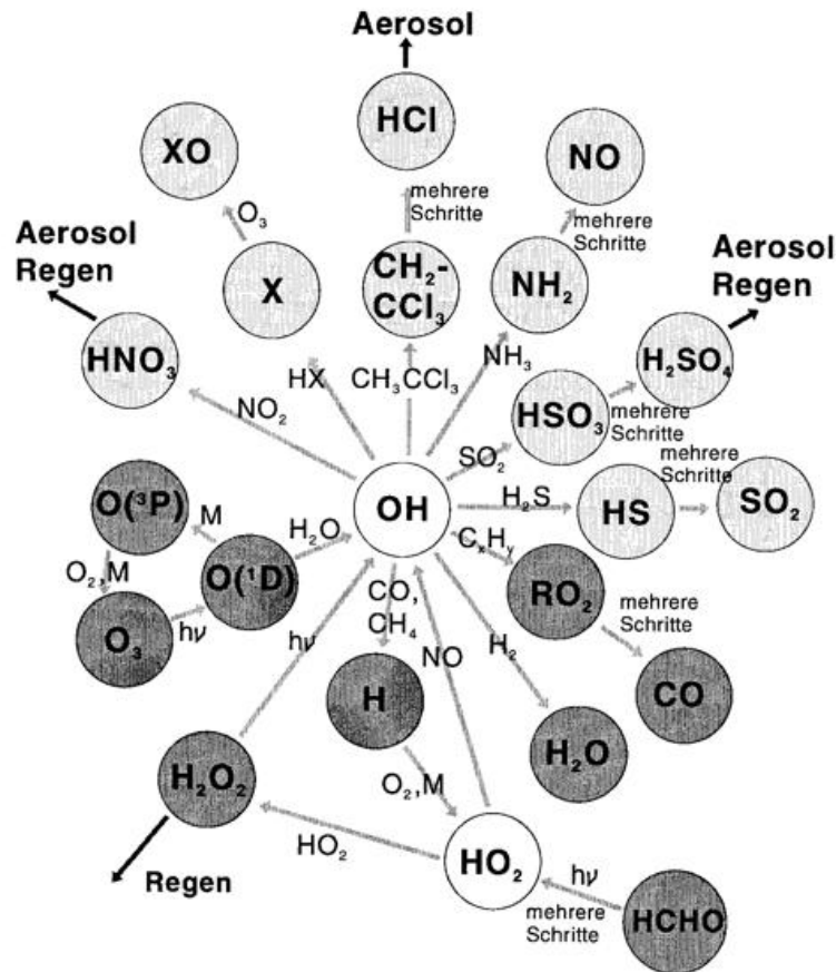
Bild 3: Die Photochemie des OH-Radikals und ihre Bedeutung für atmosphärische Spurenstoffe. Die dunkel dargestellten Verbindungen (einschließlich HO 2 ) kontrollieren die OH-Konzentration; bei den hell angeordneten Verbindungen bestimmt die Reaktion mit OH die Konzentrationen der jeweiligen Reaktanden und Produkte. Die Pfeile geben die Hauptreaktionswege zwischen den in den Kreisen dargestellten Verbindungen an. Entsprechende Beschriftungen symbolisieren die dabei beteiligten Photonen (hν) oder Reaktanden. Elementare Zwischenreaktionen sind aus Übersichtsgründen nicht aufgeführt. Es bedeuten: HX = HCl, HBr, HI oder HF, C x H y = Kohlenwasserstoffe (nach CHAMEIDES und DAVIS 1982).
