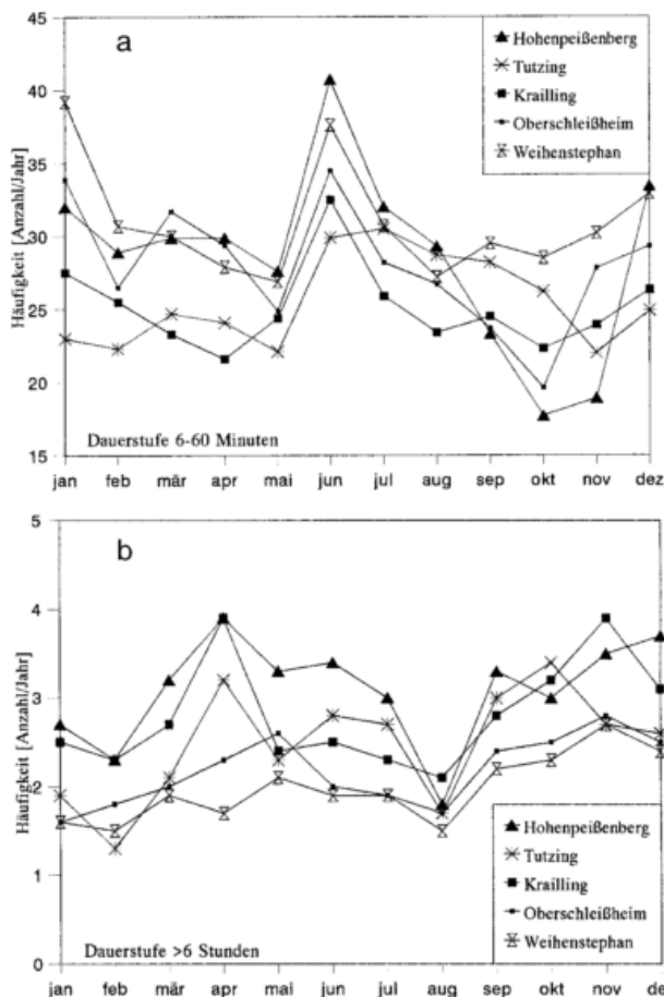
Bild 4: Jahrgang der mittleren Häufigkeit der Andauer von meßbaren Niederschlagsereignissen an fünf Ombrometer-Standorten in den Jahren 1980 – 1994; a) Ereignisdauer von 6 – 60 Minuten, b) Ereignisdauer > 6 Stunden.
