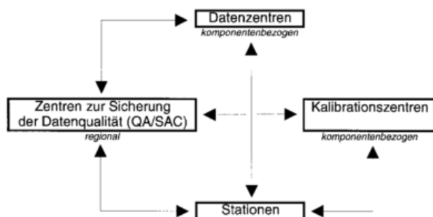
Bild 1: Aufbau des GAW-Programms
