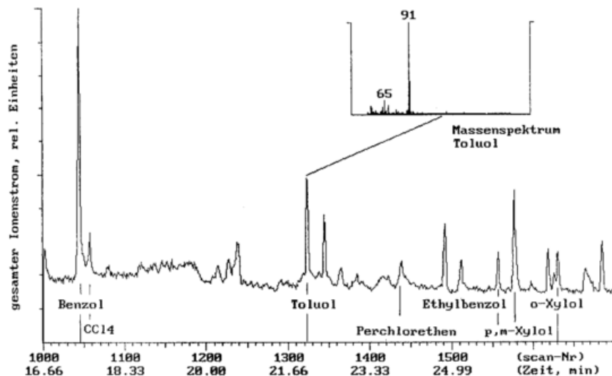
Bild 1: Ausschnitt aus einem Ionenchromatogramm anthropogener Kohlenwasserstoffe (BTEX und halogenierte Verbindungen) in einer Außenluftprobe. Eingebildet ist das Massenspektrum von Toluol. Mit GC/MS werden hauptsächlich höhermolekulare, schwerflüchtige Verbindungen erfaßt.
