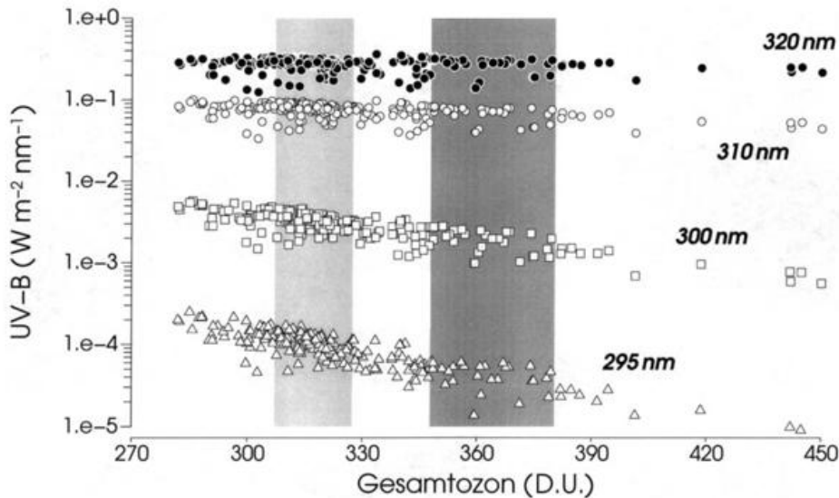
Bild 7: UV-B verschiedener Wellenlängen bei einer Sonnenhöhe von 55^\circ \pm 2^\circ in Abhängigkeit vom Gesamtozon. Der dunkelgraue Bereich (■) gibt die langfristige mittlere Schwankungsbreite des Gesamtozons im Mai an, entsprechend der hellgraue Bereich (□) für August.
