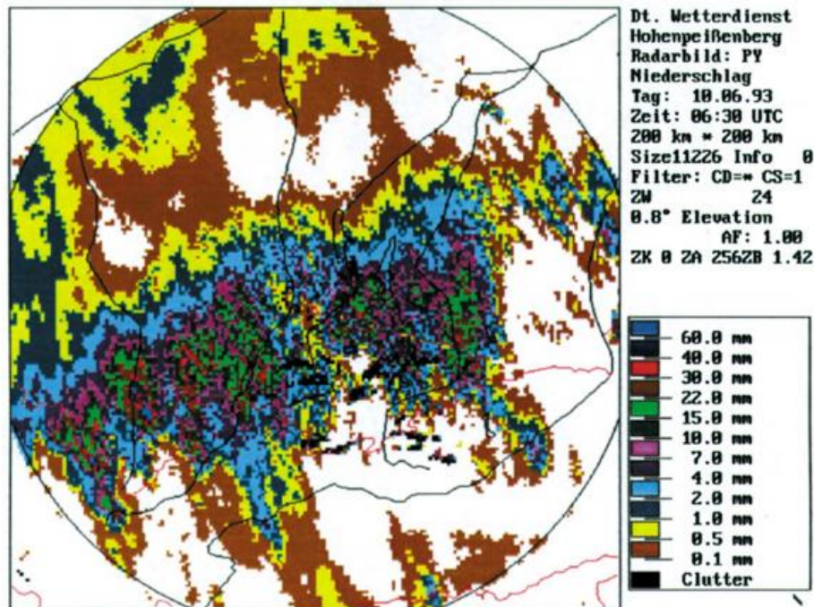
Bild 1: Beispiel einer 24h-Aufsummierung der im 5-min-Zeitrastr gemessenen Niederschlagsverteilung (unangeeicht), MOHp, 9.-10.6.93, 06:30 UTC, 100 km Radarumgebung. Stark gegliederte Niederschlagsfelder einer nach NE gezogenen konvektiven Multizelle mit Regenmaxima >40 mm (und Hagelzone, dunkelblau) im Raum Sonthofen, Iller (ca. 240°, 60 km). Die Repräsentanz eines 1km 2 -Meßwertes wird hier stark von der Niederschlagsstruktur bestimmt. (Radar im Bildzentrum (x), dort Niederschlagsminimum).
