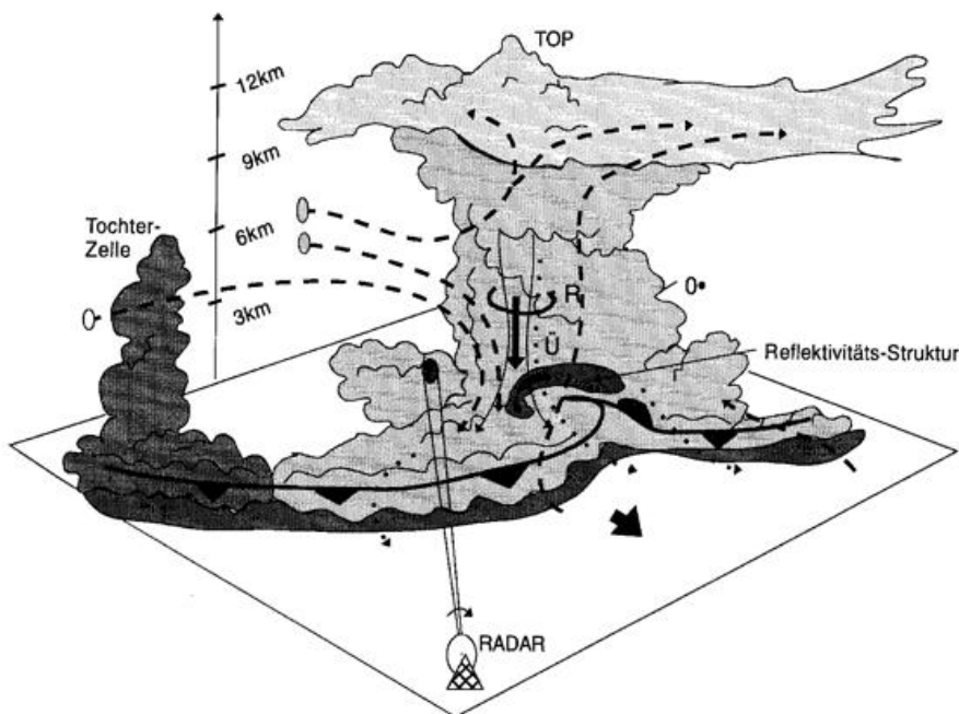
Bild 1: Schemazeichnung einer Multi-Zelle mit Boden-Reflektivitätsstruktur und Strömungsmerkmalen (gestrichelt, punktiert) aus der Sicht eines abtastenden Niederschlagsradars. Toplage, Downdraft (vertikaler Pfeil), zyklonale interne Zellrotation (R) und möglicher Echoüberhang (Ü, Schwachechozone), können als Indizien zur Kennzeichnung des jeweiligen Zell-Entwicklungsstadiums beitragen.
