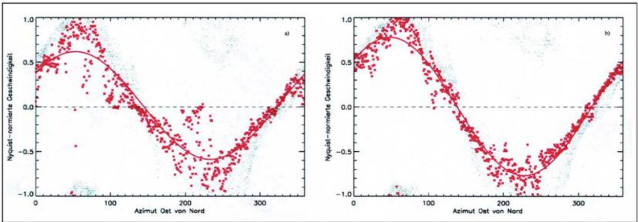
Bild 5: VAD- Darstellung der Radialgeschwindigkeit a) eines ungefilterten und b) eines gefilterten Umlaufs für 3 und 4 km Schrägenentfernung (fett). Die Abweichungen von der Sinusform in a) sind auf Clutterbeiträge (Geschw. = 0) zurückzuführen, welche in b) gedämpft wurden. Eingezeichnet sind auch die Grundschwingung der Fourierzerlegung (Linie) sowie (Punktsymbole) höhere Windgeschwindigkeiten im Entfernungsbereich 10 bis 20 km, die zu einer Faltung führen. Radar Neuhaus, 12.03.96 14:40 und 14:45, Elevation = 1°, PRF = 600 Hz, V_{\max} = 8 m/s.
