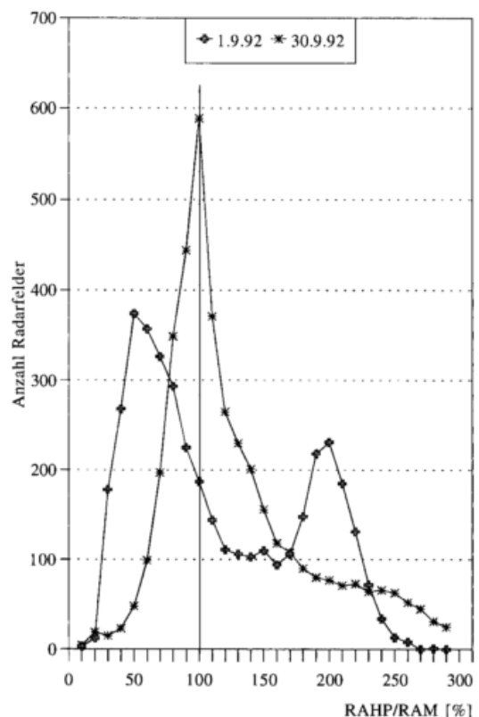
Bild 7: Vergleich zur Übereinstimmung der jeweiligen Niederschlagshöhen der Radar-messungen Hohenpeißenberg (HP) und München (M), Sept. 1992, analog Bild 6. Häufigkeit der Radarfelder mit entsprechenden Quotienten RAHP/RAM.
