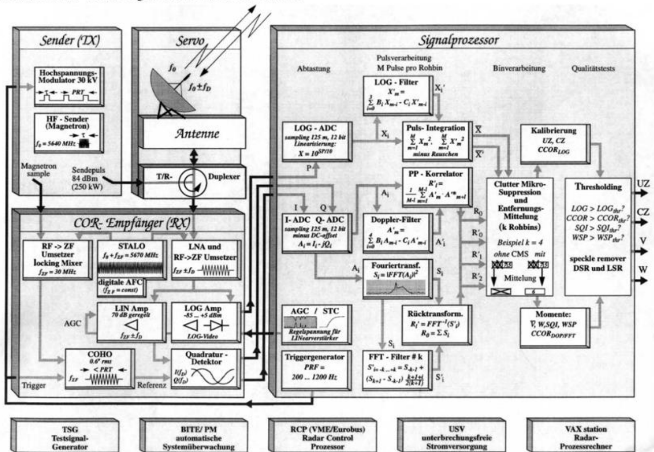
Bild 1: Radar MOHp Prinzipschaltbild. Links die eigentliche Radar-Hardware mit Sender, Servo, Antenne und Empfänger, rechts der Signalprozessor mit den einzelnen Verarbeitungsstufen inklusive einiger (im Text weitgehend vermiedener) Gleichungen. Unten symbolisch einige z.T. periphere Geräte.
