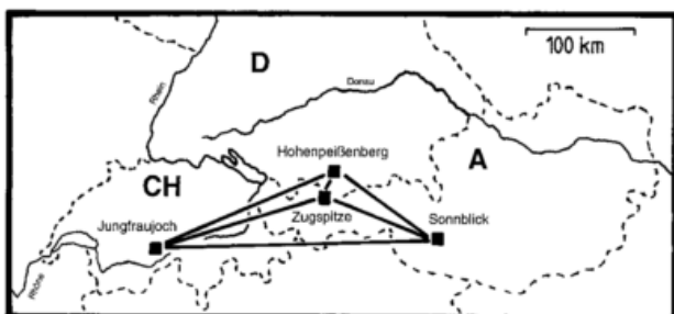
Bild 5: Am GAW-DACH-Verband beteiligte Stationen
