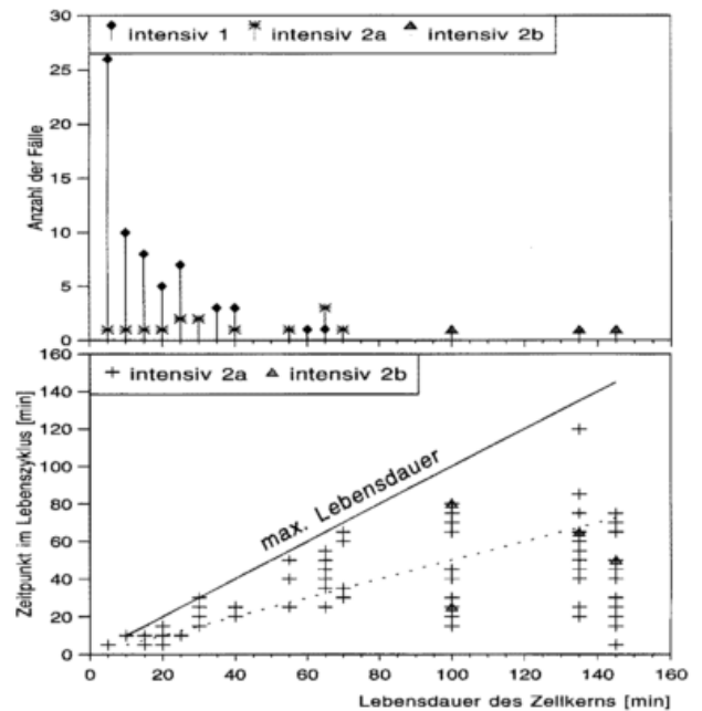
Bild 6: Versuch einer Klassifizierung von Einzelzellen bzgl. Andauer, maximal erreichtem Stadium und Zeitabschnitt ihrer jeweiligen Entwicklungshöhepunkte, Radar Hohenpeißenberg, 100 km Umkreis, 29. 6. 94, 11:30-17:50 UTC
