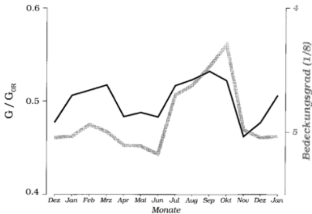
Bild 3: Mittlere Jahresgänge der normierten Globalstrahlung G/G_{0R} (schwarze Linie) und des Bedeckungsgrades (graue Linie) für den Zeitraum 1953 bis 1995. Der Bedeckungsgrad ist invers aufgetragen. Der Korrelationskoeffizient für den Zusammenhang der mittleren Jahresgänge beträgt -0,75 und ist auf dem 2\sigma -Niveau signifikant.
