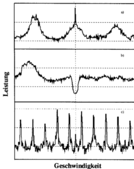
Bild 2: Gemessene Dopplerspektren, Abszisse von -V_{\max} bis +V_{\max} , Ordinatenanteile 20 dB. Oben: Clutterpeak bei V=0 , Regen- (links) mit Spiegelspektrum (rechts) infolge Fehlableichs. Mitte: Gleiche Situation nach I/Q-Abgleich, Clutterpeak beseitigt durch Dopplerfilter #2. Unten: Spektrum ohne Niederschlagsecho mit Artefakten. Der im DWD bisher eingesetzte Puls-Paar-Algorithmus kann Spiegelspektren oder Artefakte nicht erkennen.
