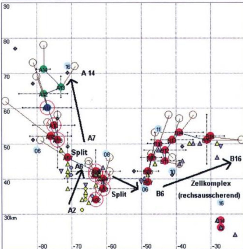
Bild 3: Gegenüberstellung von zeitlich überlagerten PX-Reflektivitätsfarbklassen einer sich aufspaltenden Multizelle (oben) mit einer entsprechenden graphisch kodierten Darstellung der Zellkernverlagerungen unter Verwendung von Identifikations-, Stadium-, Warn- und Positionssymbolen (unten, siehe Text). 2. 6. 92, 12:00-13:10 UTC, links oben: Iller-Donau-Verlauf, 3 obere Farbklassen analog Bild 2, unten: Zellidentifikation (Buchstaben-/Zeitcode, r.o.), Intensitätsstadium (Farbkreis), 10-min-Positionsprognose, Zellkennung >100 km 2 (Ring), Hagelwarnungen Δ ∇, Starkregen O, mäßig und extrem (grau, gelb), sowie Zellkernspanne (gestrichelt). Ausschnitt 70km*70km, in 10km*10km Raumraster unterteilt.
