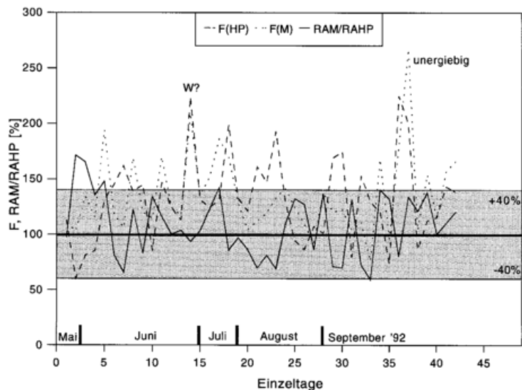
Bild 3: Variation der täglichen Radar-Aneichfaktoren F (Verhältnis Sammler-/Radar-Regenhöhe, unterbrochene Kurve) der Radars Höhenpeißenberg (HP) und München (M) an Niederschlagstagen von Mai bis Sept. 1992. Die mit F vergleichbaren Quotienten ( RAM/RAHP ) der Radarwerte zueinander (ausgezogene Kurve) liegen bei deutlich einheitlicheren Faktoren um 100% ( \pm 40\% , gründerter Bereich) als die auf die Sammler bezogenen Faktoren F . W steht für Aufgleitniederschlag mit erwartetem Aneichfaktor um 200%.
