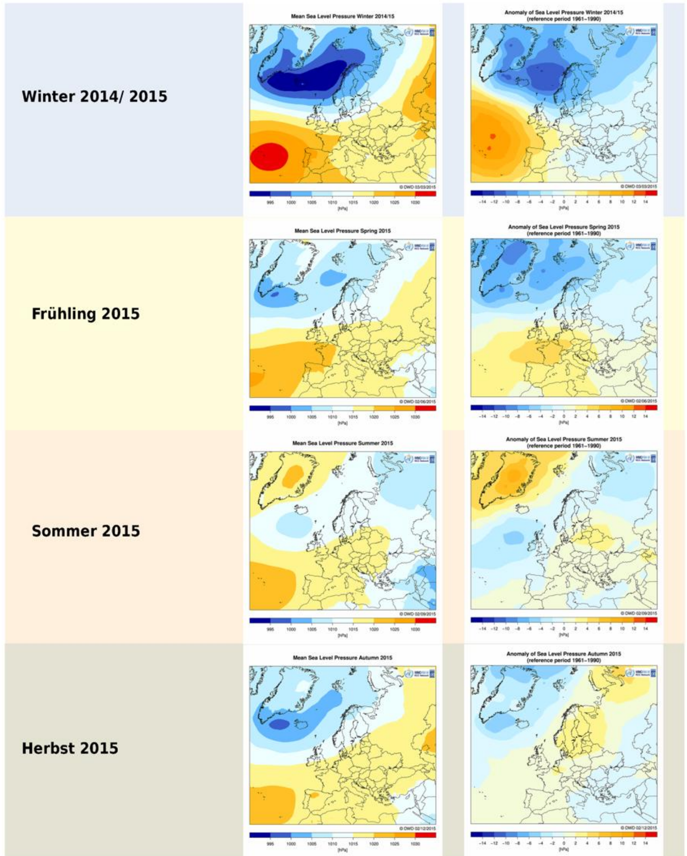
Abb. 7: Mittelwerte des Luftdrucks auf Meeresebene in hPa (links) und deren Anomalien (rechts) vom langjährigen Mittel 1961-1990 für die Jahreszeiten Winter 2014/2015, Frühling 2015, Sommer 2015 und Herbst 2015
