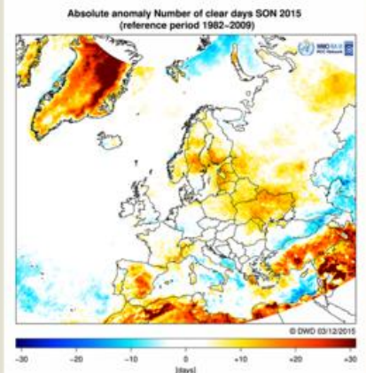
Abb. 11: Anzahl heiterer Tage (links) und deren Abweichungen (rechts) vom langjährigen Mittel 1982-2009 aus Sattelitebeobachtungen für die Jahreszeiten Winter 2014/2015, Frühling 2015, Sommer 2015 und Herbst 2015
