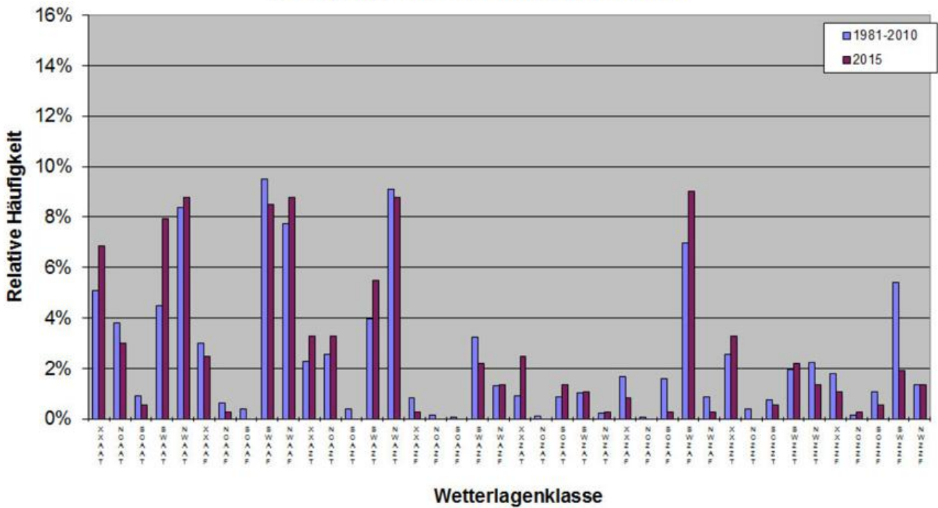
Abb. 1: Relative Häufigkeitsverteilung der objektiven Wetterlagenklassen 2015 im Vergleich zum 30-jährigen Zeitraum 1981-2010
