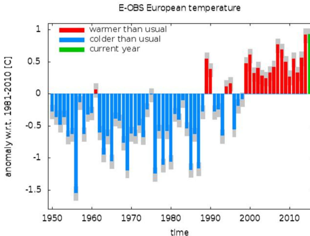
Abb. 1: Abweichungen der Jahresmitteltemperatur der Periode 1950-2015 (2 m) vom vieljährigen Mittel 1981-2010 in °C für die Landstationen im Gebiet 35°-75°N und 25°W-45°E (nach Verver et. al. 2013)
