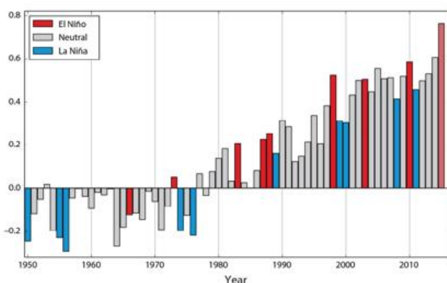
Abb. 1: Anomalien der Jahreswerte der Globaltemperatur als Mittel der 3 globalen Datensätze HadCRUT, NOAAGlobal-Temp, GISTEMP (Referenzzeitraum 1961-1990) als Balken. Durch El Niño beeinflusst: rot, La Niña: blau, ohne starken Einfluss (neutral): grau
