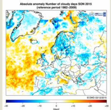
Abb. 10: Anzahl trüber Tage (links) und deren Abweichungen (rechts) vom langjährigen Mittel 1982-2009 aus Sattellitenbeobachtungen für die Jahreszeiten Winter 2014/2015, Frühling 2015, Sommer 2015 und Herbst 2015
