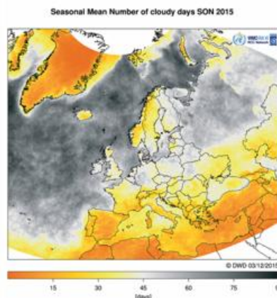
Abb. 10: Anzahl trüber Tage (links) und deren Abweichungen (rechts) vom langjährigen Mittel 1982-2009 aus Sattellitenbeobachtungen für die Jahreszeiten Winter 2014/2015, Frühling 2015, Sommer 2015 und Herbst 2015
