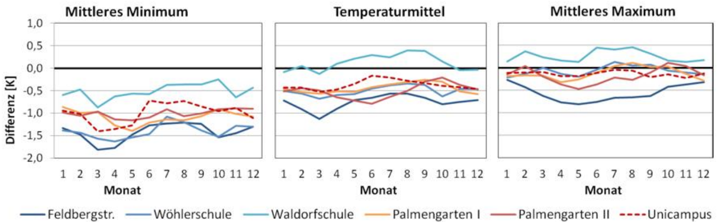
Abb. 1: Vergleich der monatlichen Mittelwerte der Lufttemperatur verschiedener Standorte der Frankfurter Innenstadtstation mit den Werten der Station Frankfurt-Flughafen (siehe Tab. 2); Standort Palmengarten für Vergleichszwecke mit den anderen Stationen in zwei ähnlich lange Perioden getrennt: 11/1985 bis 1996 (I) und 1997 bis 7/2008 (II)
