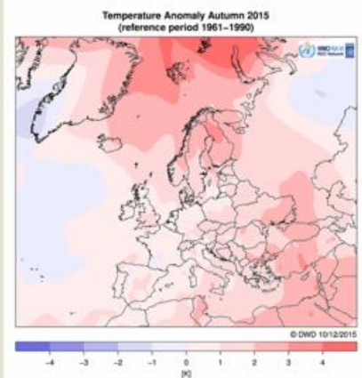
Abb. 3: Mittlere Lufttemperatur (in 2 m Höhe) in °C im Winter 2014/2015, Frühjahr 2015, Sommer 2015 und Herbst 2015 (linke Spalte) und die dazugehörigen mittlere Anomalie der Lufttemperatur (in 2 m Höhe) in K (rechte Spalte; Quelle: http://www.dwd.de/rcc-cm )
