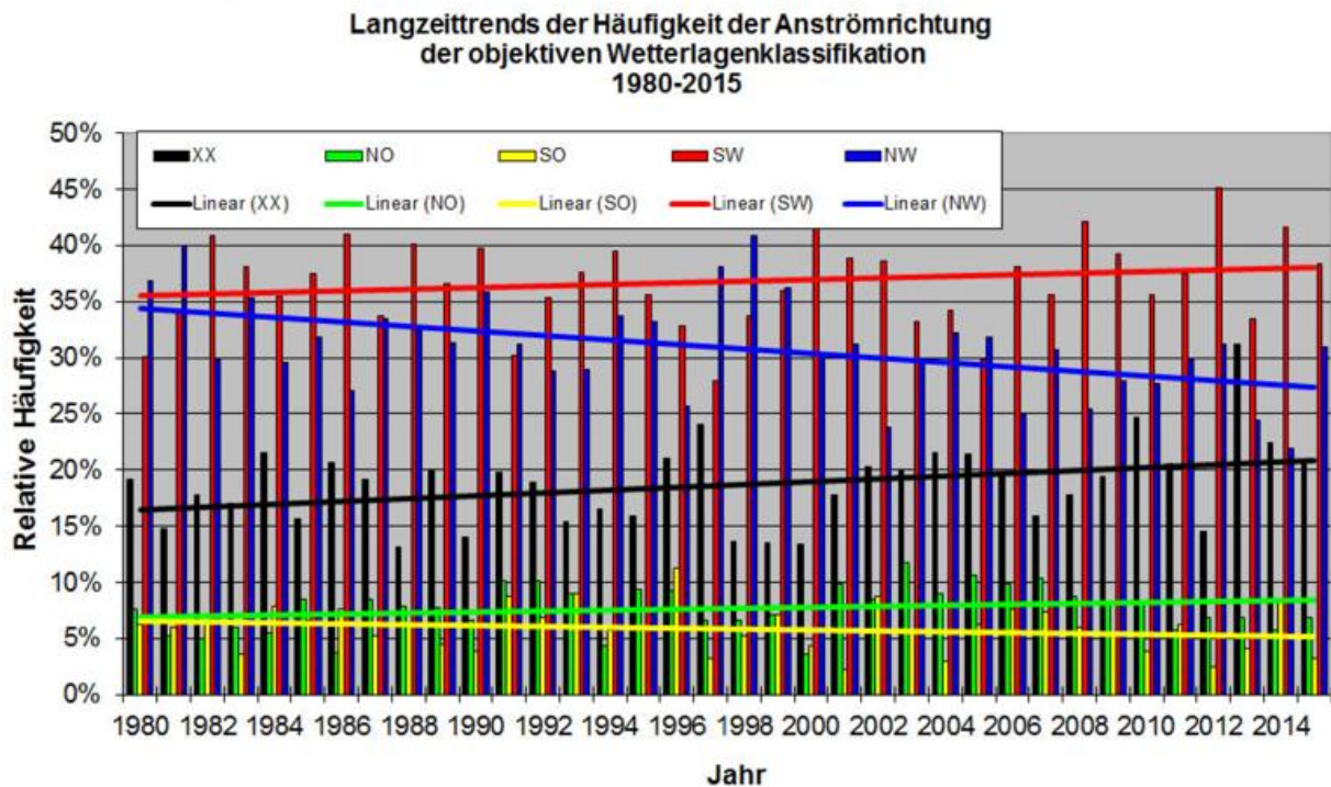
Abb. 4: Langzeittrends der Häufigkeit der Anströmrichtungen der objektiven Wetterlagenklassifikation 1980-2015
