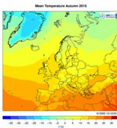
Abb. 3: Mittlere Lufttemperatur (in 2 m Höhe) in °C im Winter 2014/2015, Frühjahr 2015, Sommer 2015 und Herbst 2015 (linke Spalte) und die dazugehörigen mittlere Anomalie der Lufttemperatur (in 2 m Höhe) in K (rechte Spalte; Quelle: http://www.dwd.de/rcc-cm )
