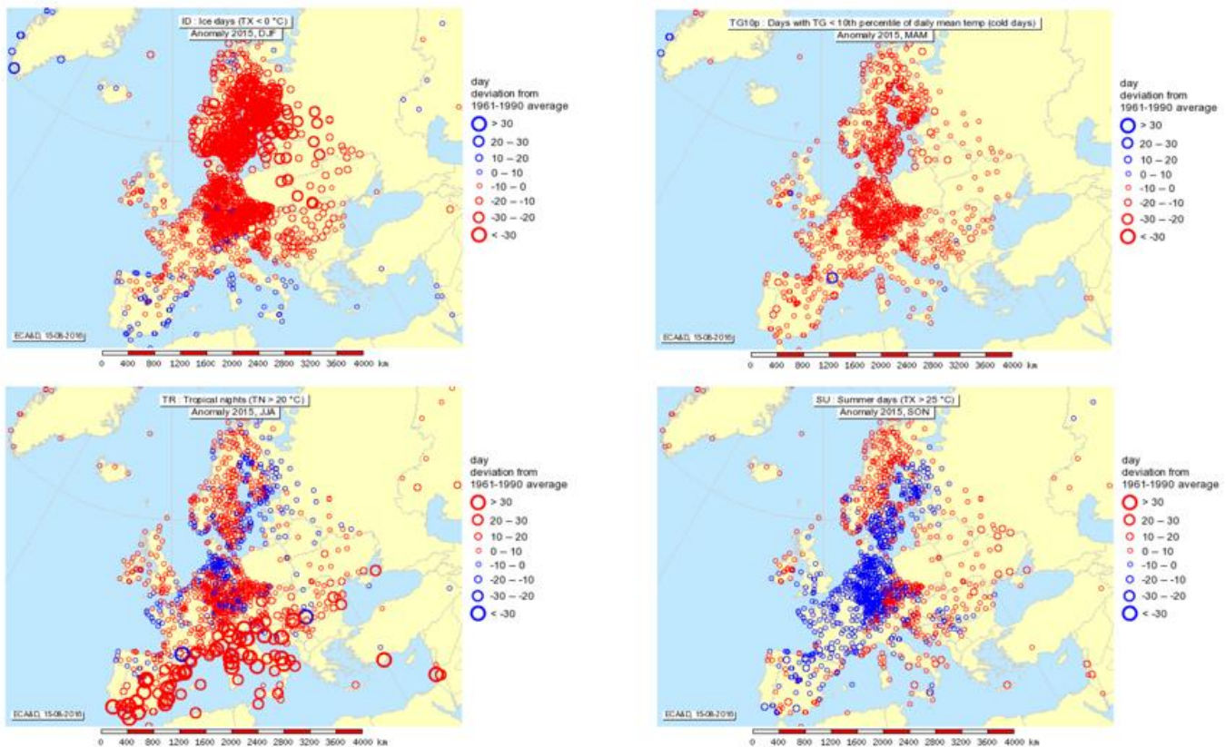
Abb. 12: Jahreszeitliche Anomalien ausgewählter Temperaturindizes nach ECA&D für Winter (links oben; ID (ice days) Eistage: Maximumtemperatur <0°C), Frühjahr (rechts oben; TG10p, Kalte Tage oder Tage mit Tagesmitteltemperatur unter dem 10 %-Perzentilwert), Sommer (links unten; TR Tropennächte: Minimumtemperatur >20°C) und Herbst (rechts unten; SU Sommertage Maximumtemperatur >25°C)
