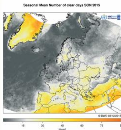
Abb. 11: Anzahl heiterer Tage (links) und deren Abweichungen (rechts) vom langjährigen Mittel 1982-2009 aus Sattelitebeobachtungen für die Jahreszeiten Winter 2014/2015, Frühling 2015, Sommer 2015 und Herbst 2015
