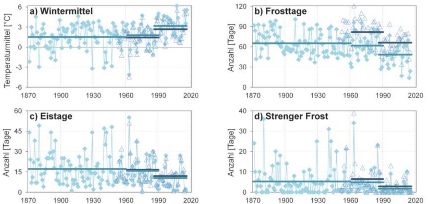
Abb. 5: Übersicht verschiedener Temperaturkenntage zur Charakterisierung der Winterkälte für 1870/71-2015/16; Linien: 11-jährig gleitende Mittelwerte; türkisarbenne Markierungen/Linien beziehen sich auf die Zeitreihe Frankfurt-Innenstadt, blaue Markierungen/Linien auf die Kombination Innenstadt bis 1950/Flughafen ab 1951; Mittelwerte 1870-1960, 1961-1990 und 1986-2015; Wintermittel: Dezember, Januar, Februar; Anzahl Kenntage: Summe Juli bis Juni für Frosttage (Minimum <0^{\circ}\text{C} ), Eistage (Maximum <0^{\circ}\text{C} ) und Tage mit strengem Frost (Minimum \leq -10^{\circ}\text{C} )
