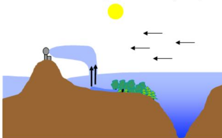
Abb. 2: Skizze des Hohen Peißenbergs und des südlichen Hangfußbereichs. Dargestellt ist der frei konvektive Aufstieg eines bodennahen Luftpaketes mit anschließendem Transport zum Observatorium.
