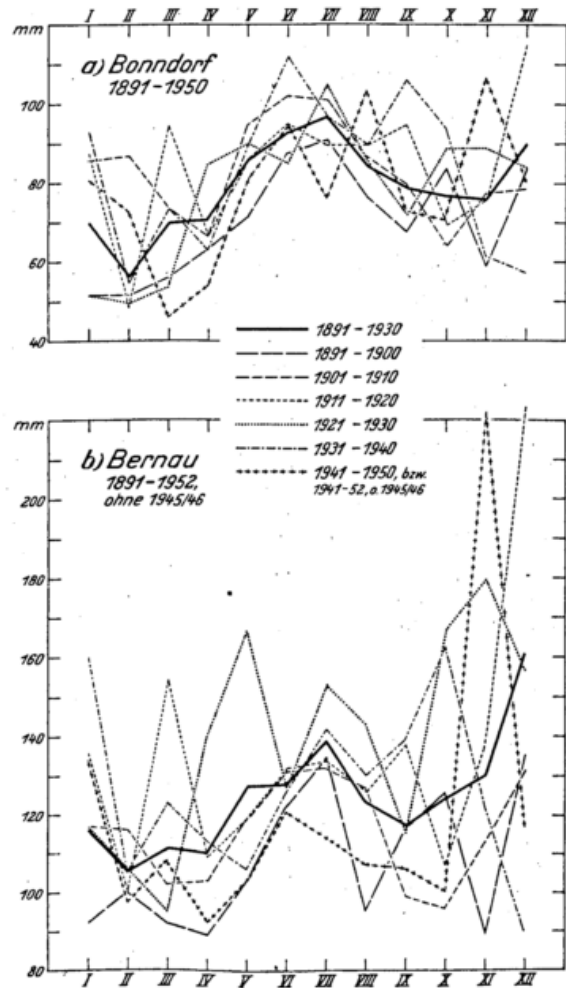
Abb. 3 Dezennienmittel der Monatssummen des Niederschlags (mm)
