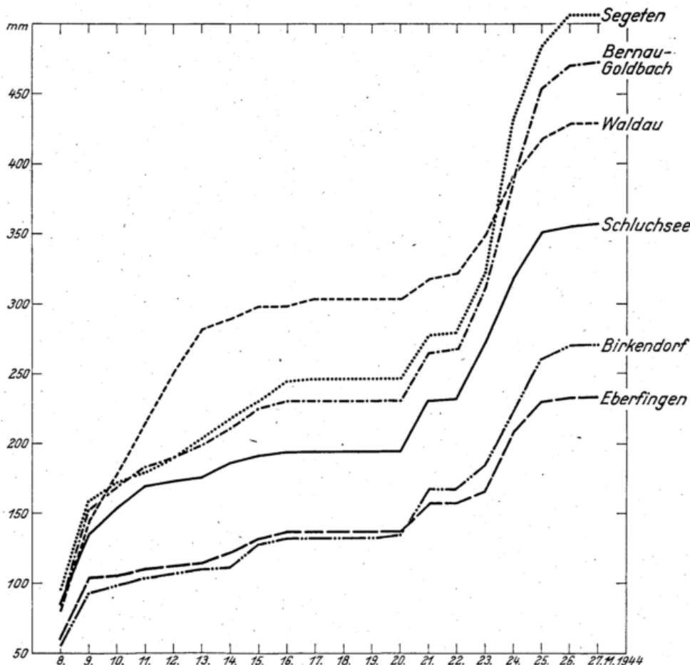
Abb. 7 Tagessummen des Niederschlags (mm) vom 8. 11. — 27. 11. 1944
