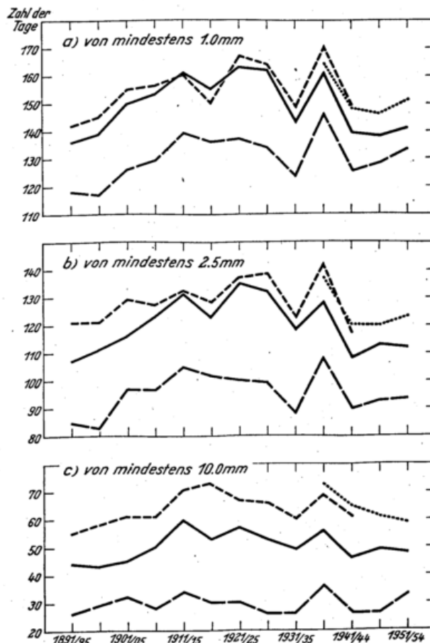
Abb. 5 Lustrenmittel der Zahl der Tage mit Niederschlag Zeitraum: 1891—1954 — Bernau — — Bonndorf ..... Segeten - - - Todtmoos
