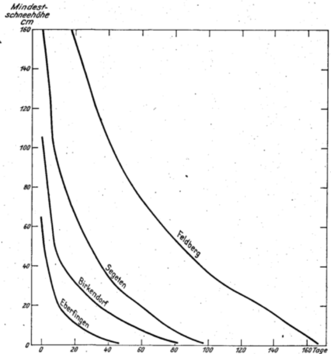
Abb. 14 Mittlere jährliche Zahl der Tage mit Schneedecke verschiedener Schneehöhen. Zeitraum: 1936/37—1943/44, 1946/47—1952/53
