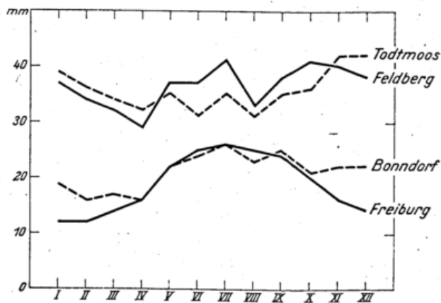
Abb. 6. Mittlere größte Tagessummen des Niederschlags von Freiburg, Bonndorf, Todtmoos, Feldberg Zeitraum: 1891—1940
