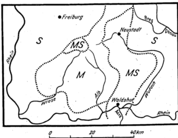
Abb. 2 Typen im mittleren Jahresgang des Niederschlags Zeitraum: 1891—1930
