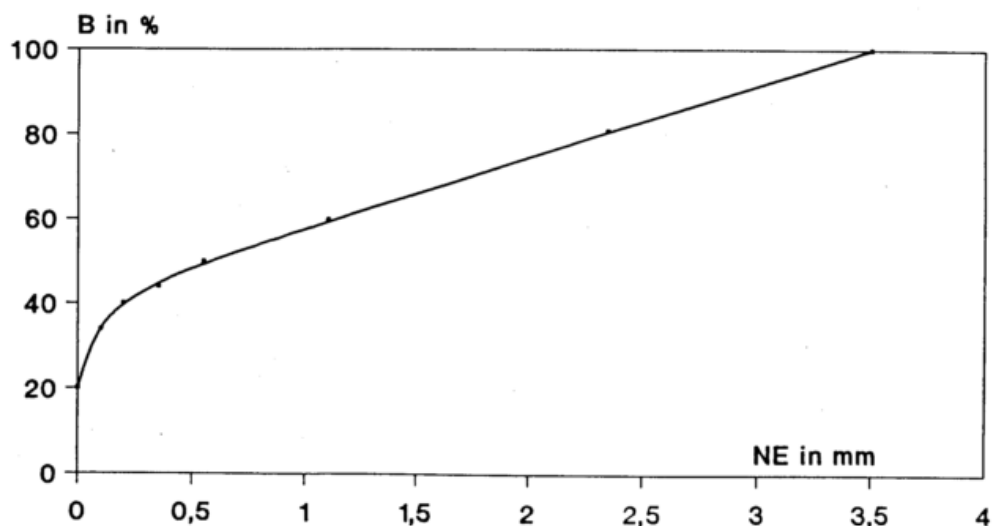
Abb.1: Mittlere Zunahme der prozentualen Benetzung (B) des Auffangtrichters mit der Höhe des Niederschlagsereignisses (NE)
