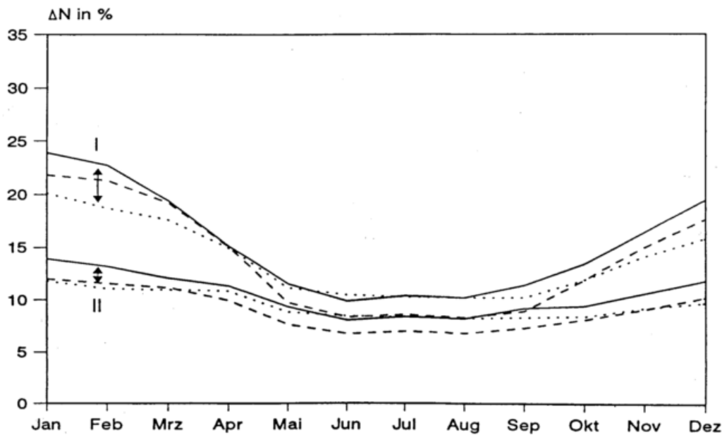
Abb.25: Mittlerer Jahresgang des Niederschlagsmeßfehlers \Delta N bei freier (I) und mäßig geschützter Stationslage (II) : — Südwestdeutschland, - - Schwarzwald (<700m), - - - westl. Saarland
