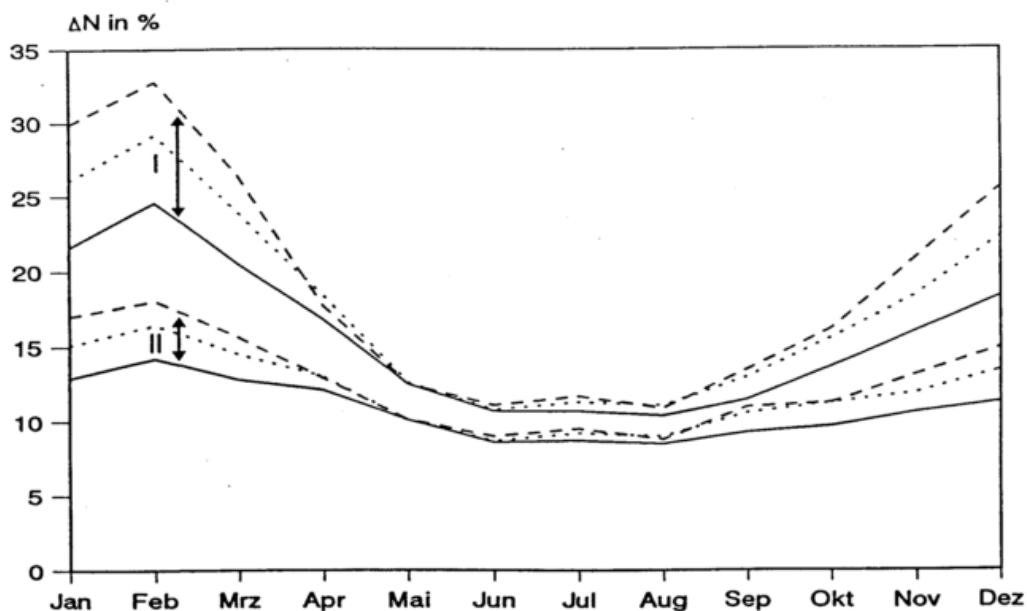
Abb.23: Mittlerer Jahresgang des Niederschlagsmeßfehlers \Delta N im Norddeutschen Tiefland bei freier (I) und mäßig geschützter Stationslage (II) : — westlicher Bereich, ..... mittlerer Bereich, - - - östlicher Bereich
