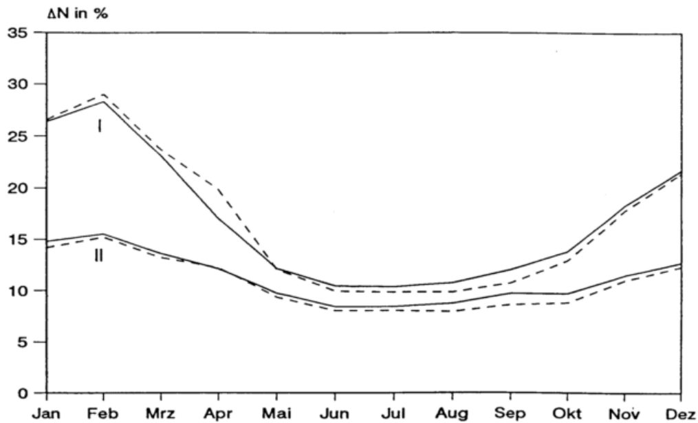
Abb.27: Mittlerer Jahresgang des Niederschlagsmeßfehlers \Delta N im Bereich der westlichen Mittelgebirge bei freier (I) und mäßig geschützter Stationslage (II): — Höhenlage 200 bis 400 m, - - - Höhenlage 400 bis 700 m
