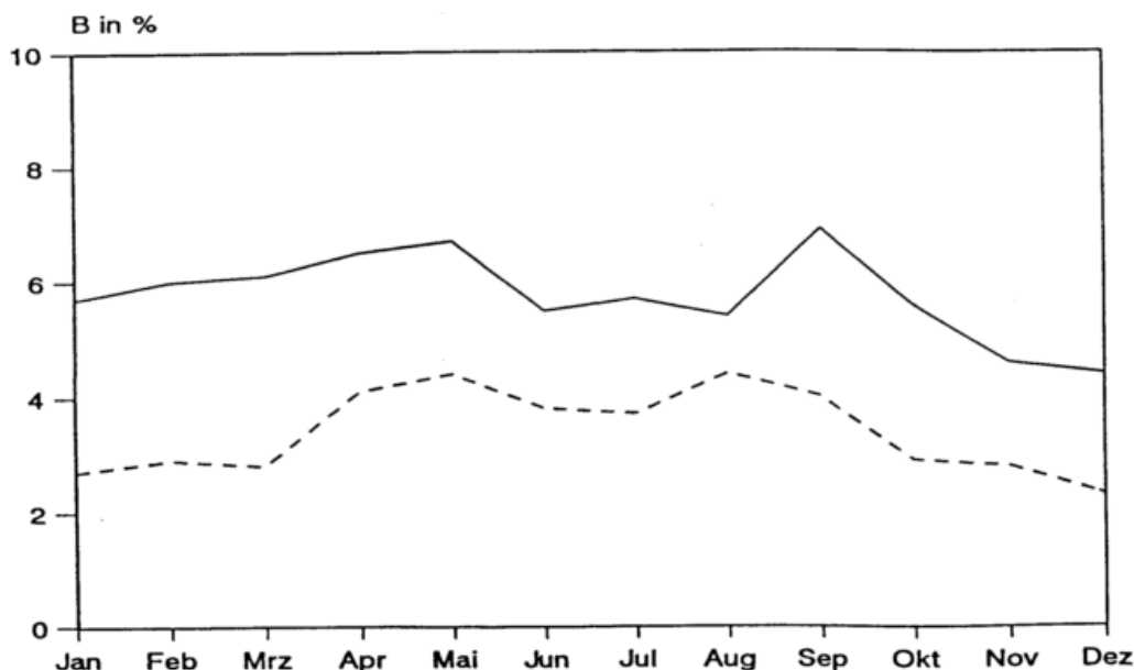
Abb.4: Mittlerer Jahresgang der prozentualen Benetzungsverluste (B) des Auffangtrichters für Tiefland- (—) und Mittelgebirgsstationen (- -)
