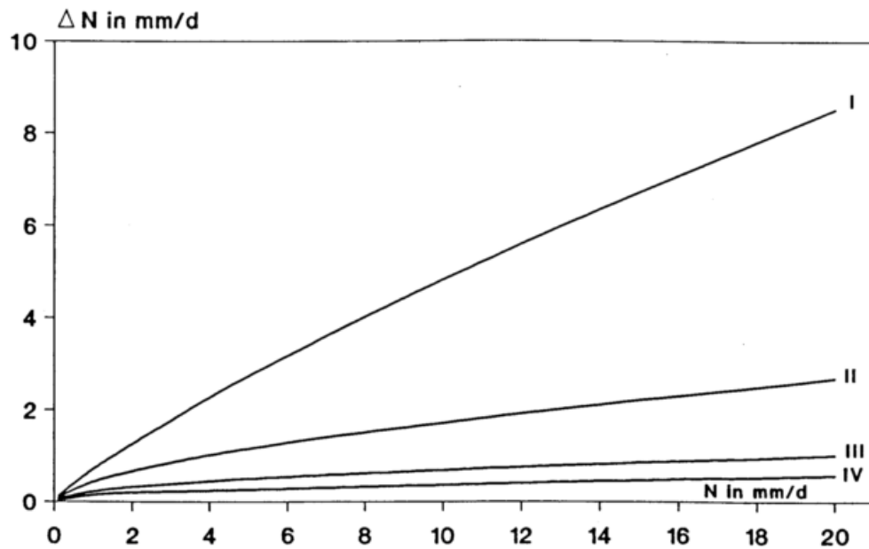
Abb.14: Mittlere Zunahme des Windfehlers \Delta N für Tageswerte der Niederschlags- höhe (N) bei freier Stationslage I: Schnee, II: Mischniederschlag, III: Regen(Winter), IV: Regen(Sommer)
