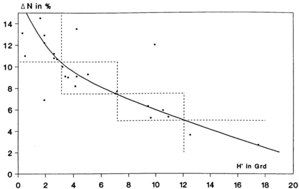
Abb.8: Mittlere Horizontabschirmung (H') im Sektor S bis N (gewichtet) und mittlerer gemessener Windfehler \Delta N
