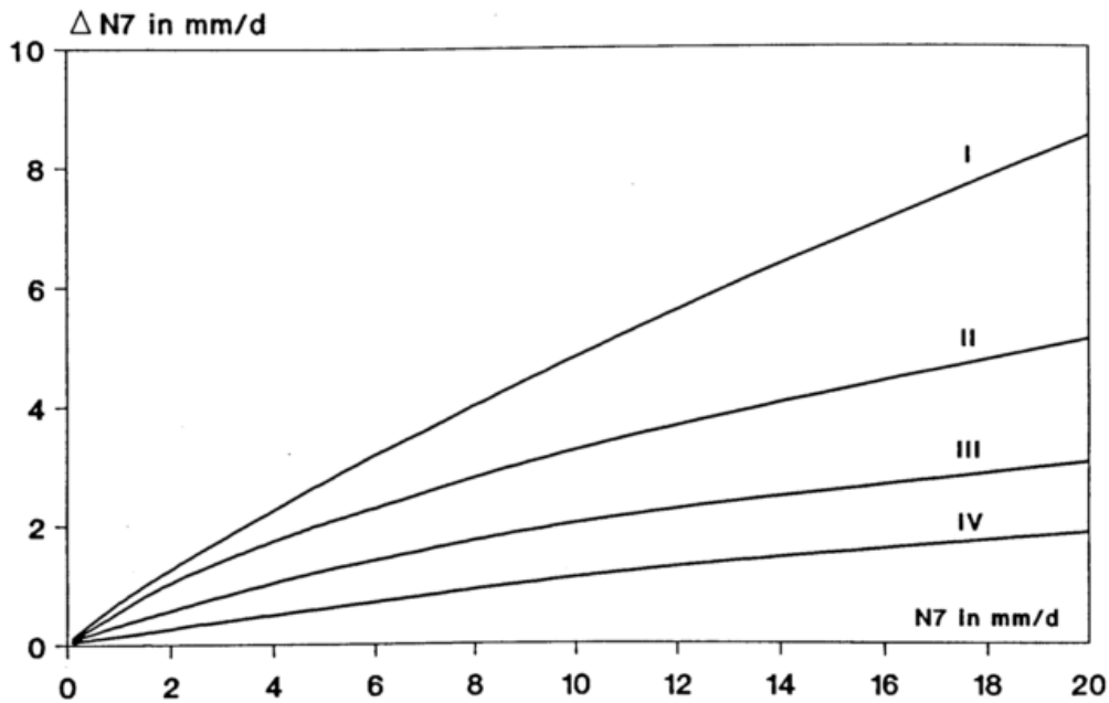
Abb.13: Mittlere Zunahme des Windfehlers bei Schneefall \Delta N7 für Tageswerte der Niederschlagshöhe (N7), I: freie, II: leicht geschützte, III: mäßig geschützte, IV: stark geschützte Stationslage
