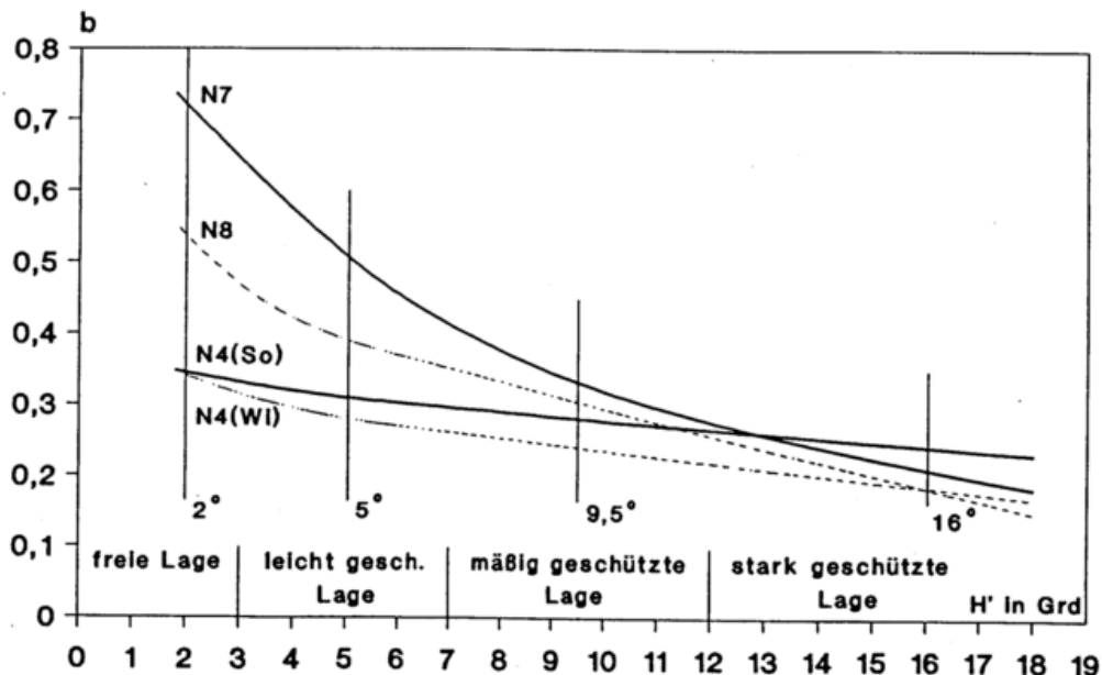
Abb.18: Abhängigkeit des Koeffizienten b der Niederschlagskorrekturfunktion \Delta N = b \cdot N^c von der Horizontabschirmung ( H' ) für die Niederschlagsarten N4(So,Wi), N8 und N7
