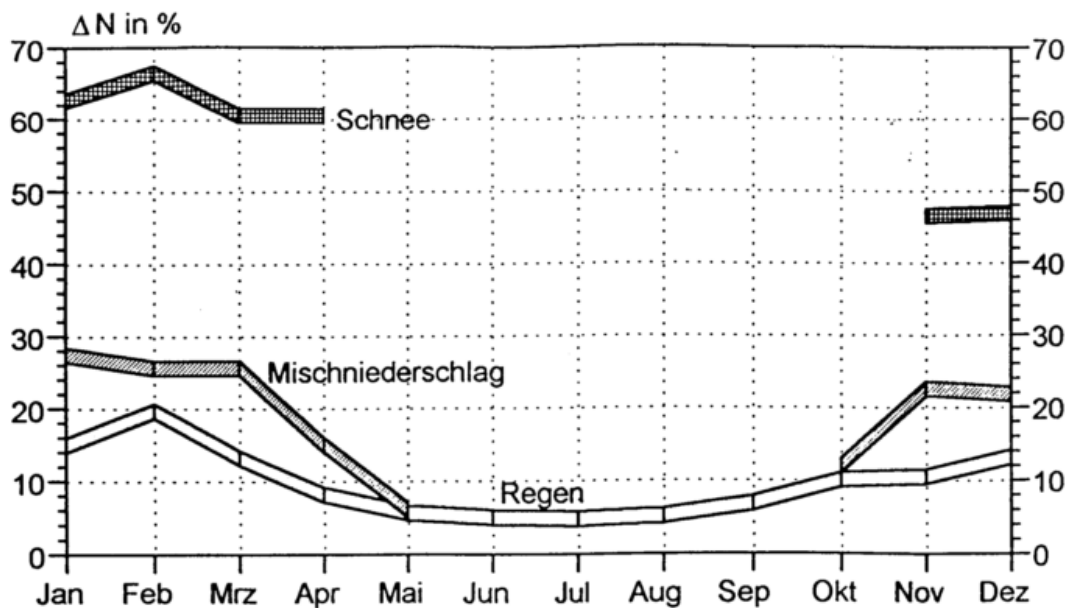
Abb.10: Mittlerer Jahresgang des Windfehlers \Delta N bei freier Stationslage
