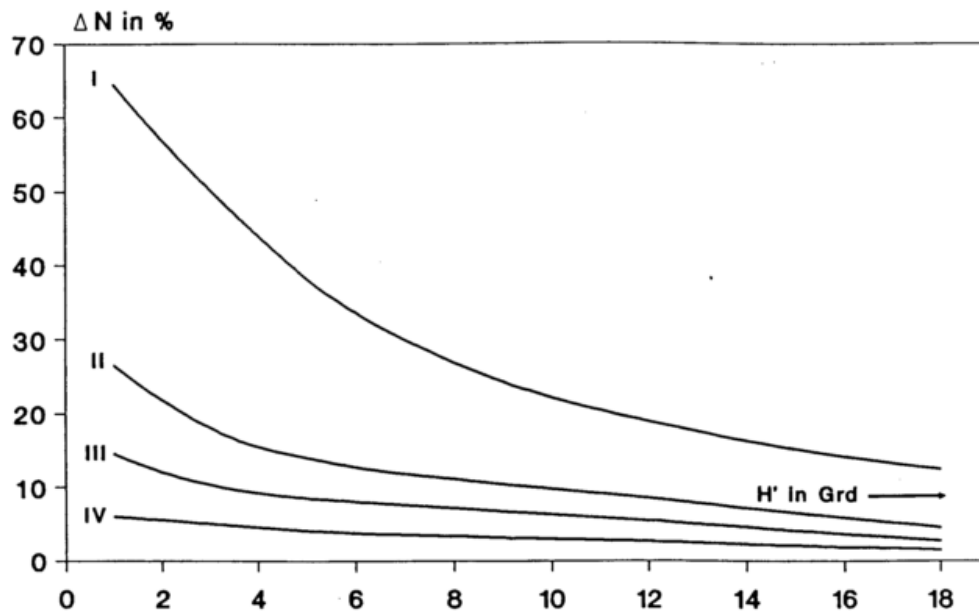
Abb.16: Abnahme des mittleren Windfehlers \Delta N mit der Horizontabschirmung H' I: Schnee, II: Mischniederschlag, III: Regen(Winter), IV: Regen(Sommer)
