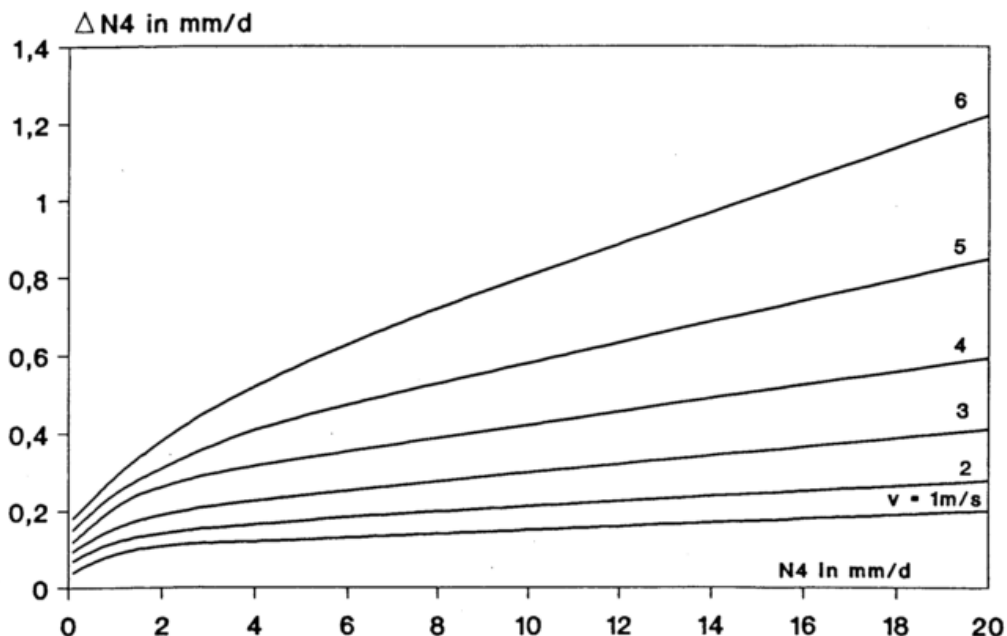
Abb.11: Mittlere Zunahme des Windfehlers bei Regen \Delta N4 in Abhängigkeit von der Niederschlagshöhe (N) und der Windgeschwindigkeit (v) in 1m Höhe, Harzgerode 1977/93
