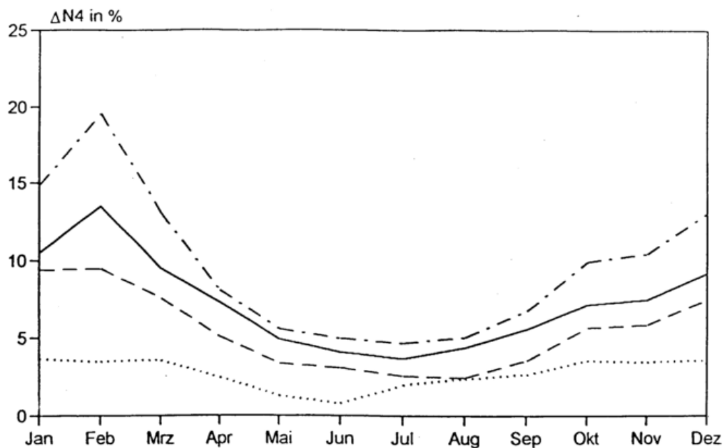
Abb.9: Mittlerer Jahresgang des Windfehlers bei flüssigem Niederschlag \Delta N_4 , Reihe 1983/1993
