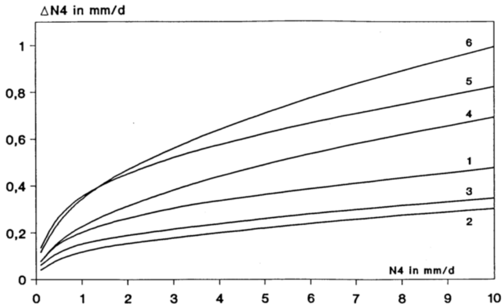
Abb.17: Mittlere Zunahme der Fehler mit der Niederschlagshöhe bei Regen, freie Stationslage: Benetzung und Verdunstung im Sommer(1) und Winter(2), Windfehler im Sommer(3) und Winter(4), Gesamtfehler im Sommer(5) und Winter(6)
