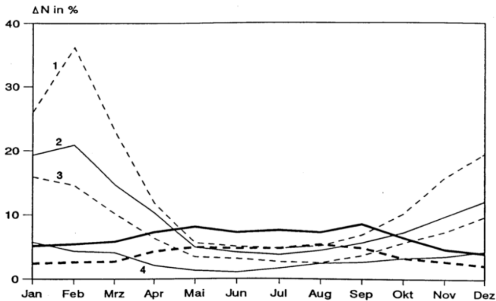
Abb.15: Mittlerer Jahresgang des gemessenen Windfehlers für 1. --- freie, 2. — leicht geschützte 3. --- mäßig geschützte und 4. — stark geschützte Stationslagen sowie des Benetzungs- und Verdunstungsfehlers für Tiefland (—) und Mittelgebirgsstationen (---)
