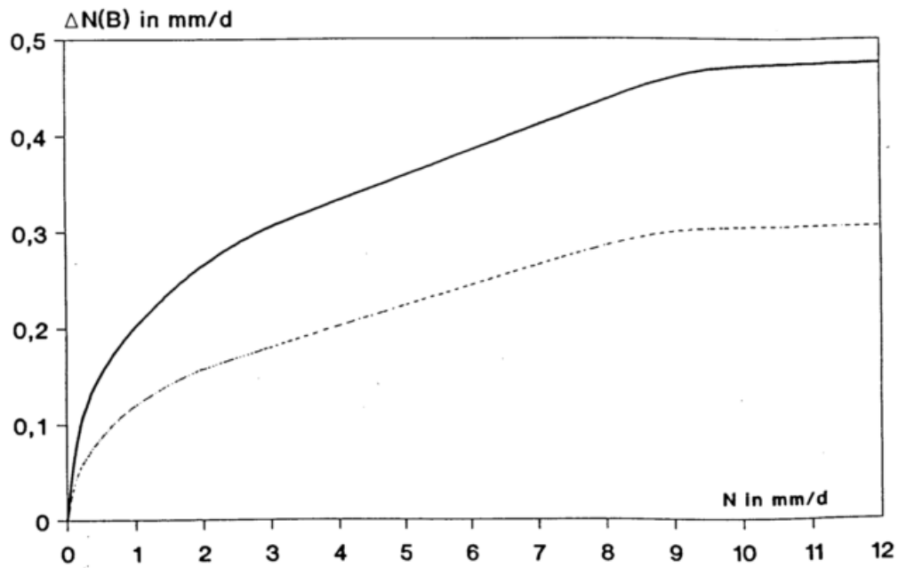
Abb.6: Mittlere Zunahme der Benetzungs- und Verdunstungsfehler \Delta N(B) mit der täglichen Niederschlagshöhe ( N ), — Sommerhalbjahr, --- Winterhalbjahr
