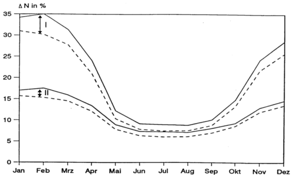
Abb.29: Mittlerer Jahresgang des Niederschlagsmeßfehlers \Delta N bei freier(I) und mäßig geschützter Stationslage (II) : — Mittelgebirge(>700m), - - - Alpen (700 bis 1000m)
