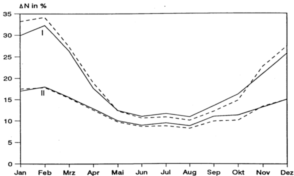
Abb.30: Mittlerer Jahresgang des Niederschlagsmeßfehlers \Delta N bei freier(I) und mäßig geschützter Stationslage (II) : — Gebiet III, --- Gebiet V (siehe Abb.28)
