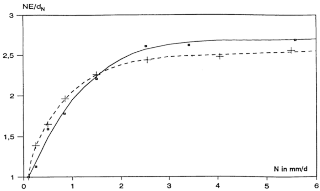
Abb.5: Mittlere Anzahl der Niederschlagsereignisse pro Niederschlagstag ( NE/d_N ) in Abhängigkeit von der Niederschlagshöhe ( N ), — Sommerhalbjahr, - - Winterhalbjahr
