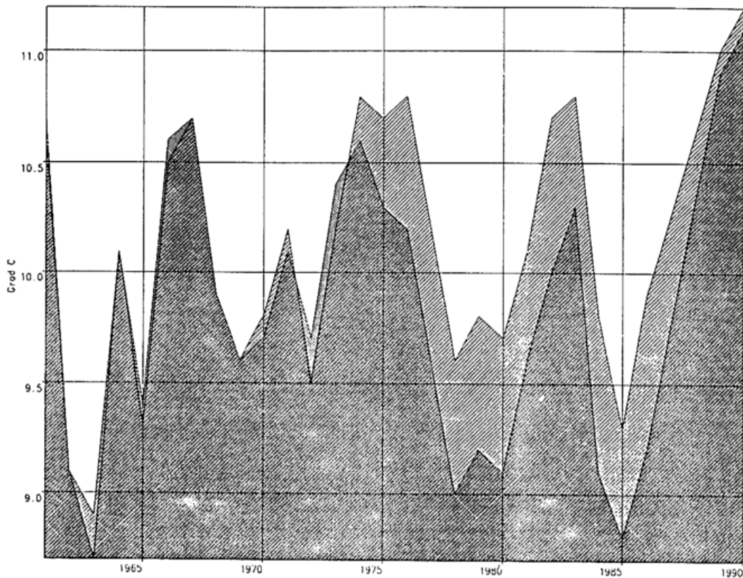
Abbildung 3: Zeitlicher Verlauf der zu prüfenden Meßreihe und der Referenzreihe für die Jahresmitteltemperatur der Station Bad Dürkheim
