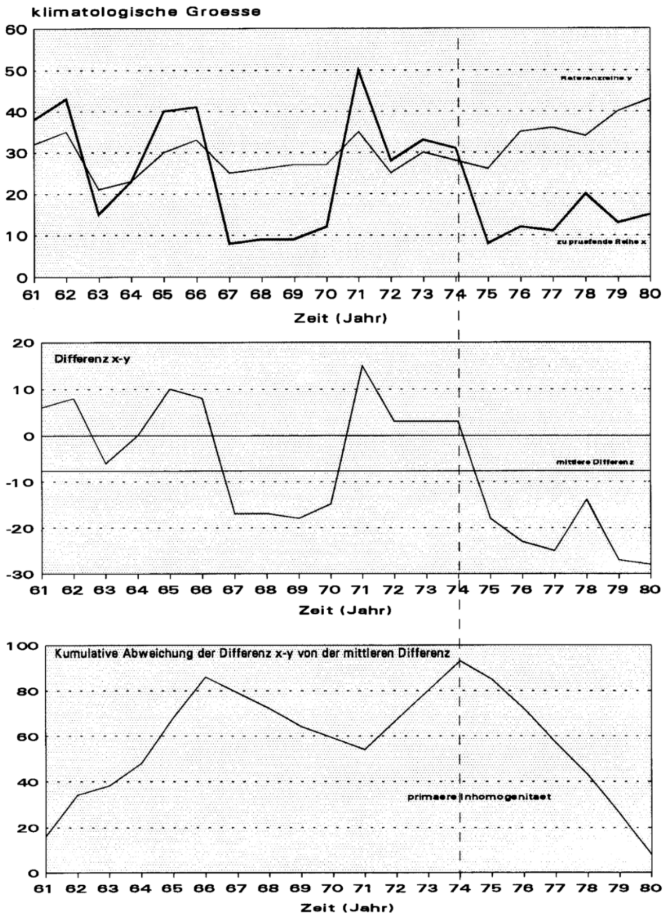
Abbildung 1: Schematische Darstellung der Homogenitätsprüfung mit dem Buishandtest
