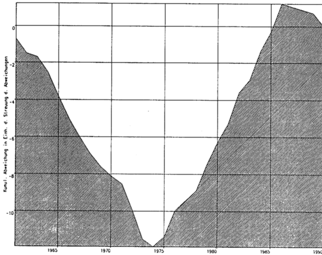
Abbildung 5: Zeitlicher Verlauf der kumulativen Abweichungen zwischen der zu prüfenden Meßreihe und der Referenzreihe für die Jahresmitteltemperatur der Station Bad Dürkheim
