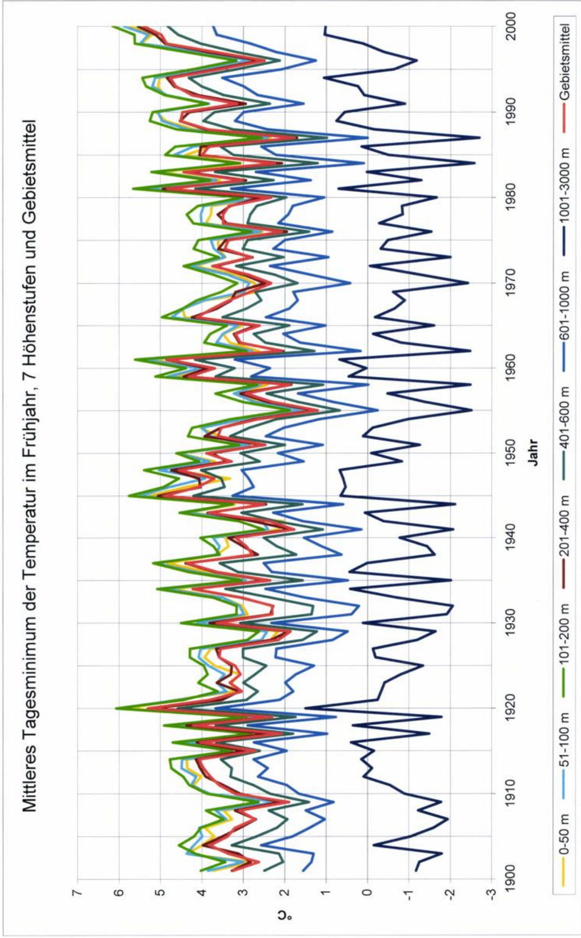
Abbildung 9 Mittleres Tagesminimum der Temperatur im Frühjahr, 7 Höhenstufen und Gebietsmittel
