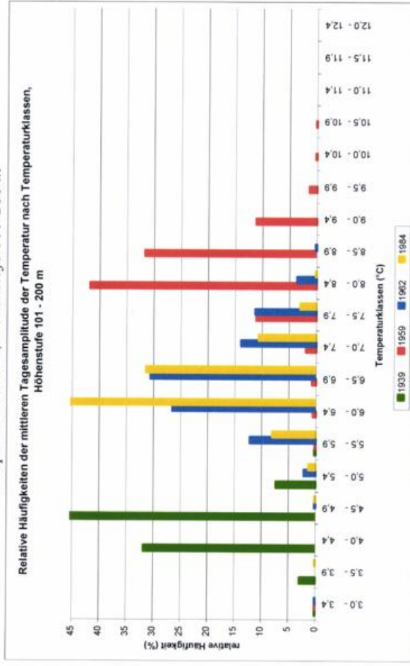
Abbildung 43 relative Häufigkeiten der mittleren Tagesamplitude der Temperatur nach Temperaturklassen, Höhenstufe 101-200 m
