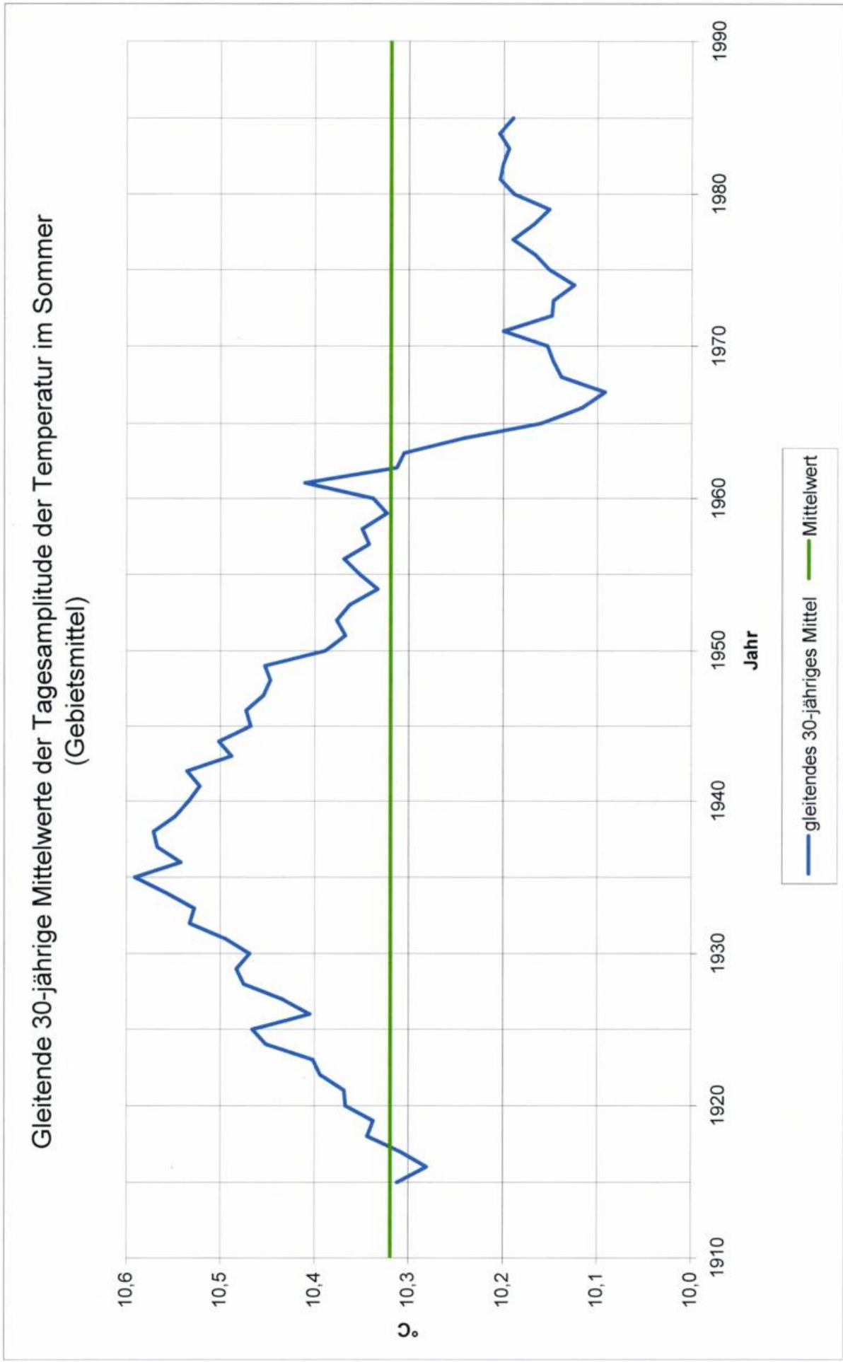
Abbildung 49 Gleitende 30-jährige Mittelwerte der Tagesamplitude der Temperatur im Sommer (Gebietsmittel)
