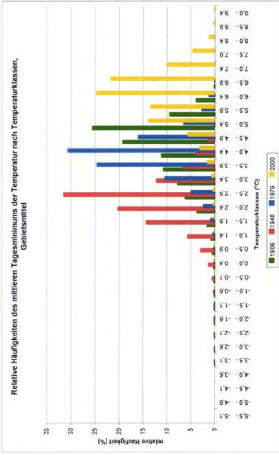
Abbildung 4 Relative Häufigkeiten des mittleren Tagesminimums der Temperatur nach Temperaturklassen, Gebietsmittel
