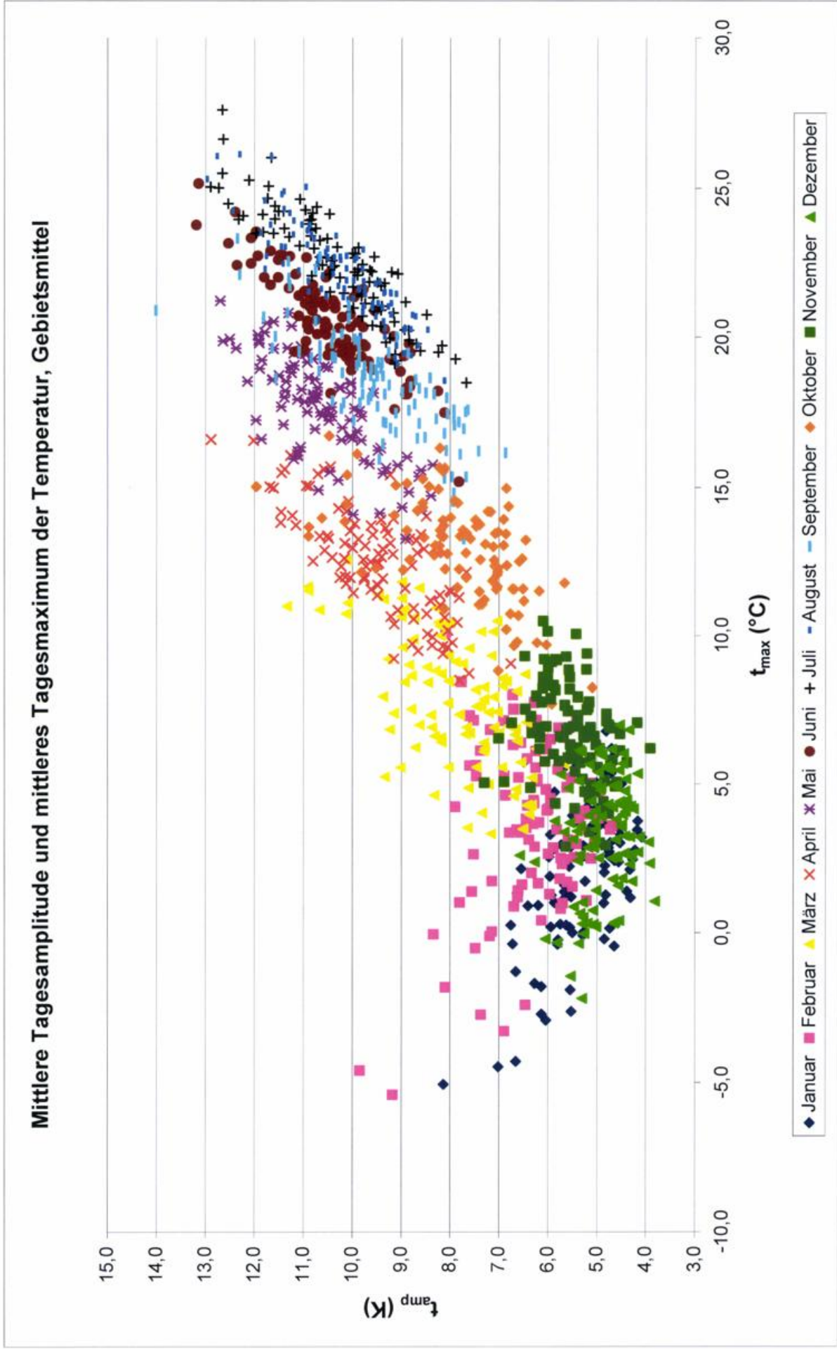
Abbildung 37 Mittlere Tagesamplitude und mittleres Tagesmaximum der Temperatur, Gebietsmittel
