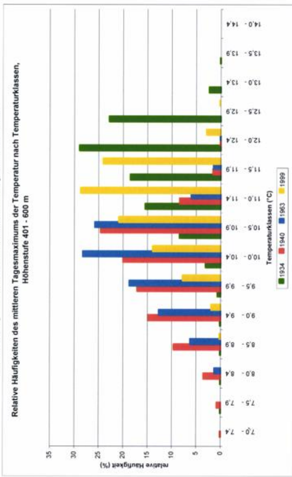
Abbildung 24 relative Häufigkeiten des mittleren täglichen Tagesmaximums der Temperatur nach Temperaturklassen, Höhenstufe 401-600 m
