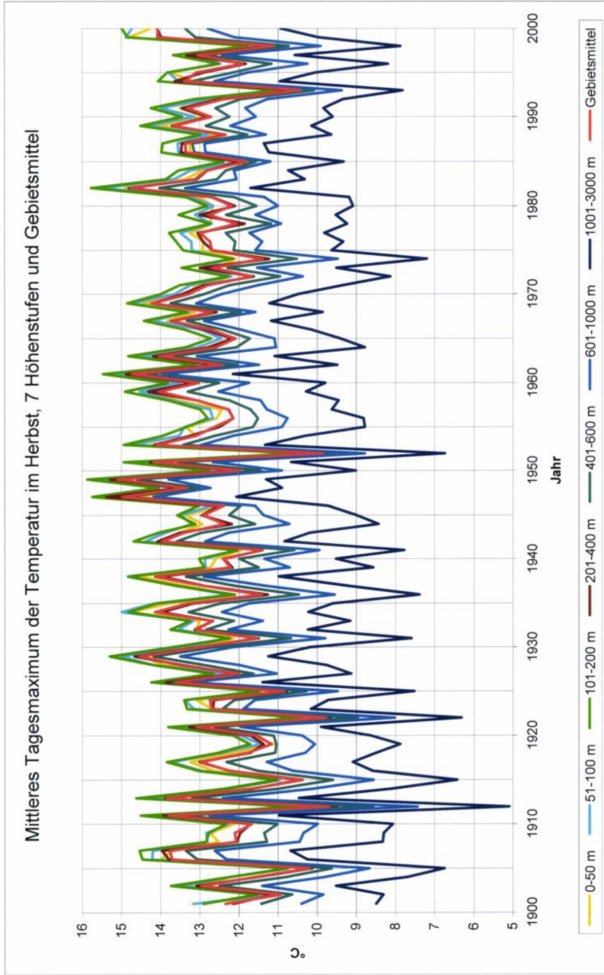
Abbildung 33 Mittleres Tagesmaximum der Temperatur im Herbst, 7 Höhenstufen und Gebietsmittel
