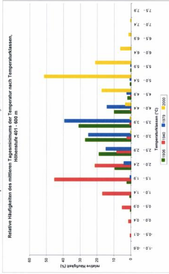
Abbildung 6 Relative Häufigkeiten des mittleren Tagesminimums der Temperatur nach Temperaturklassen, Höhenstufe 401-600 m
