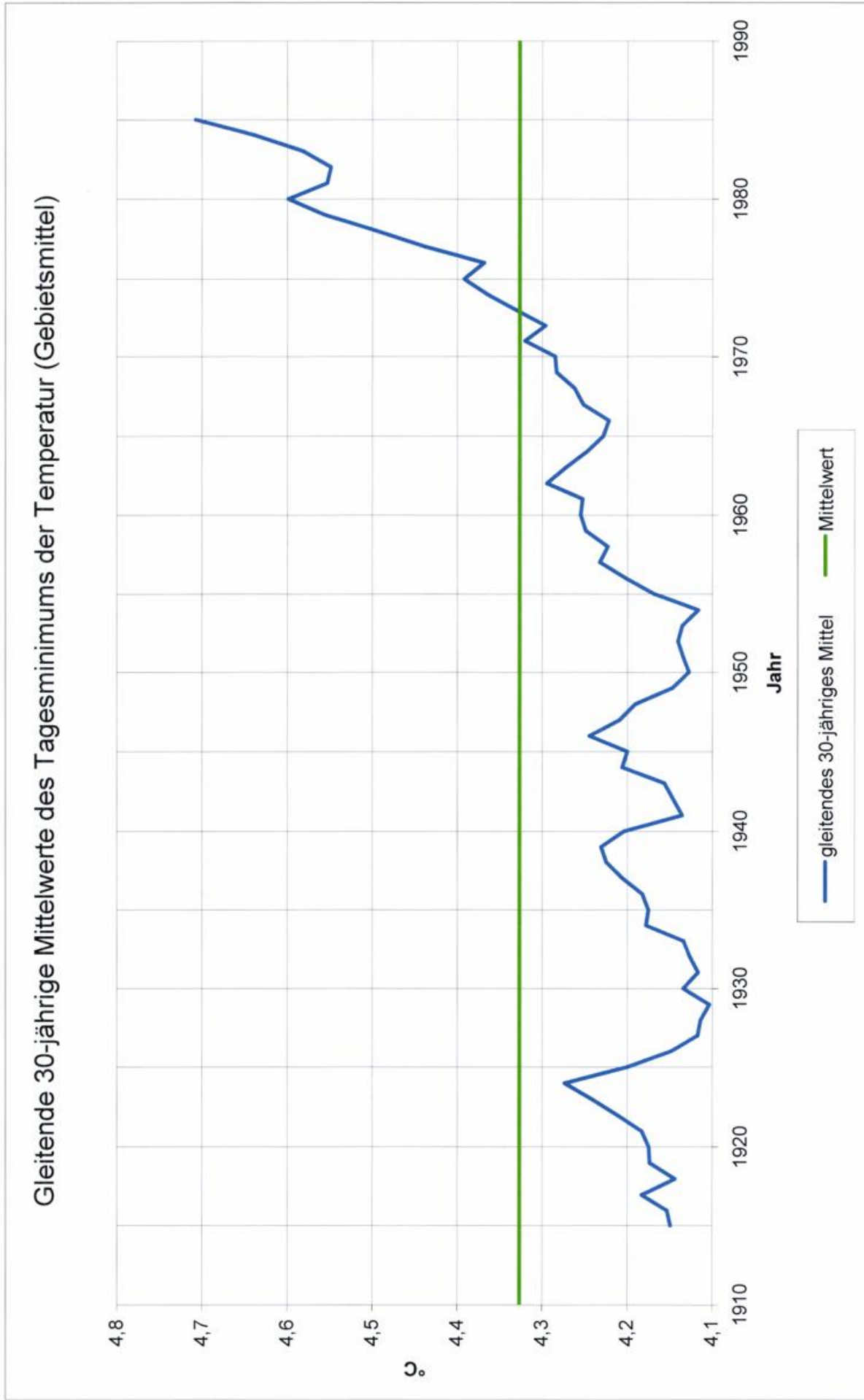
Abbildung 2 Gleitende 30-jährige Mittelwerte des Tagesminimums der Temperatur (Gebietsmittel)
