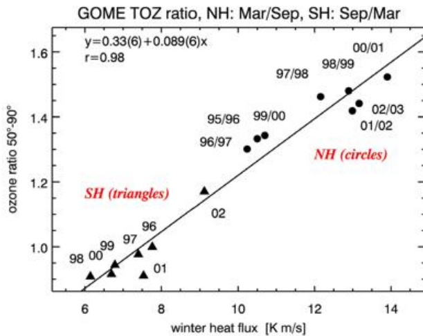
Abb. 2. Fröhling-Herbstverhältnis im hemisphärischen Ozon als Funktion des mittleren Wärmeflusses durch die 100 hPa Fläche.
