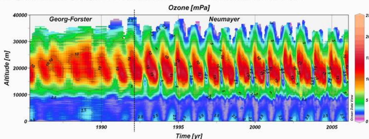
Abb. 2: Höhenzeitschnitt des Ozonpartialdruckes über Georg-Forster und Neumayer von 1985 -2006
