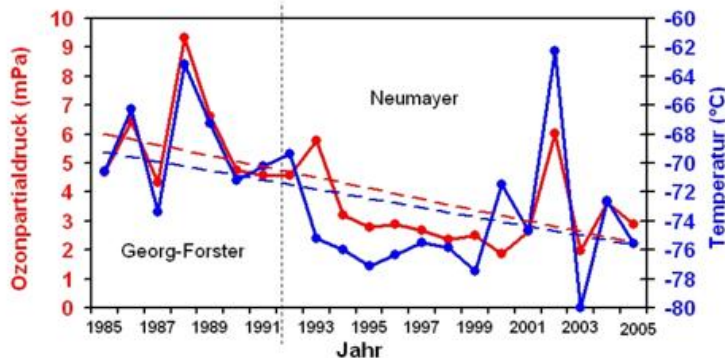
Abb.3: Zeitserien von über September, Oktober, November gemittelten Ozonpartialdrücken (rot) und Temperaturen (blau) in 70 hPa über Georg-Forster und Neumayer. Die entsprechenden linearen Trends sind gestrichelt eingezeichnet
