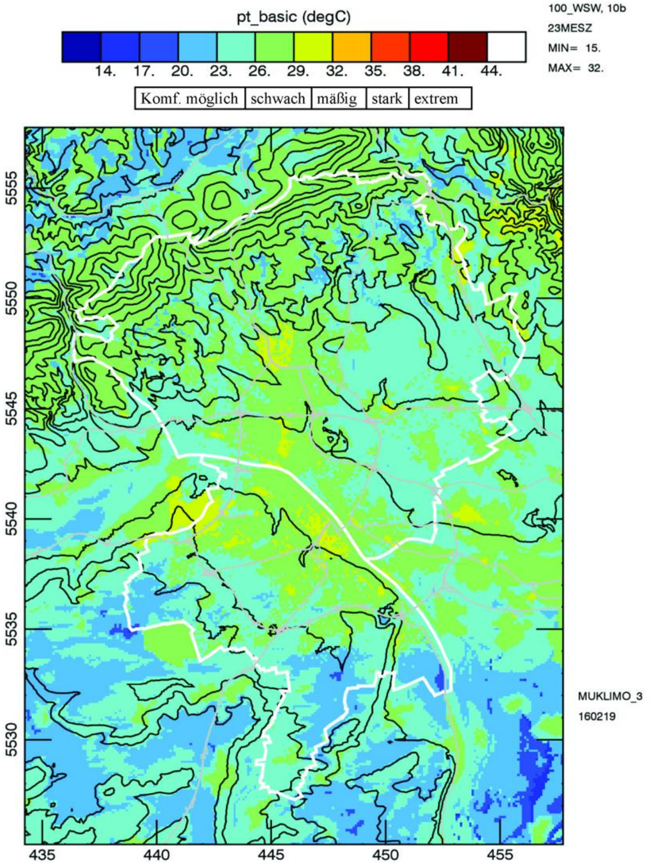
Abbildung 5-5: Wie Abbildung 5-4, aber für 23 MESZ.
