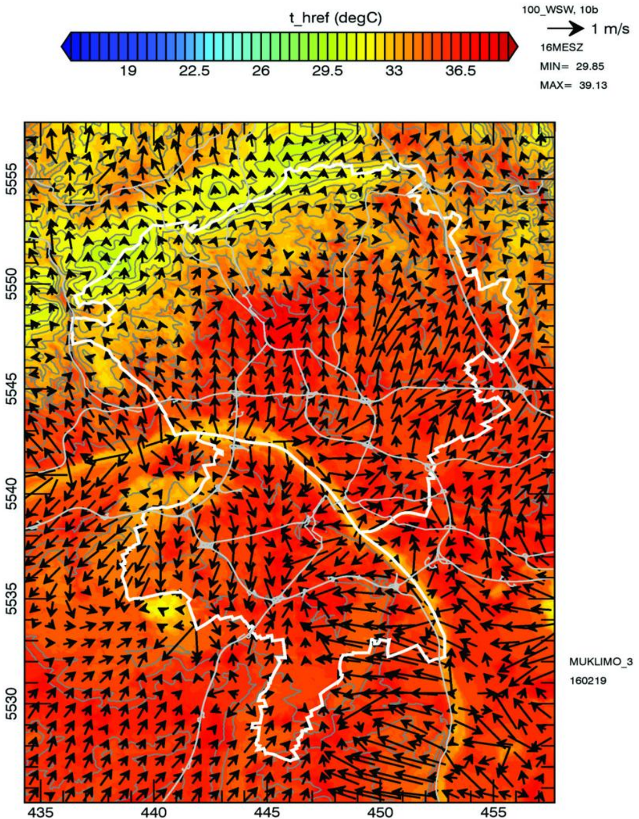
Abbildung 5-1: Windfeld und Lufttemperatur in 5 m über Grund ( t_{\text{href}} ) um 16 MESZ für einen heißen, trockenen, windschwachen Tag mit Anströmung aus WSW. Es ist nur jeder achte. Windpfeil entsprechend einem Abstand von 800 m dargestellt. Die hellgrauen Linien geben die Hauptverkehrsstraßen wieder.
