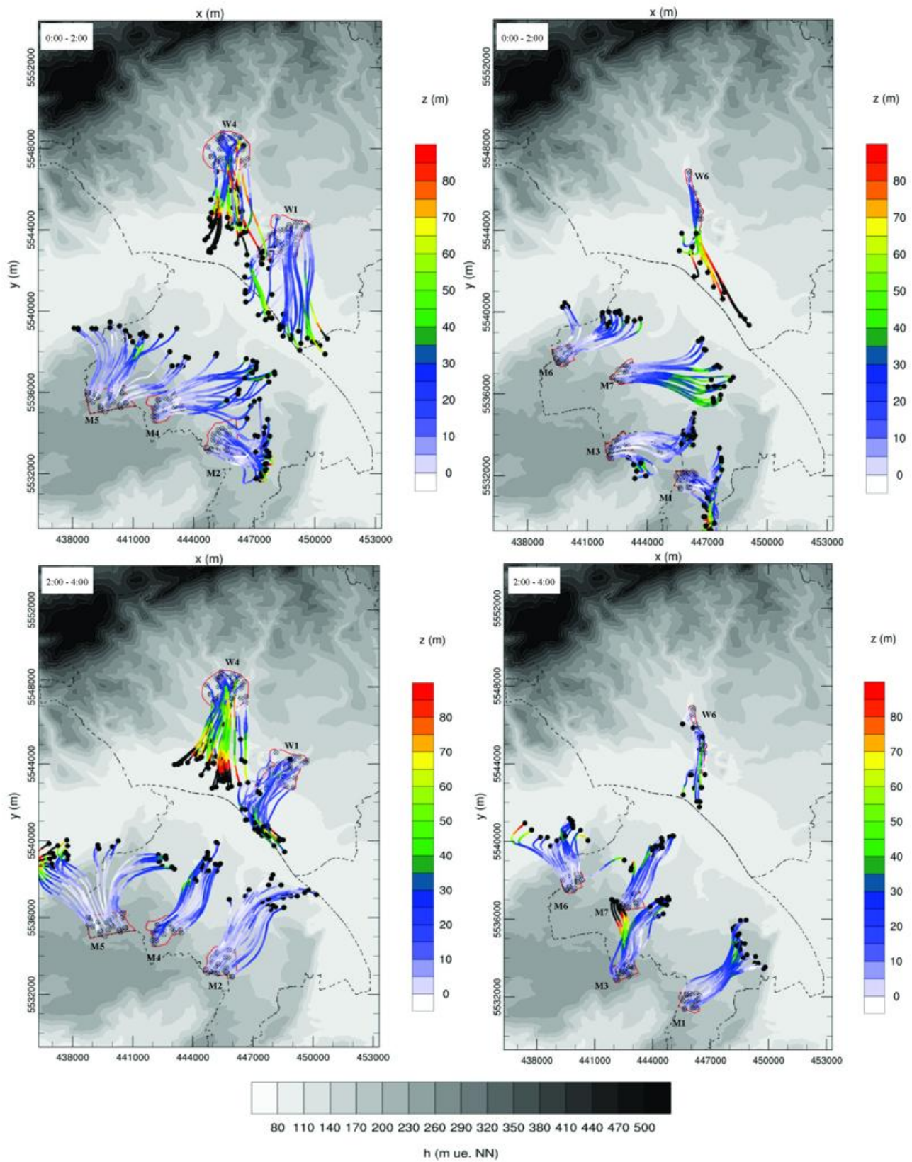
Abbildung 8-4: Vorwärtstrajektorien mit Startpunkt \otimes und Endpunkt \bullet . Die Farbe gibt die Höhe über Grund an, die dünneren roten Linien die Umrisse der Quellgebiete. Schwarz strichliert: Stadtgrenze. Links: Quellgebietsgruppe Q_{gr} , rechts: Q_{kl} . Oben: Start um 0 MESZ, Ende um 2 MESZ, unten: Start um 2 MESZ, Ende um 4 MESZ.
