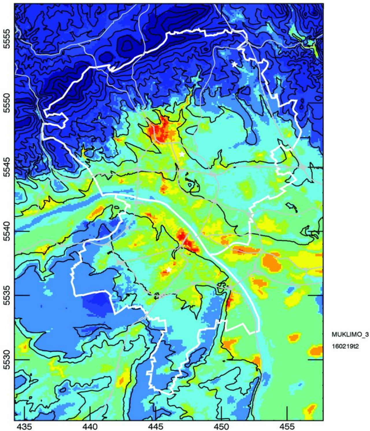
Abbildung 6-2: wie Abbildung 6-1, aber für heiße Tage.
