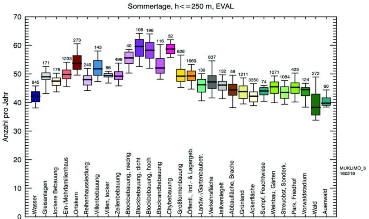
Abbildung 6-4: Box-Whisker-Plots für jede Landnutzungsclass 1971-2000 (EVAL) für die mittlere jährliche Anzahl an Sommertagen. Berücksichtigt wurden nur die innerhalb der beiden Stadtgebiete und unter 250 m ü. NN gelegenen Gitterzellen. Die Zahlen über den Box-Whiskers geben die Anzahl der ausgewerteten Gitterzellen der jeweiligen Klasse an.
