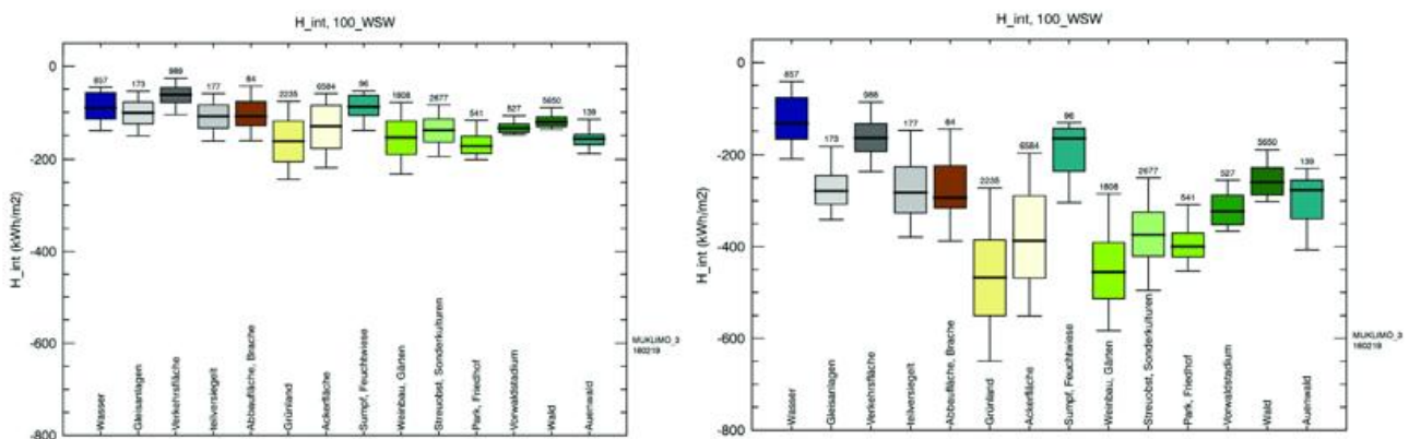
Abbildung 8-2: Box-Whisker-Plots des zeitlich aufintegrierten fühlbaren Wärmestroms vom Untergrund und den Bäumen in Abhängigkeit von der Landnutzungsklasse. Links: 22 bis 00 MESZ, rechts: 22 bis 04 MESZ,
