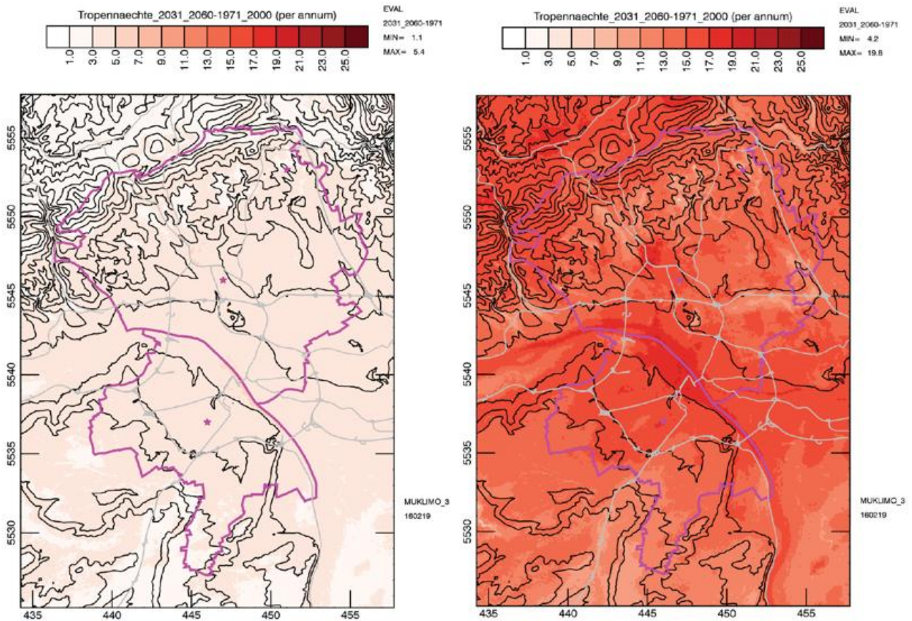
Abbildung 7-6: wie Abbildung 7-4, aber für die Tropennächte.
