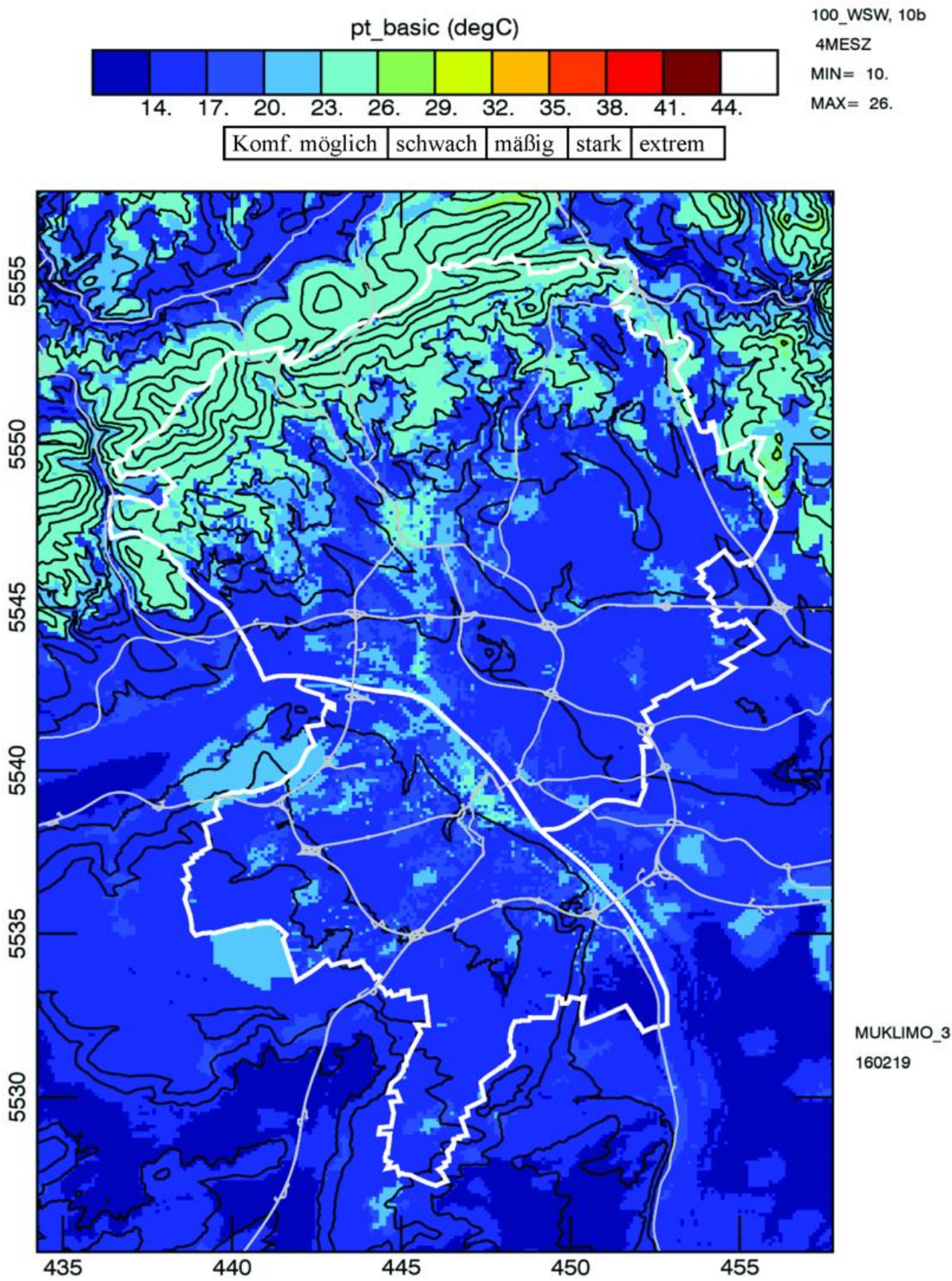
Abbildung 5-6: Wie Abbildung 5-4, aber für 4 MESZ.
