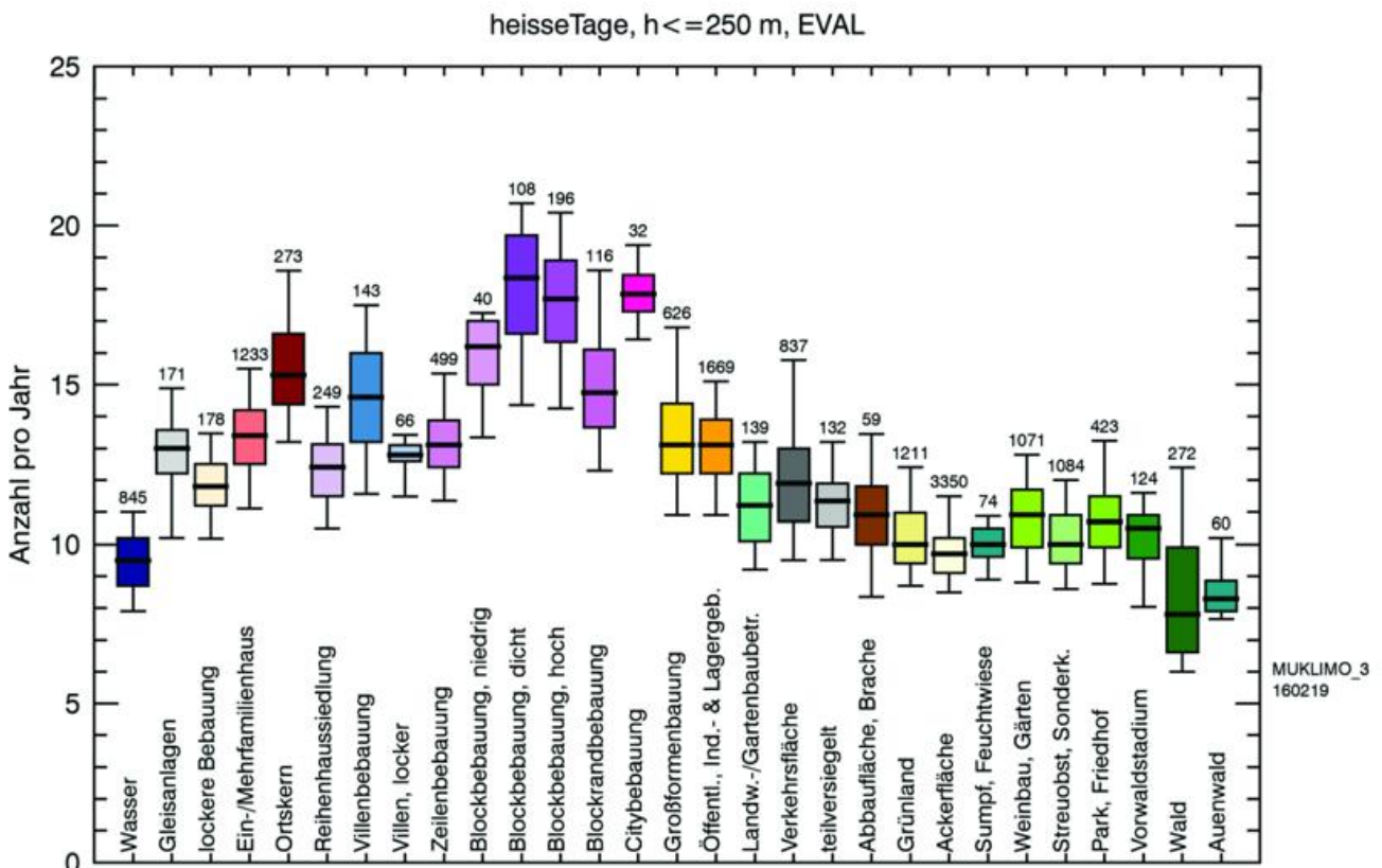
Abbildung 6-5: Wie Abbildung 6-4, aber für heiße Tage
