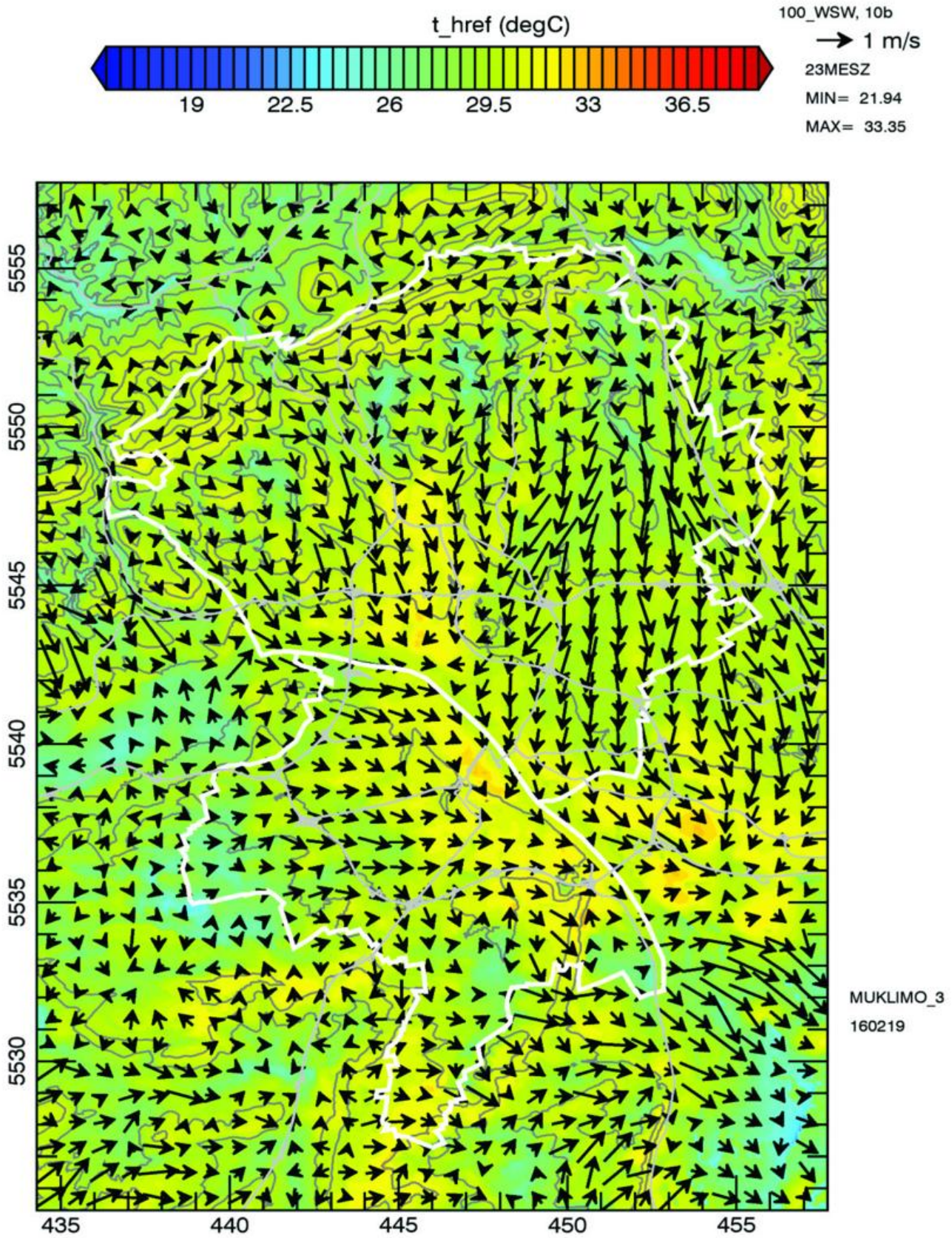
Abbildung 5-2: Wie Abbildung 5-1, aber für 23 MESZ.
