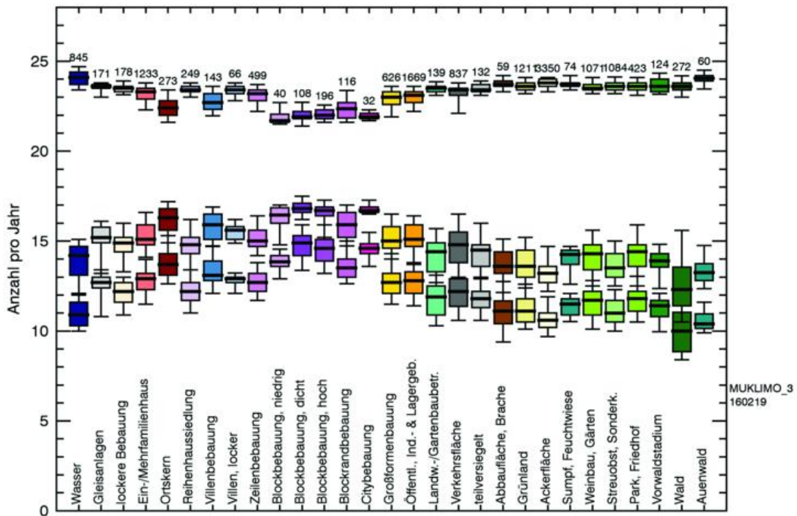
Abbildung 7-7: Box-Whisker-Plots für die projizierte Änderung der Anzahl der Sommertage in Abhängigkeit von der Landnutzungsklasse. Untere Reihe: 25. Perzentil der Änderung, Mitte: Median, obere Reihe: 75. Perzentil. Berücksichtigt wurden nur die innerhalb der beiden Stadtgebiete und unter 250 m ü. NN gelegenen Gitterzellen.
