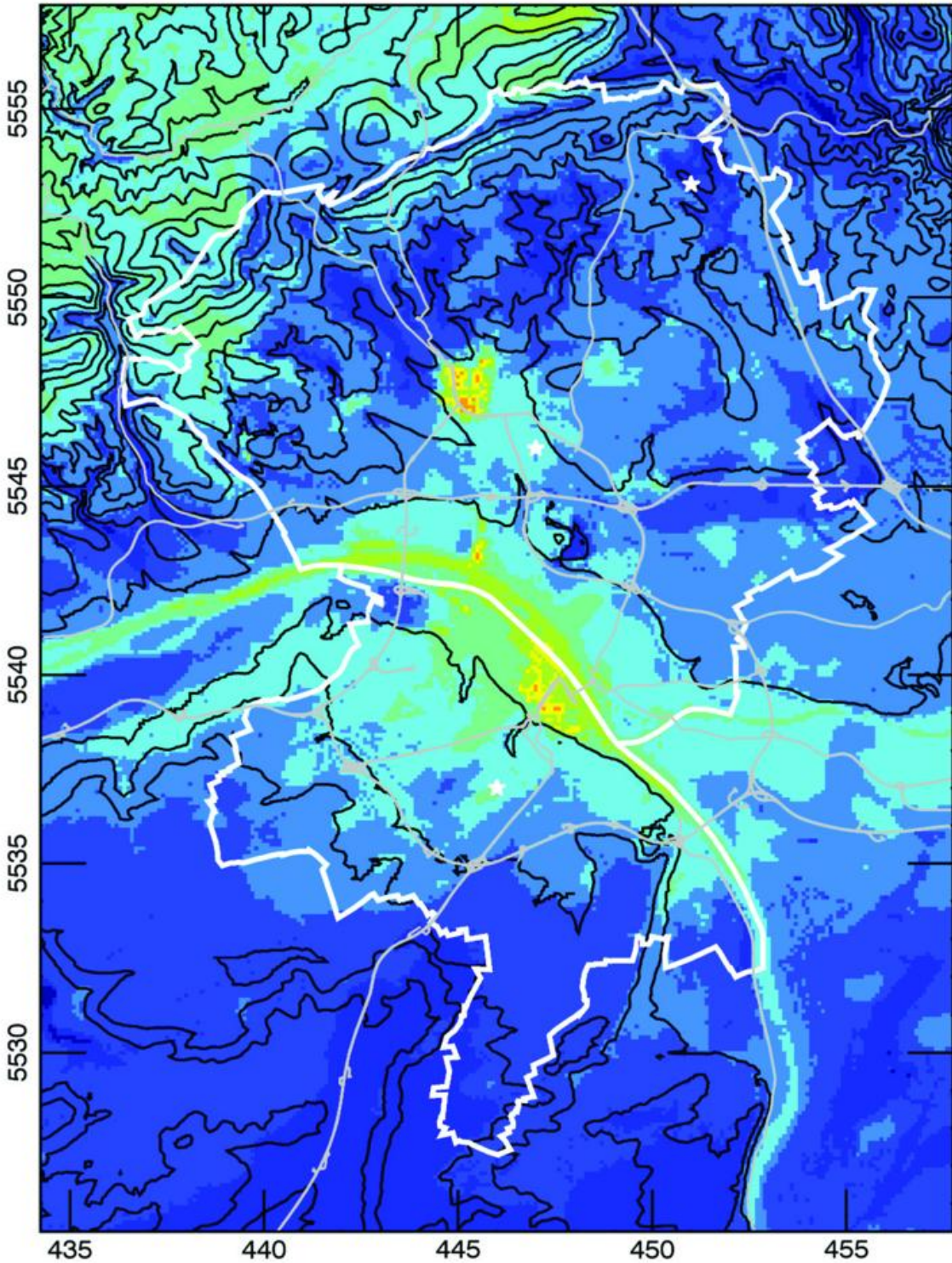
Abbildung 6-3: Wie Abbildung 6-1, aber für Tropennächte.
