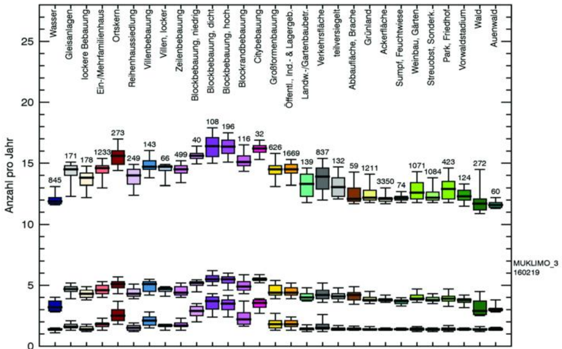
Abbildung 7-8: wie Abbildung 7-7, aber für die heißen Tage.
