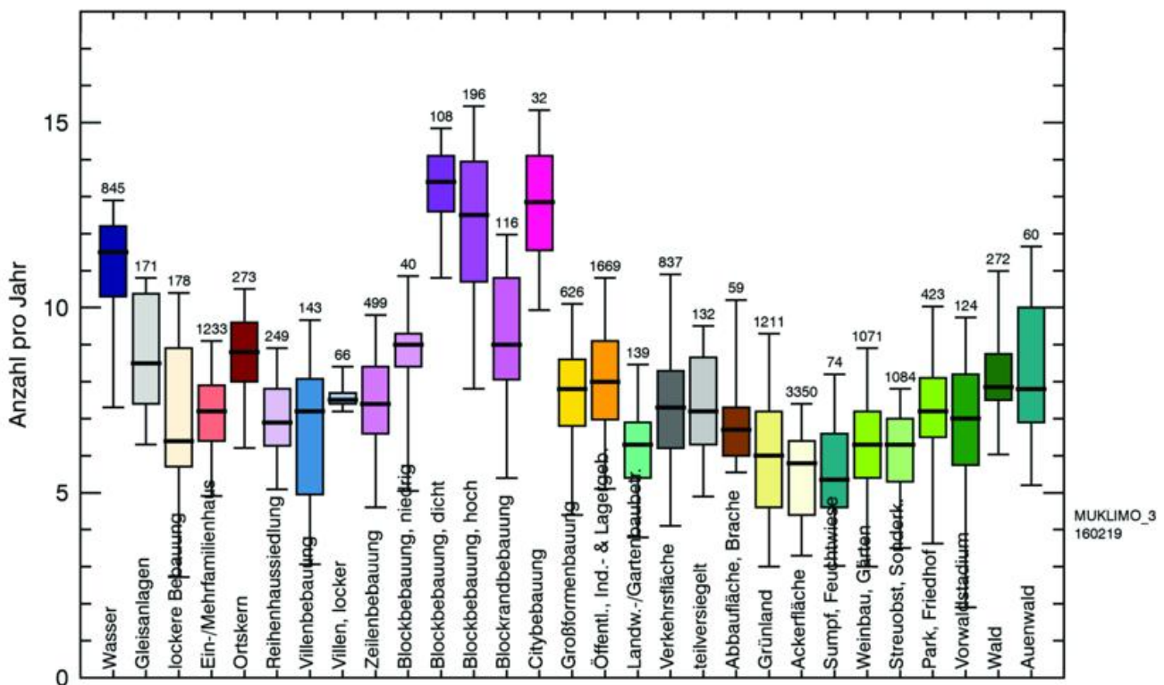
Abbildung 6-6: Wie Abbildung 6-4, aber für Tropennaechte
