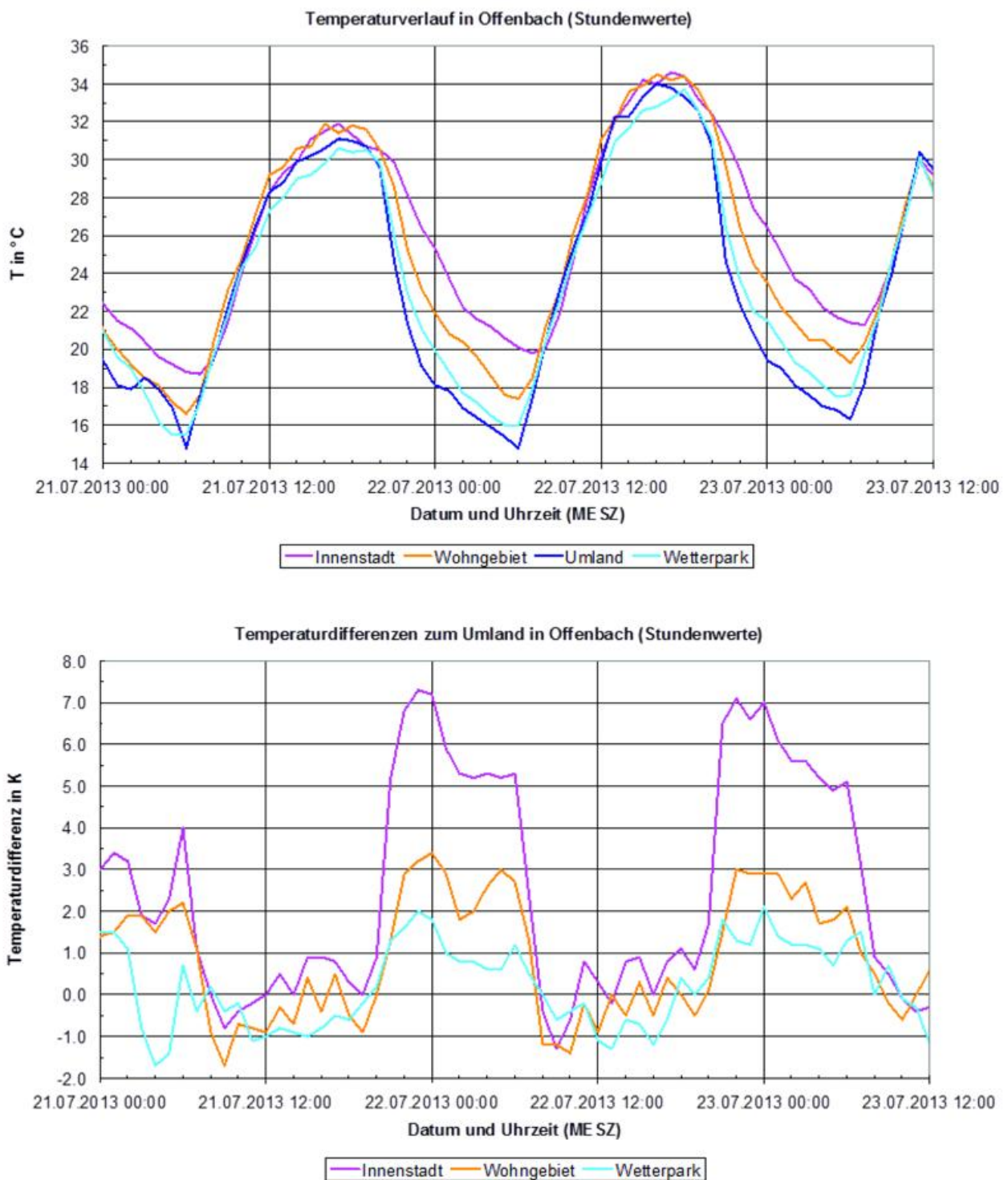
Abbildung A-1: Tagesgang der Lufttemperatur (oben) und der Temperaturdifferenz zum Umland (unten) in Offenbach für eine Schönwetterperiode (21.07.2013 bis 23.07.2013) aus Stundenwerten (Quelle: DWD).
