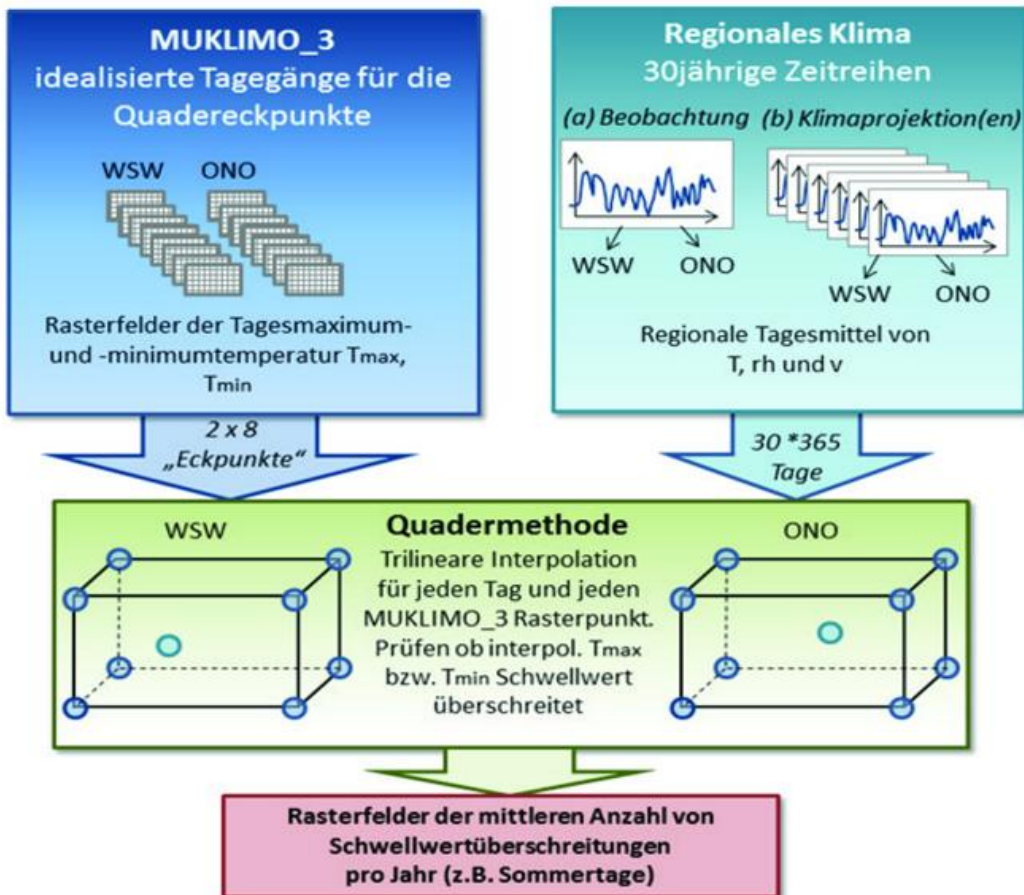
Abbildung B-3: Skizze der Arbeitsschritte zur Berechnung der räumlich hoch aufgelösten mittleren jährlichen Anzahl an Kenntagen (z. B. Sommertagen) in einer Stadt, beispielhaft für die zwei Hauptwindrichtungen WSW und ONO.
