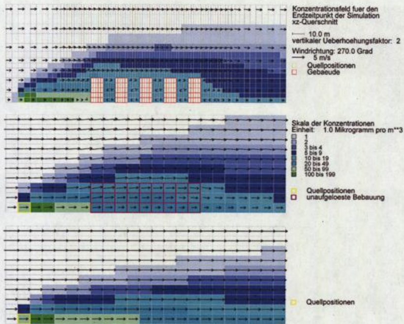
Abbildung 5.16: Resultate für den Wind und die Konzentration einer Luftbeimengung für die aufgelöste (a) und unaufgelöste (b) Modellierung eines Ensembles von 25 kubischen Blöcken. Das Resultat (c) gehört zu einer Vergleichssimulation mit fehlender Bebauung. Die Abbildung zeigt zentrale Querschnitte des Modellgebiets.
