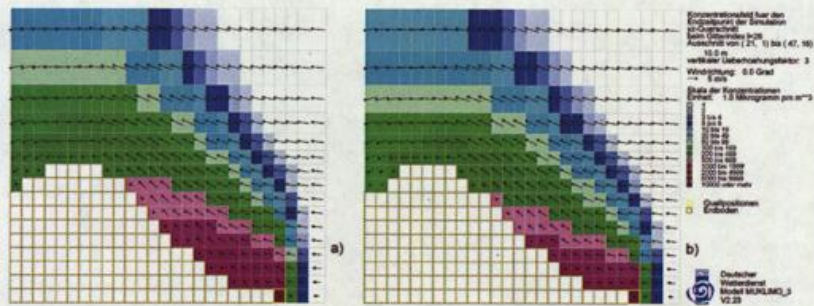
Abbildung 5.20: Modellbeispiel „Gaussberg“. Gezeigt ist ein Resultsvergleich für unterschiedliche Modellierungen der Orographie, zum einen als blockförmiges Gelände (a) und zum anderen vermittelt einer Höhen-Rasterdatei (b).
