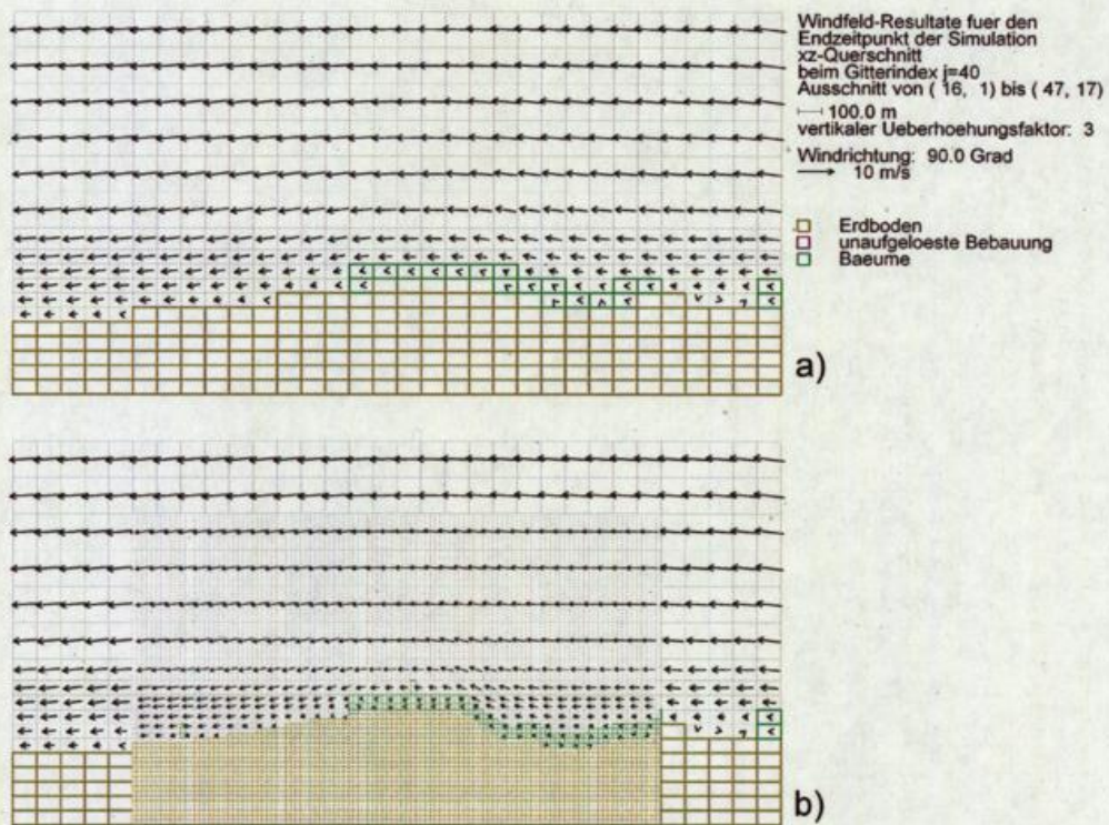
Abbildung 5.22: Modellbeispiel „Weinbaugbiet“. Der Teil a) zeigt Resultate des „umfassenden“ Modells für das Gesamtgebiet im Ausschnitt. In b) sind in dieselbe Abbildung Resultate für den Kernbereich des „verfeinerten“ Modells für das „Teilgebiet“ eingeblendet.
