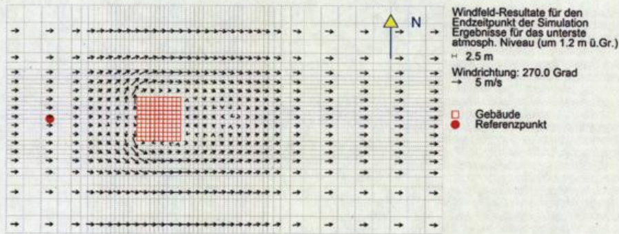
Abbildung B.2: Validierungsrechnungen. Resultate zur Gebäudeumströmung (Testfall a3-1).
