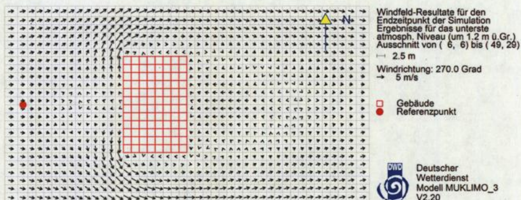
Abbildung B.7: Validierungsrechnungen. Anströmung eines „breiten“ Gebäudes mit einer Grundfläche von 30 \times 20 \text{ m}^2 bei einer Höhe von 25 m (Testfall c5).
