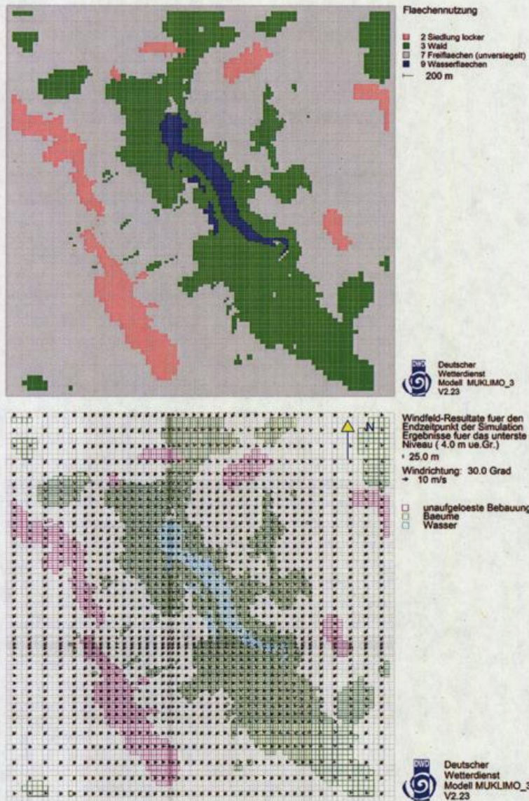
Abbildung 5.23: Modellbeispiel zum Landnutzungsklassenmodus. Oben flächennutzung, unten Resultat Windfeldsimulation.
