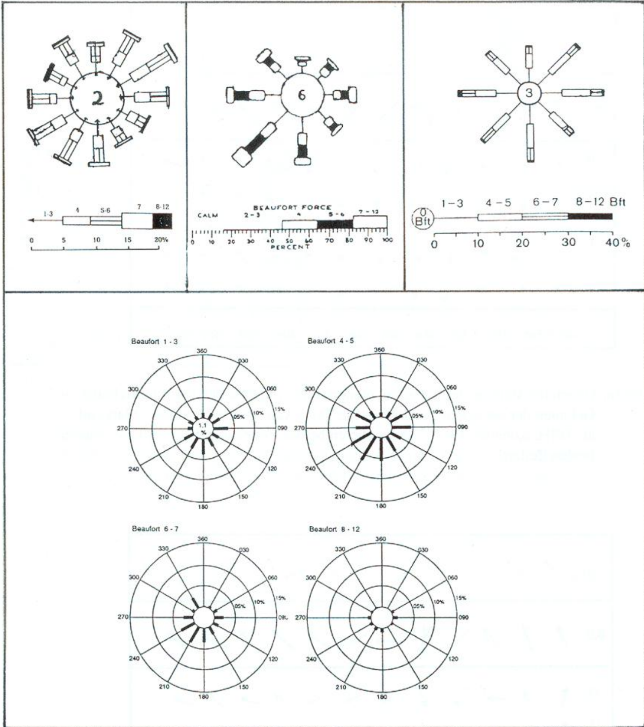
Abb.6a: Gegenüberstellung mittlerer Windrosen mit zugehörigen Skalen für die südliche Nordsee: im Februar nach Oilfield Publication (links oben) und BSH (rechts oben), im Januar nach Höhn (Mitte oben) und Korevaar (unten).
