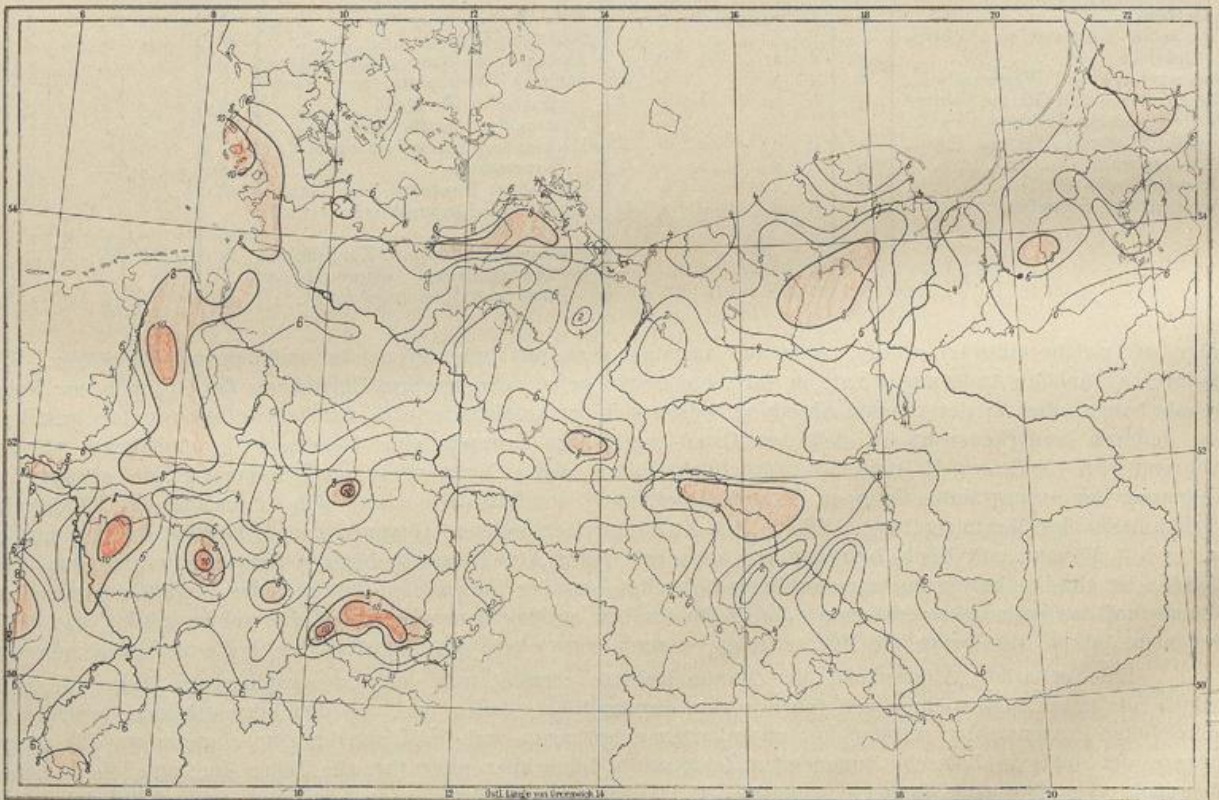
Fig. 3. Mittlere jährliche Häufigkeit der Gewitter mit Hagel- oder Graupelfällen in Prozenten der Gesamtzahl der Gewitter.
