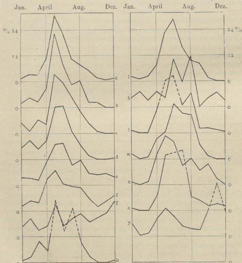
Fig. 2. Typen der jährlichen Verteilung der Gewitter mit Hagel- und Graupelfällen.
