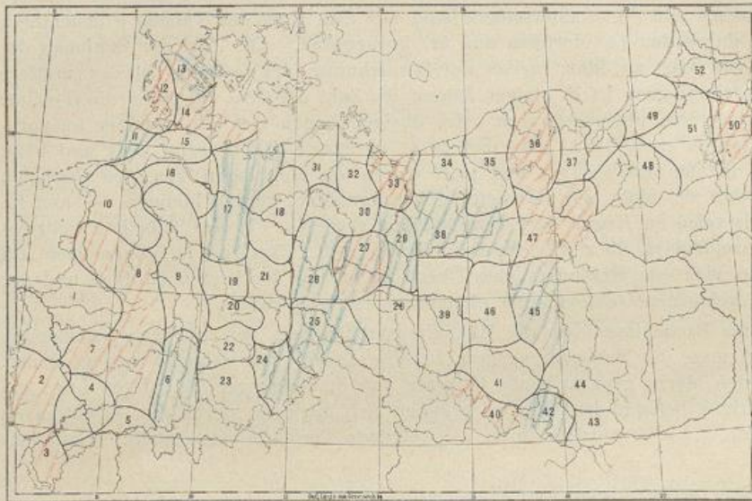
Fig. 1. Gruppierung der Stationen auf Grund der Übereinstimmung der jährlichen Verteilung der Gewittertage.
