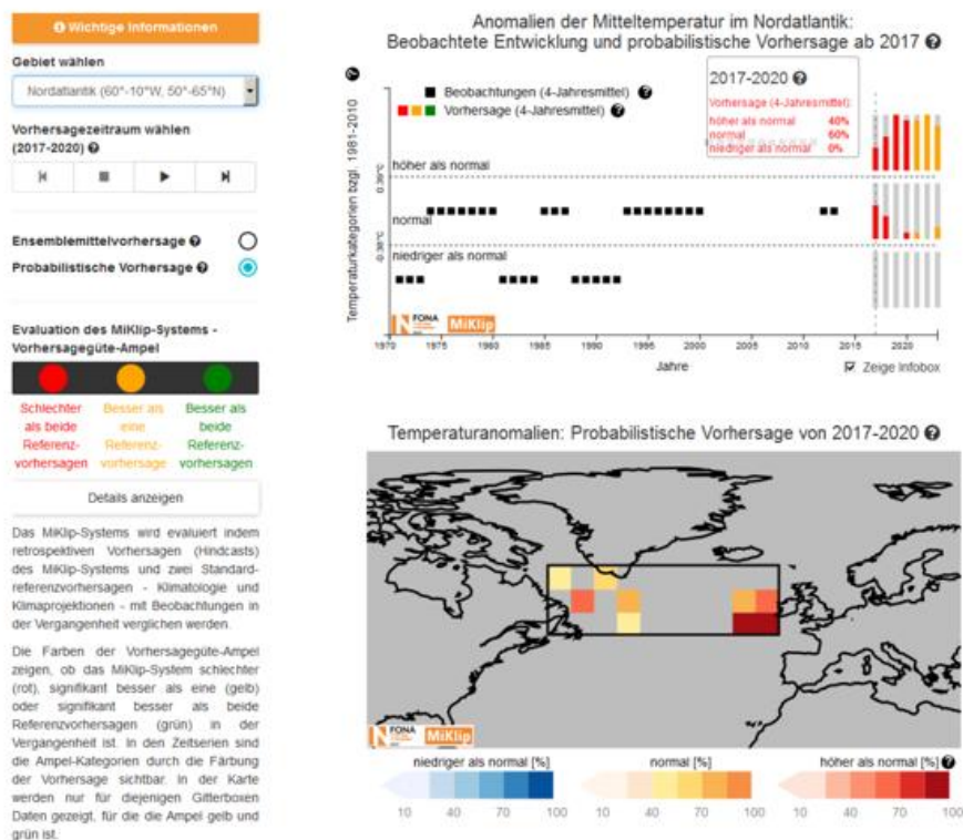
Abb. 2: Probabilistische Vorhersage der Ensemble-Verteilung von MPI-ESM-LR für die Mitteltemperatur im Nordatlantik im Vergleich zu Beobachtungen von HadCRUT (Quelle: MiKlip-Webseite).
