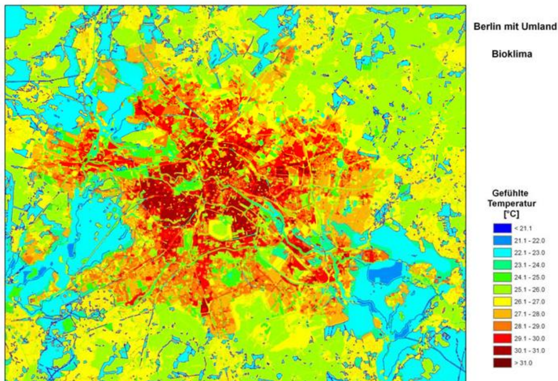
Karte 5 Gefühlte Temperatur in °C an einem windschwachen, wolkenlosen Sommertag nachmittags in Berlin und Umland
