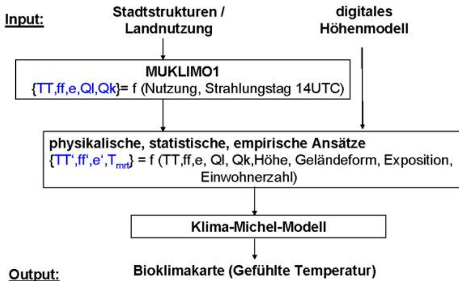
Abbildung 3: Schematischer Aufbau des Stadtbioklimamodells UBIKLIM (TT: Lufttemperatur, ff: Windgeschwindigkeit, e: Feuchte, Ql: langwellige Strahlungsflüsse, Qk: kurzwellige Strahlungsflüsse, T_{mrt} : mittlere Strahlungstemperatur des Menschen, Werte für 1 m über Grund)
