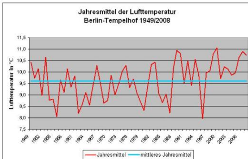
Abbildung 1: Jahresmittel der Lufttemperatur an der Station Berlin-Tempelhof (1949-2008)
