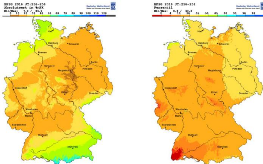
Abbildung 3: Wassergehalte in Prozent nutzbarer Feldkapazität (%nFK) unter Gras (Sandböden) für den 12.9.2016 (links) sowie Perzentil-Verteilung auf Basis der Zeitreihe 1961-2016 (rechts).
