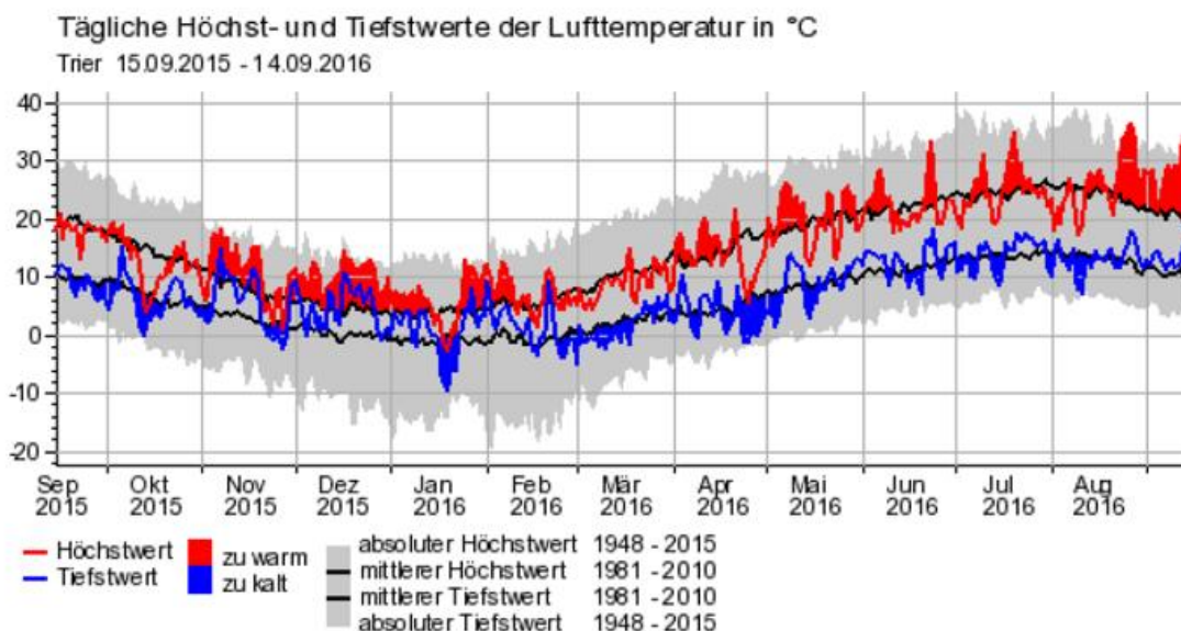
Abbildung 1: Tägliche Höchst und Tiefstwerte der Lufttemperatur in °C für Trier ( link ).
