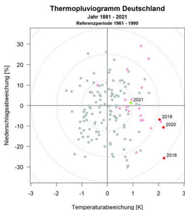
▲ Abweichungen der Jahresmitteltemperatur und der Jahresniederschlagssumme vom Mittelwert der Referenzperiode 1961-1990. Die grauen Punkte symbolisieren die Jahre vor der letzten Jahrtausendwende und die roten Punkte die letzten 21 Jahre.
