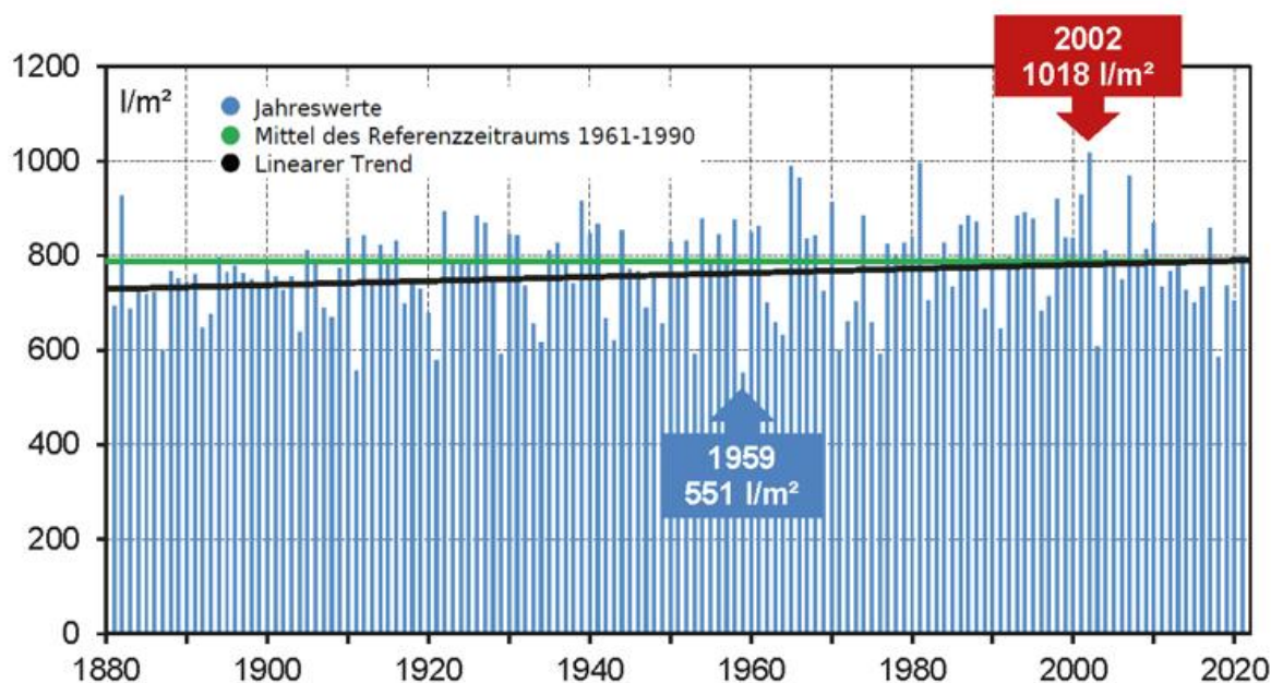
▲ Es ist nasser geworden in Deutschland: Zeitreihe der Jahresniederschlagshöhen (Flächenmittel aus Stationsmessungen) von 1881 bis 2021.
