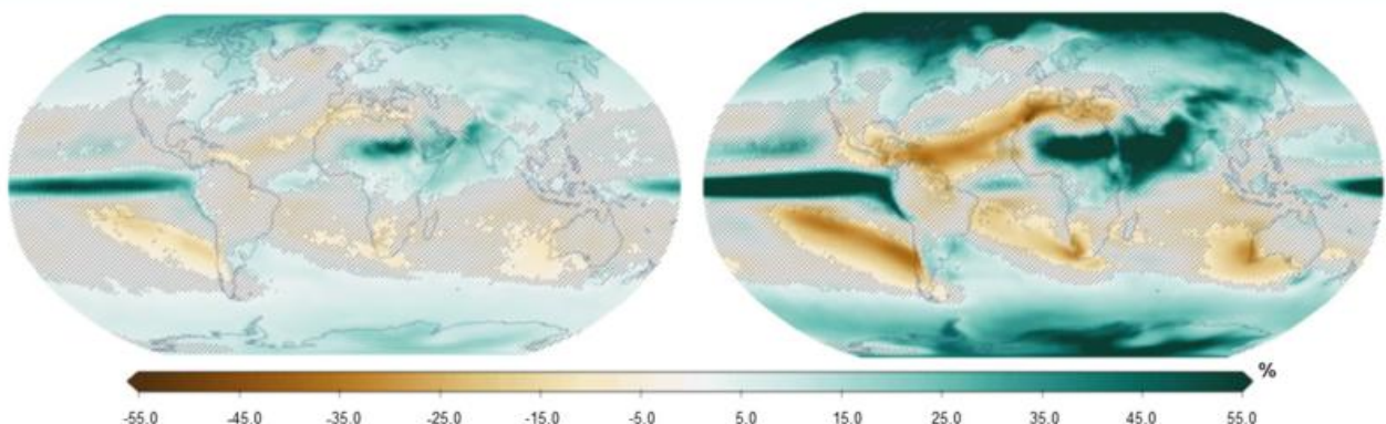
▲ Mittlere Niederschlagsänderung für den Zeitraum 2081–2100 auf der Basis des SSP1-2.6 (links) und des SSP5-8.5 (rechts) Szenarios. Dargestellt ist der Unterschied zum Zeitraum 1961–1990. Die Schraffur zeigt Regionen, in denen der gezeigte Änderungswert kleiner als die natürliche Klimavariabilität ist. (Quelle: https://interactive-atlas.ipcc.ch )
