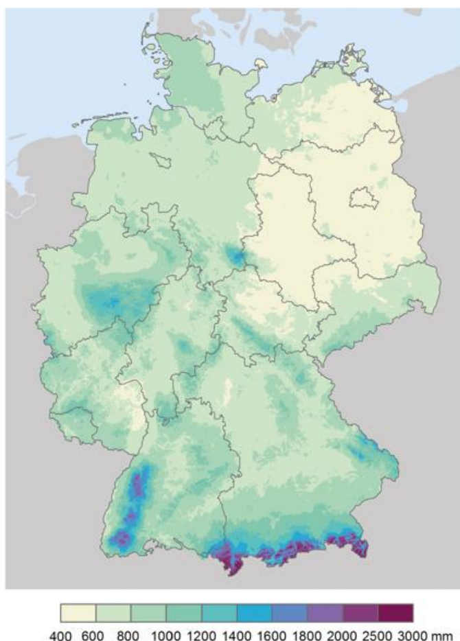
▲ Jährliche Niederschlagshöhe in Deutschland im Referenzzeitraum 1961–1990 als Flächendarstellung der Rasterwerte ( 1 \text{ km} \times 1 \text{ km} ).
