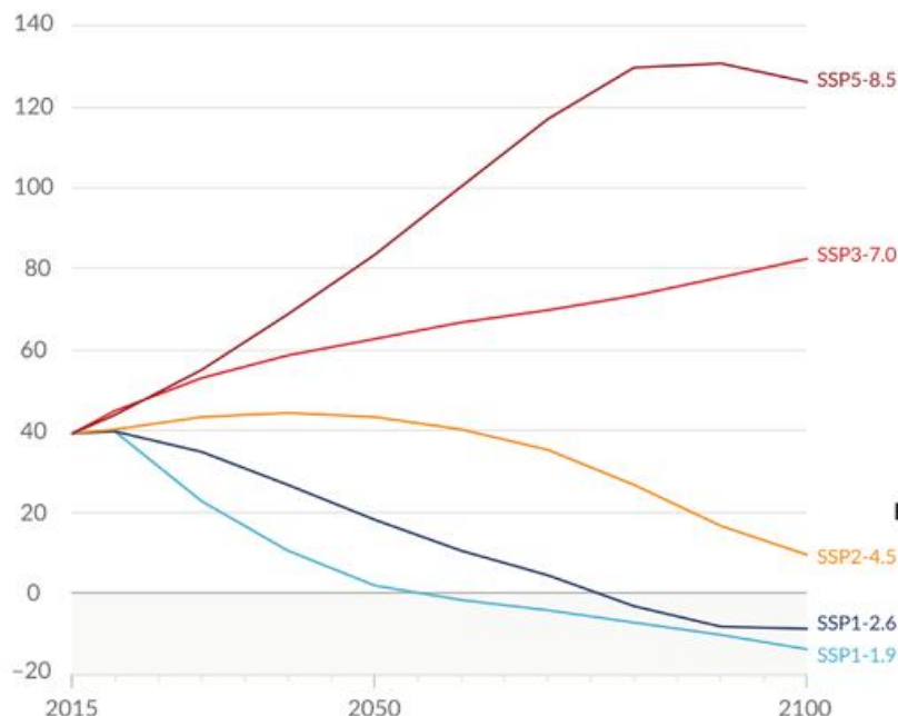
Kohlendioxid (Gt CO 2 / Jahr)
