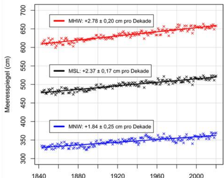
Mittlerer relativer Meeresspiegel (MSL), ► Hochwasser- (MHW) und Niedrigwasserscheitel (MLW) am Pegel Cuxhaven als Jahresmittel für 1843-2020. Trendangaben in cm/Dekade mit 95% Konfidenzintervall. (Quelle: Bundesamt für Seeschifffahrt und Hydrographie; Rohdaten: WSA Cuxhaven)
