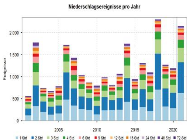
▲ Jährliche Anzahl extremer Niederschlagsereignisse in Deutschland für verschiedene charakteristische Dauerstufen. Datenbasis für die Jahre 2001 bis 2020 ist der klimatologisch aufbereitete Datensatz RADKLIM_V2017.002. Die (vorläufigen) Daten für 2021 basieren auf den Echtzeitanalysen aus RADOLAN.
