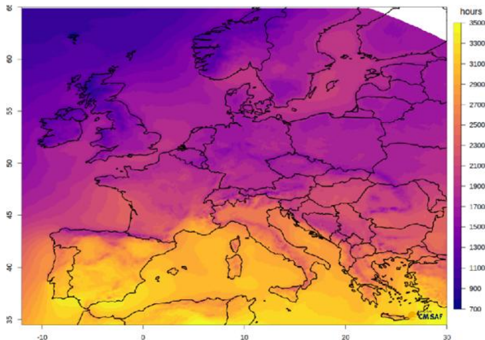
Abbildung 2: Räumliche Verteilung der klimatologischen Sonnenscheindauer basierend auf SARA3-Daten von 1991 bis 2020
