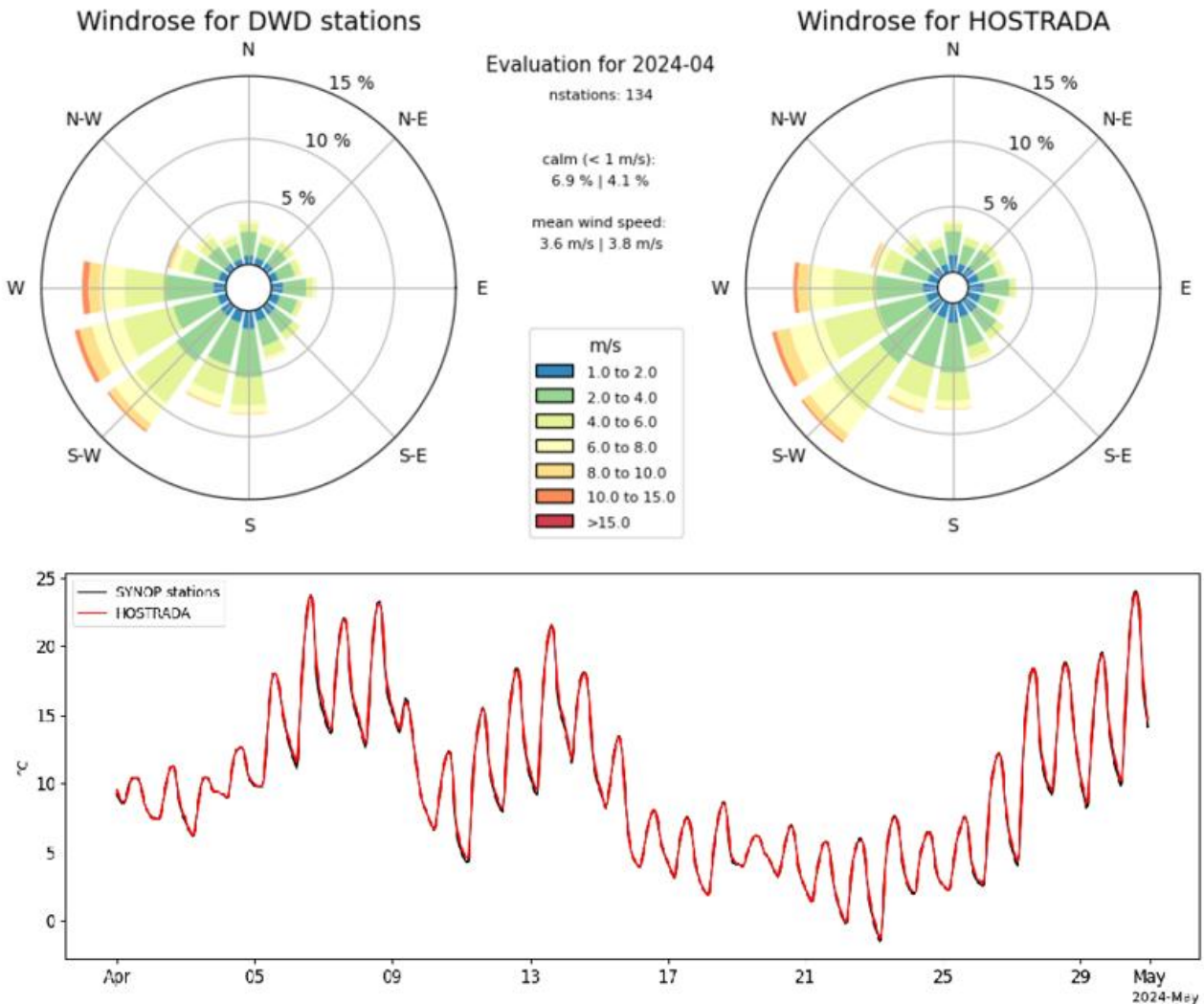
Abbildungen: Vergleich der Temperaturzeitreihe und Windstatistiken für April 2024 aus dem Messnetz des DWD (420 Messstandorte der Lufttemperatur in 2m Höhe, 134 Messstandorte der Windrichtung und -geschwindigkeit in 10m Höhe; oben) mit den korrespondierenden Rasterpunkten im Datensatz HOSTRADA (unten).
