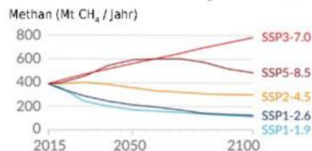
Ausgewählte Beiträge von Nicht-CO 2 -Treibhausgasen
