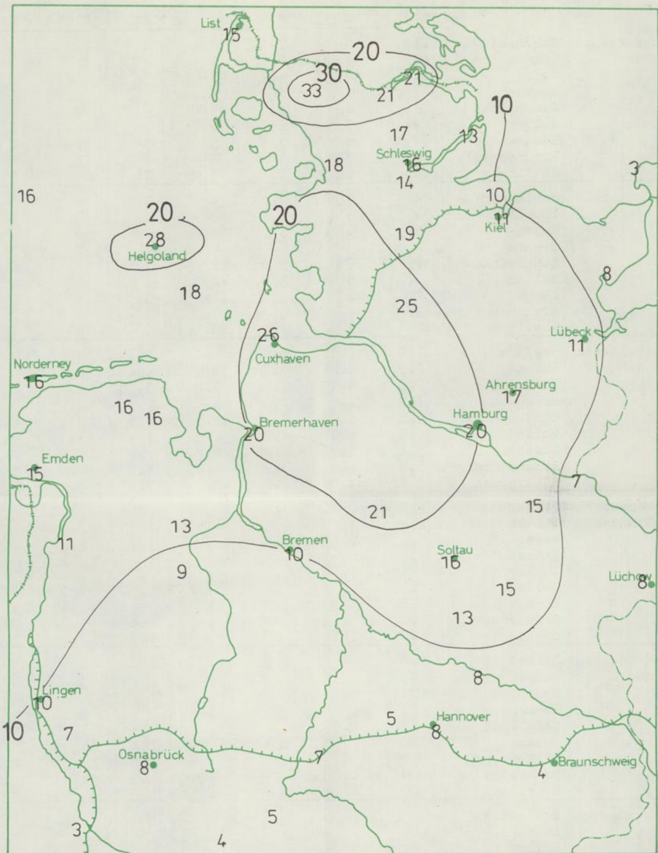
Wochensummen des Niederschlags in mm vom 28.10. - 03.11.1985
