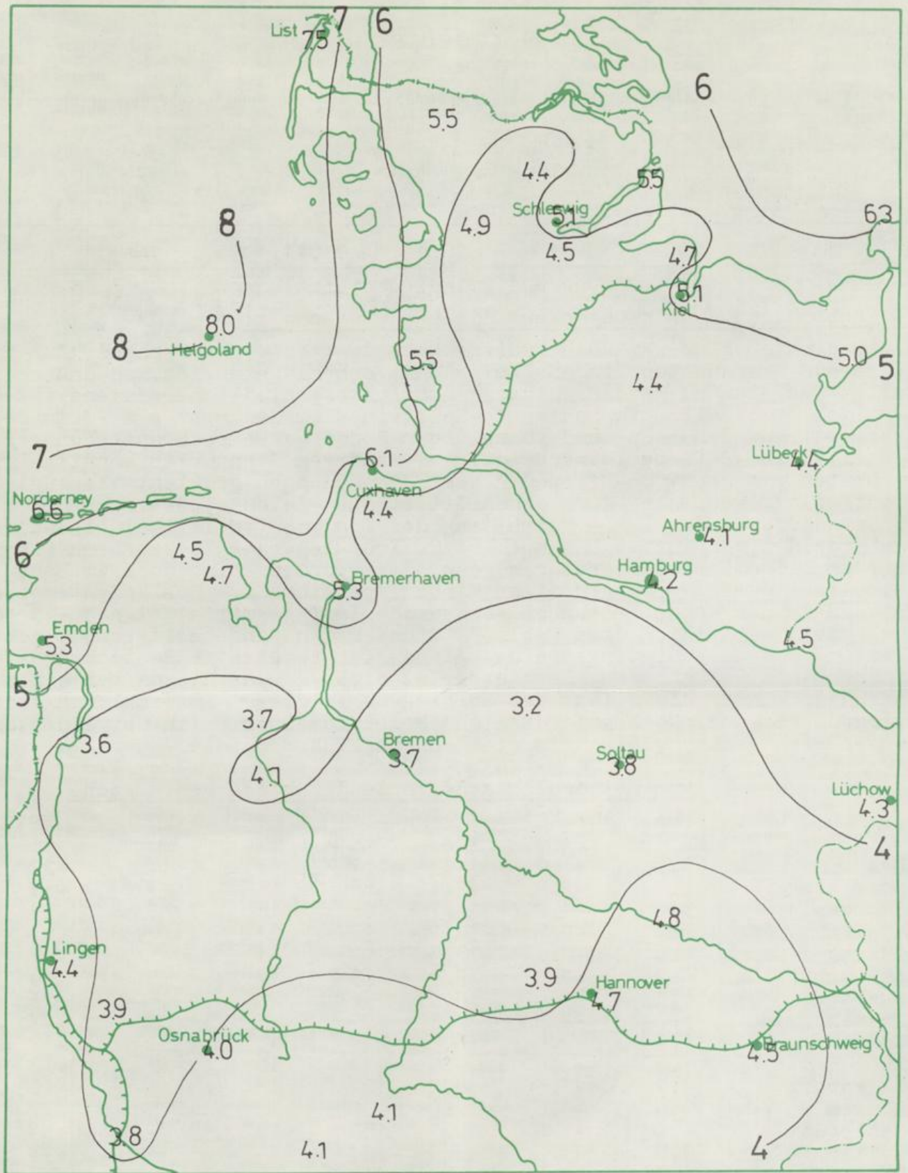
Wochenmittel der Lufttemperatur in °C vom 28.10. - 03.11.1985
