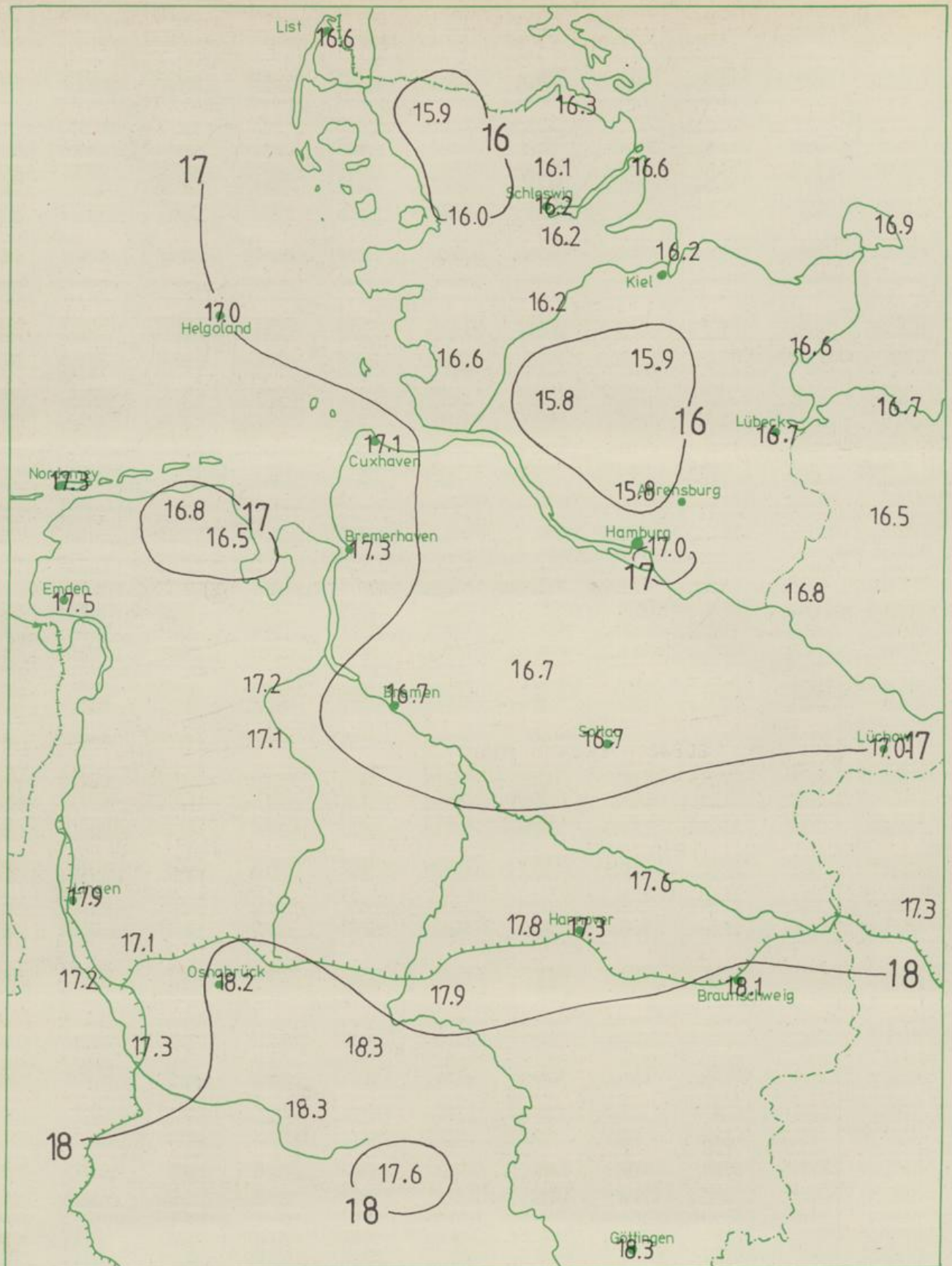
Wochenmittel der Lufttemperatur in °C vom 06.08. bis 12.08.1990
