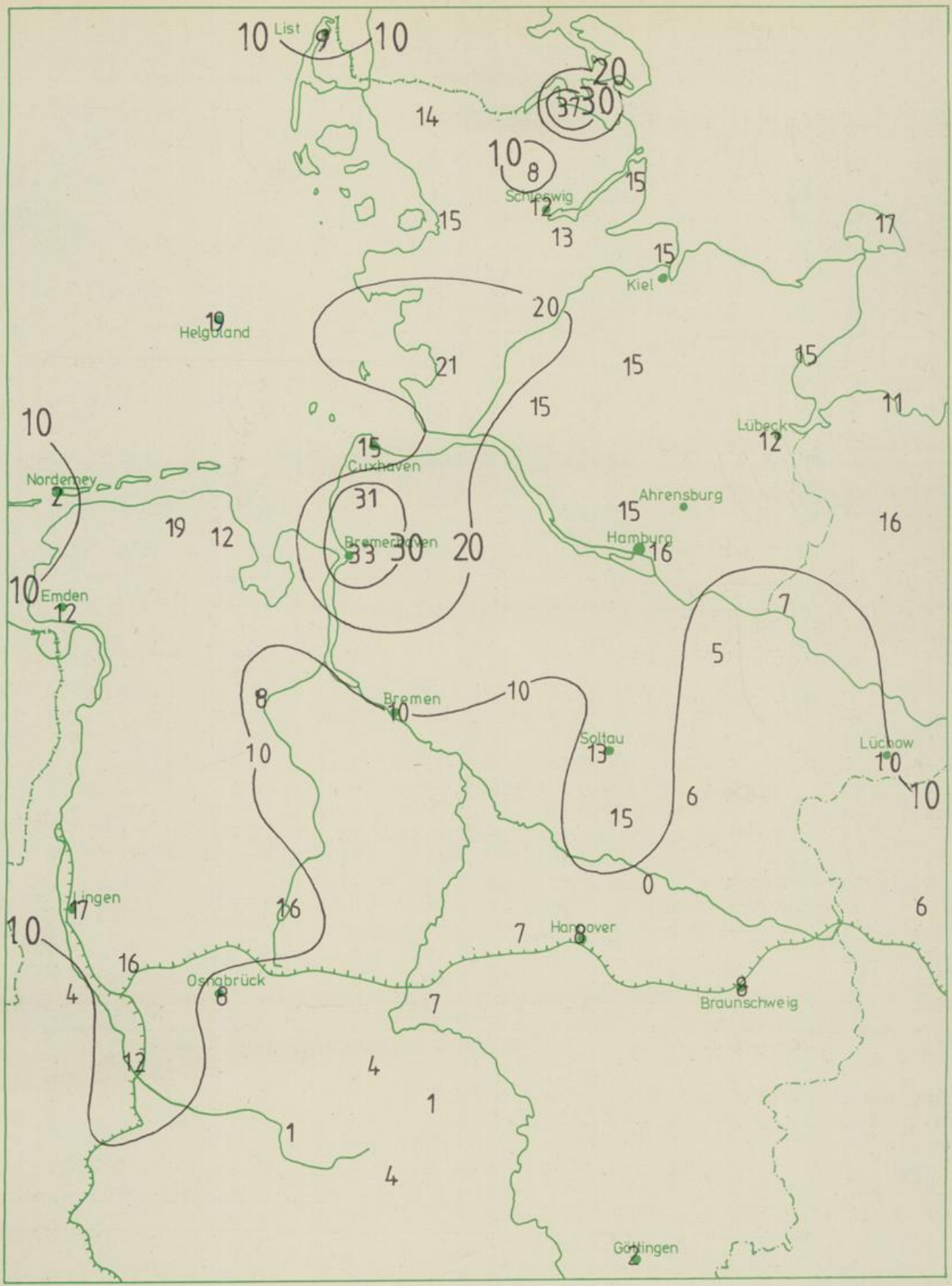
Wochensummen des Niederschlags in mm vom 06.08. bis 12.08.1990
