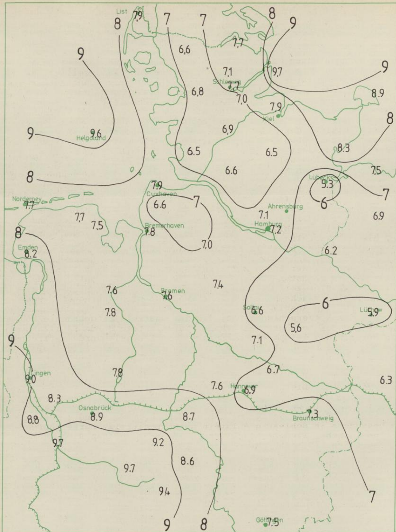
Wochenmittel der Lufttemperatur in °C vom 22.10. bis 28.10.1990
