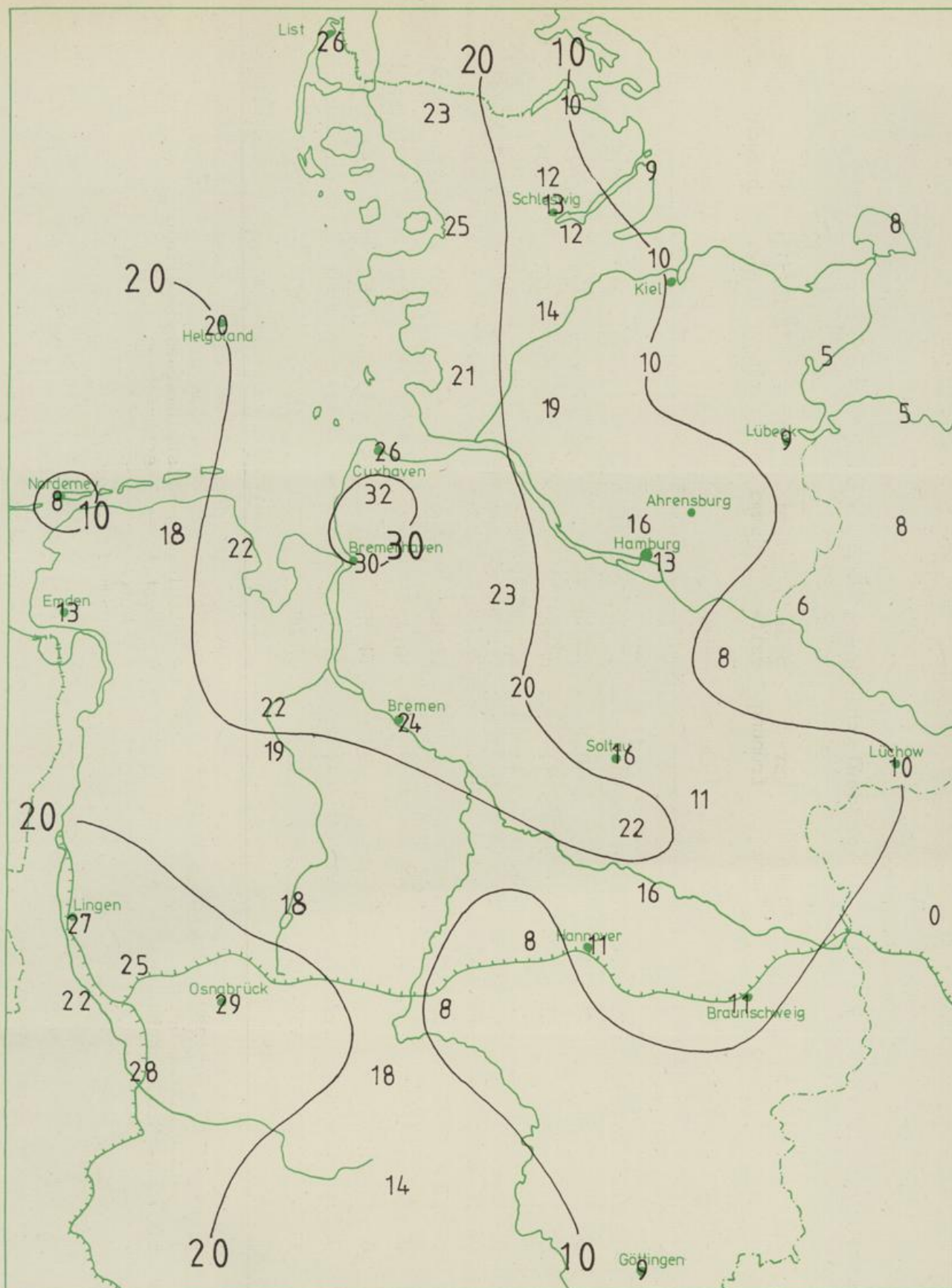
Wochensummen des Niederschlags in mm vom 22.10. bis 28.10.1990
