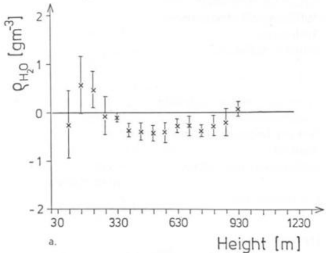
Abb. 8: Mittelwert und seine Streuung einer 10 min Testmessung mit beiden Lasern on line, zu der Messung aus Abbildung 5.
