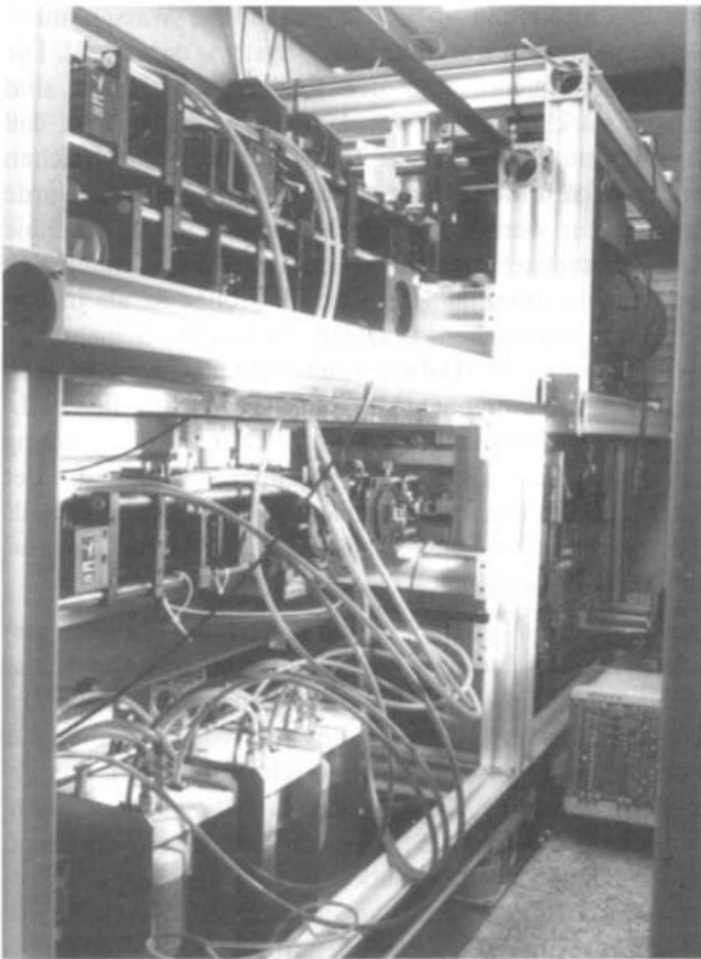
Abb. 3: Teilansicht Differential-Absorption-Lidar-System.
