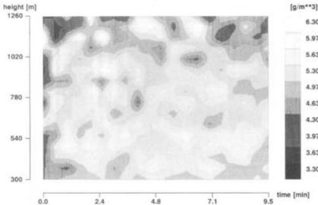
Abb. 4: Wasserdampfdichte, Messung vom 12. Juni 1986, 16 h 30, Mittelwert über 300 Schuß (30 sec), Höhengauflösung 60 m (Signalglätte über 120 m).
