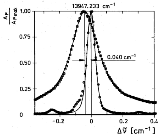
Abb. 1: Photoakustische Spektren der Wasserdampfabsorptionslinie 13947.233 \text{ cm}^{-1} . \circ : Zelle gefüllt mit 16 hPa \text{H}_2\text{O} , \square : Zelle gefüllt mit 16 hPa \text{H}_2\text{O} und 1000 hPa synthetischer Luft.
