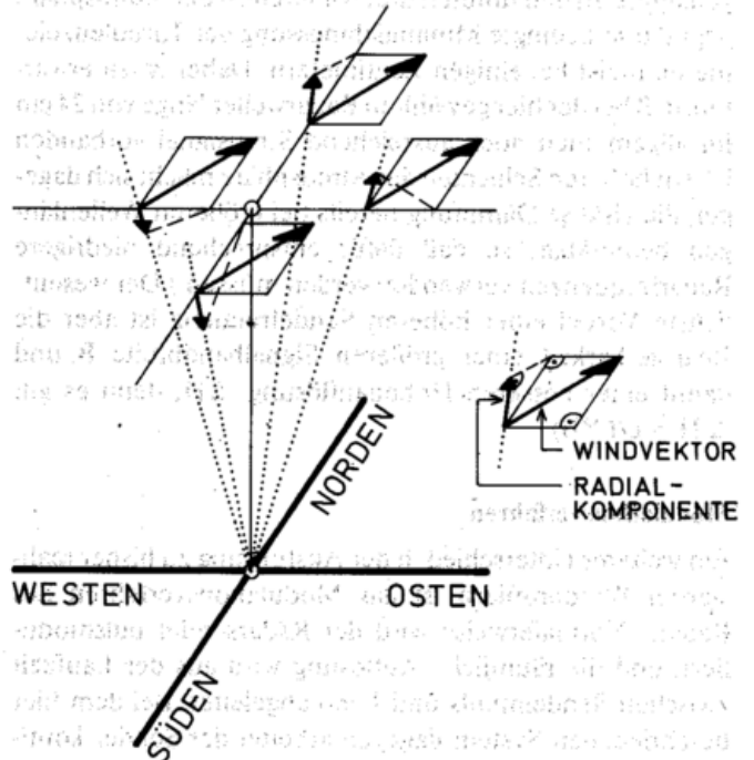
Abb. 1: Typische Strahlanordnung eines Windprofilers.
