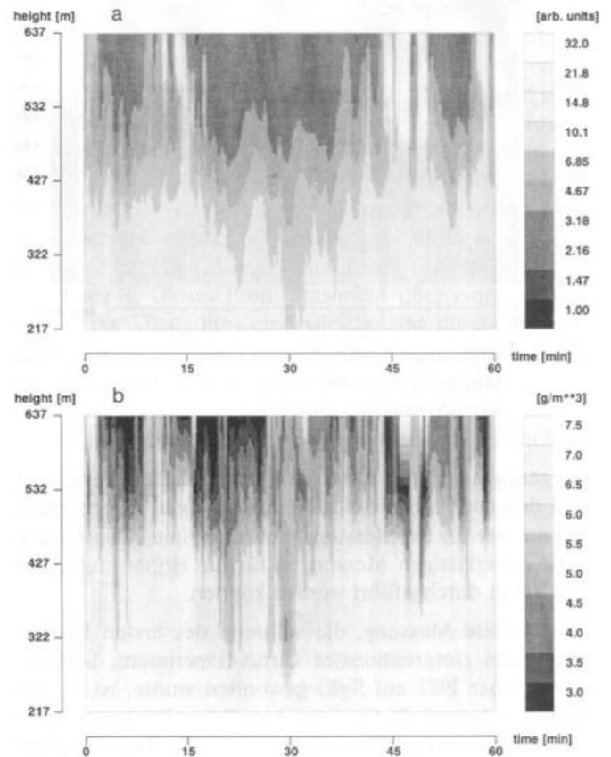
Abb. 9: Stärke des Rückstreusignals in willkürlichen Einheiten und Wasserdampfkonzentration aus Messungen am 18. September 1987, 14.00 GMT, Auflösung 75 m, 25 sec, Signalglättung 150 m.
