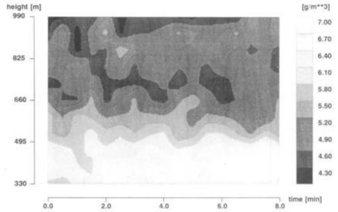
Abb. 5: Wasserdampfdichte, Messung vom 11. Juni 1986, 21 h 40, Mittelwert über 300 Schuß (30 sec), Höhengauflösung 60 m (Signalglätte über 120 m).
