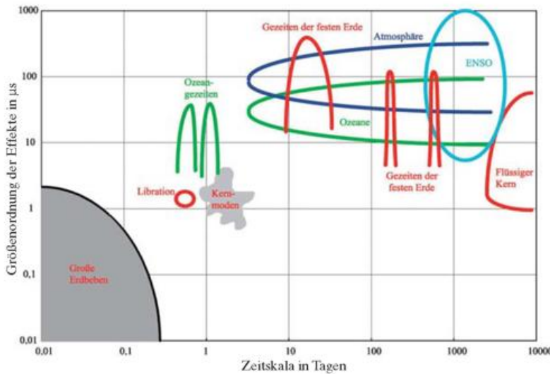
Abb. 2: Einflüsse auf die Weltzeit UT1 - Größenordnungen und Zeitskalen in logarithmischer Achskalierung (Quelle: ftp://gemini.gsfc.nasa.gov/pub/core/fig1.ps; modifiziert). Die Einflüsse der Atmosphäre und Ozeane wirken im Bereich von mehreren Tagen bis zu Dekaden. Für Perioden bis zu einem Jahr kommen Gezeiteneffekte der festen Erde und der Ozeane hinzu. Die wichtigsten Variationen der Weltzeit besitzen Perioden im jährlichen und halbjährlichen sowie im monatlichen und halbmonatlichen Bereich. Weiterhin gibt es signifikante dekadische Variationen. 1 \mu s als Zeiteinheit entspricht 15 \mu as als Winkleinheit.
