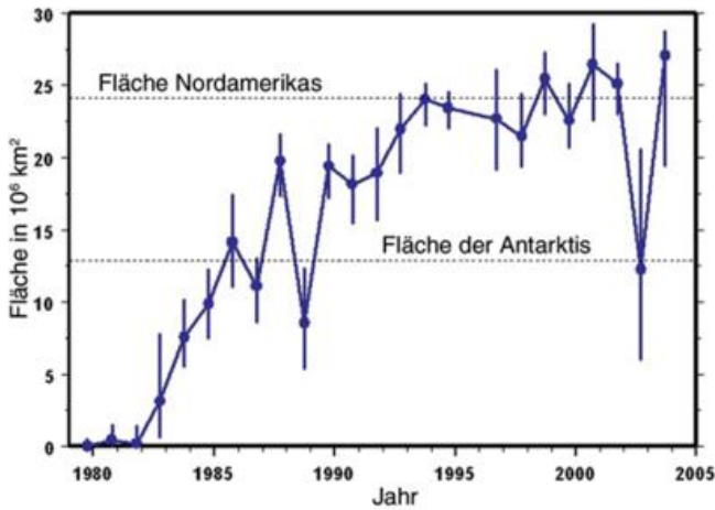
Abb. 23-3: Mittlere Ausdehnung des Ozonlochs (Gebiet mit < 220\text{ DU}</math>) von 1979 bis 2003. Schwankungen sind durch die Länge der vertikalen Linien gekennzeichnet. Zum Vergleich sind die geographischen Größen der Antarktis und des nordamerikanischen Kontinents angegeben. Variationen der vom Ozonloch bedeckten Fläche von Jahr zu Jahr resultieren insbesondere aus der Variabilität der großskaligen Dynamik in der Südhemisphäre. Beispielsweise ist die relativ geringe Ausdehnung im Jahr 2002 mit der Entwicklung einer außergewöhnlich starken planetaren Welle und einer davon ausgehenden Stratosphärenenerwärmung zu erklären. Quelle: NASA (2004, http://toms.gsfc.nasa.gov/index.html ).
