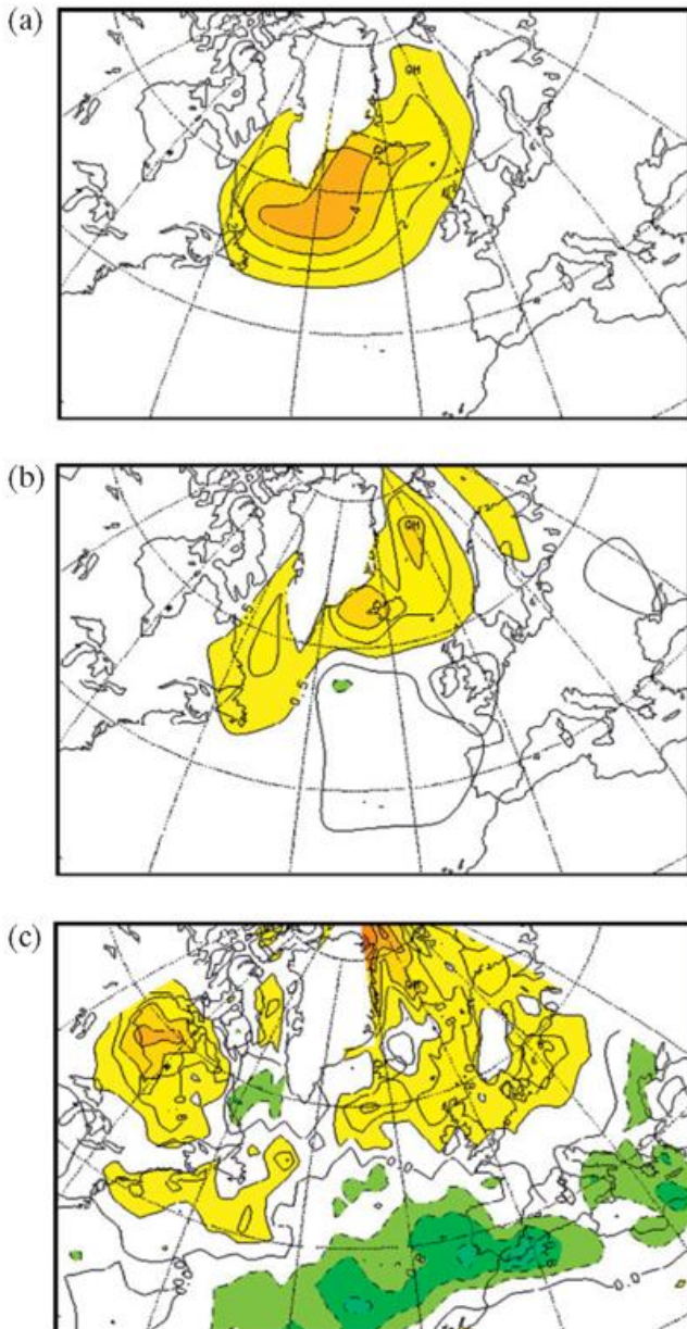
Abb. 22-5: (a) Zahl von extremen Zyklonen mit einem Kerndruck < 970 \text{ hPa} in den Wintermonaten (Dezember bis Februar) als Mittelwert über die Jahre 1980 bis 1990 im „Treibhausgasexperiment“, in dem \text{CO}_2 und andere Treibhausgase als Funktion der Zeit vorgegeben wurden. Die Zahlen charakterisieren die Häufigkeit des Auftretens von Extremzyklonen in Flächenelementen von jeweils 10^\circ \times 10^\circ . Der Abstand der Isolinien beträgt 1. (b) Änderung in der Häufigkeit von Extremzyklonen im gleichen Experiment zum Zeitpunkt der \text{CO}_2 -Verdoppelung (2060-2070). Der Abstand der Isolinien beträgt 0,5. (c) Änderung von Extremwindgeschwindigkeiten in 10 m Höhe in den Wintermonaten 2060-2070 bezogen auf 1970-1980 im „Treibhausgasexperiment“. Dargestellt sind Änderungen der oberen 10 % der Häufigkeitsverteilung. Der Isolinienabstand beträgt 0,4 m/s, wobei Gebiete mit Windzunahmen im Starkwindbereich von mehr als 0,4 m/s gelb und Gebiete mit Windabnahmen von mehr als 0,4 m/s grün gekennzeichnet sind. Die Änderungen über Norddeutschland entsprechen einer Zunahme im Starkwindbereich von etwa 5-10 % (Quelle: U. ULBRICH, pers. Mitteilung).
